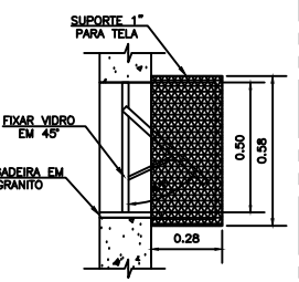
CORTE C-C ESC. 1:70
