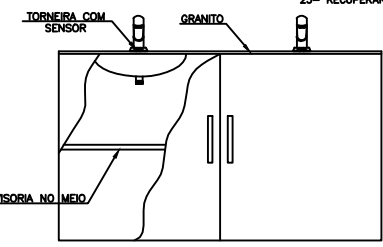
DETALHE TORNEIRA E CABINETE ESC. 1:70
