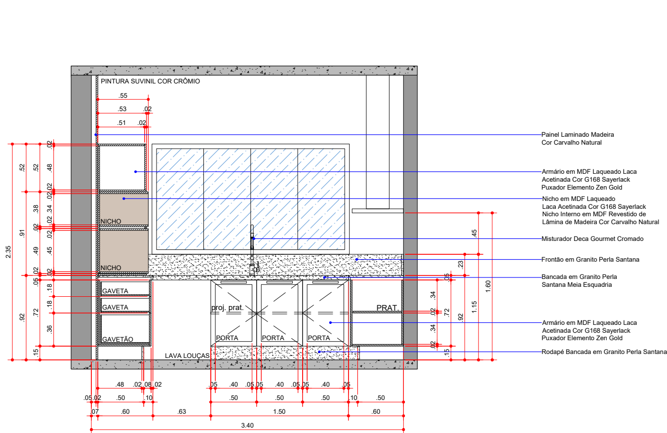
COZINHA - VISTA 01 esc. 1/25
