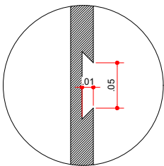
DET. PUXADOR MEIA CAVA - PLANTA sem escala
