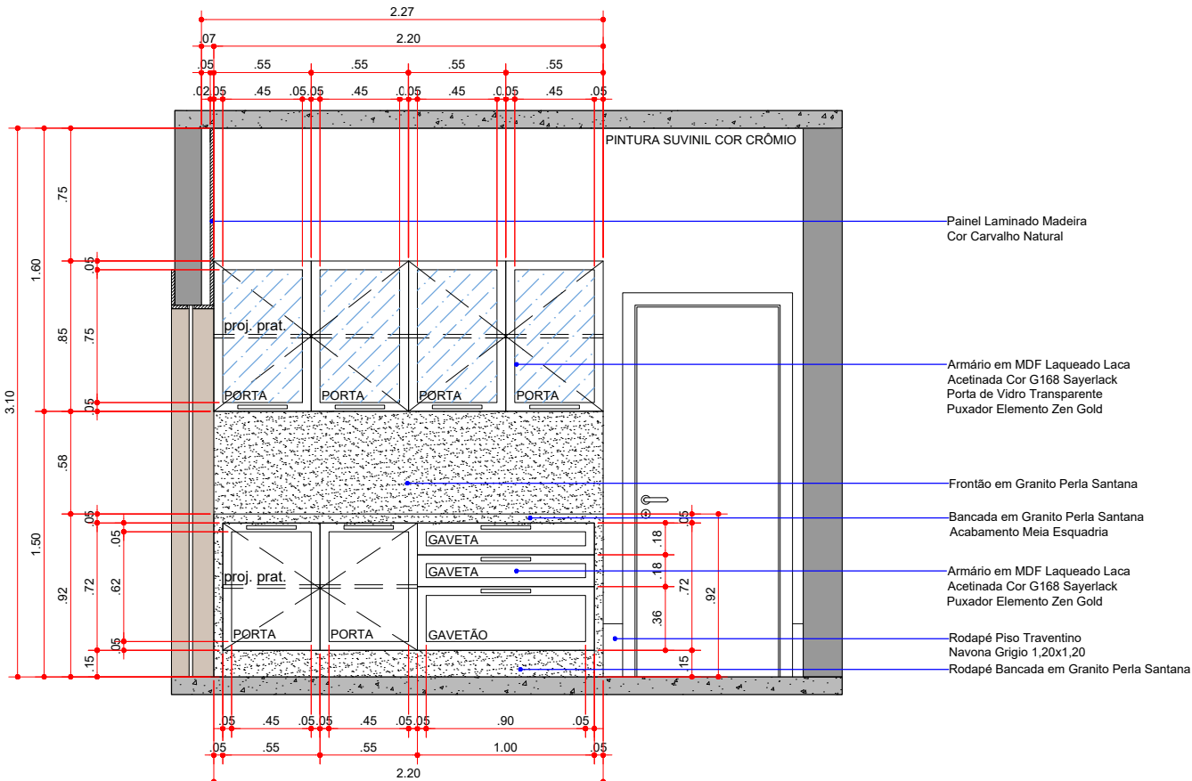
COZINHA - VISTA 03 esc. 1/25
