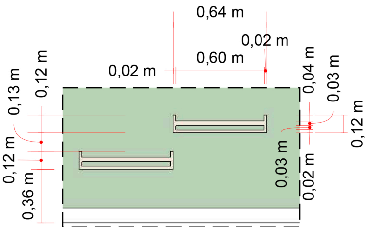
VISTA FRONTAL - PORTA LIVROS Esc: 1/25
