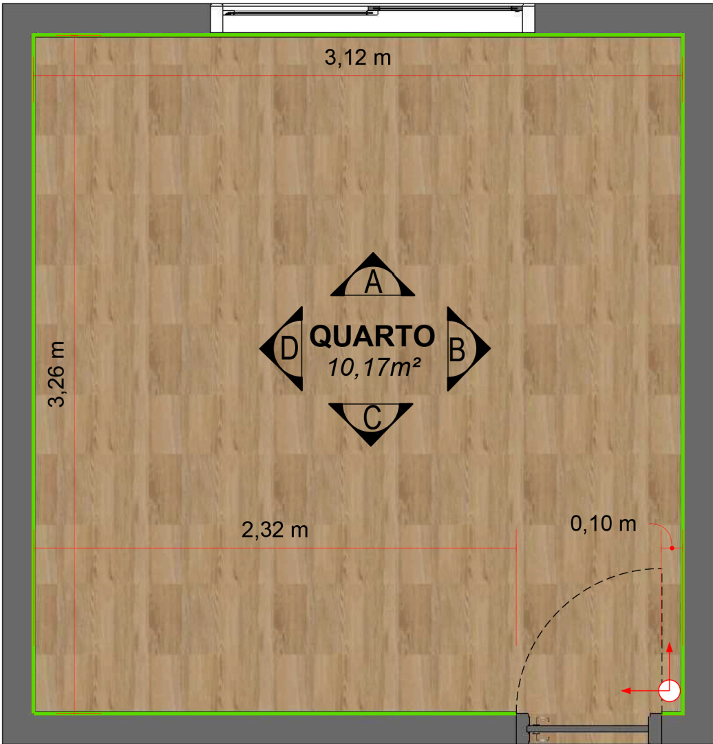
PLANTA DE PAGINAÇÃO DE PISO Esc: 1/25
