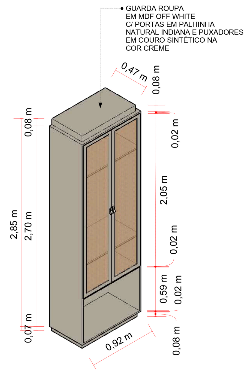
PERSPECTIVA - GUARDA ROUPA Esc: 1/25
