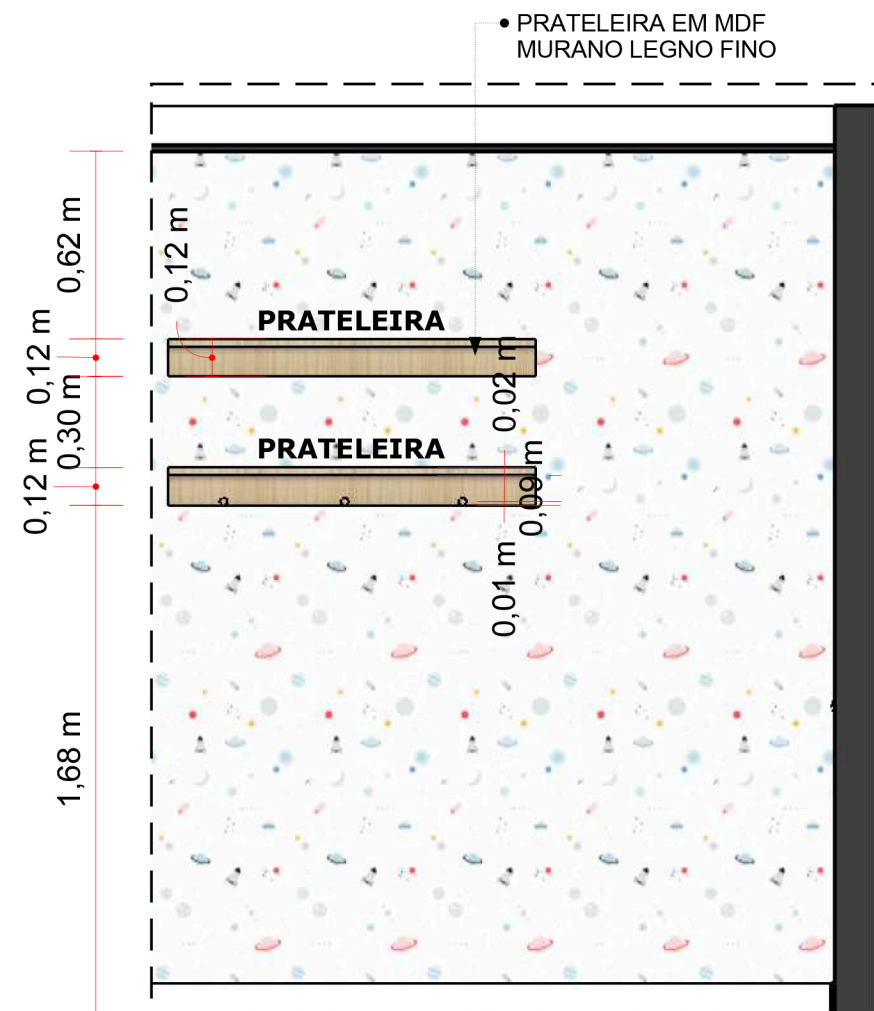
VISTA FRONTAL - PRATELEIRAS Esc: 1/25
