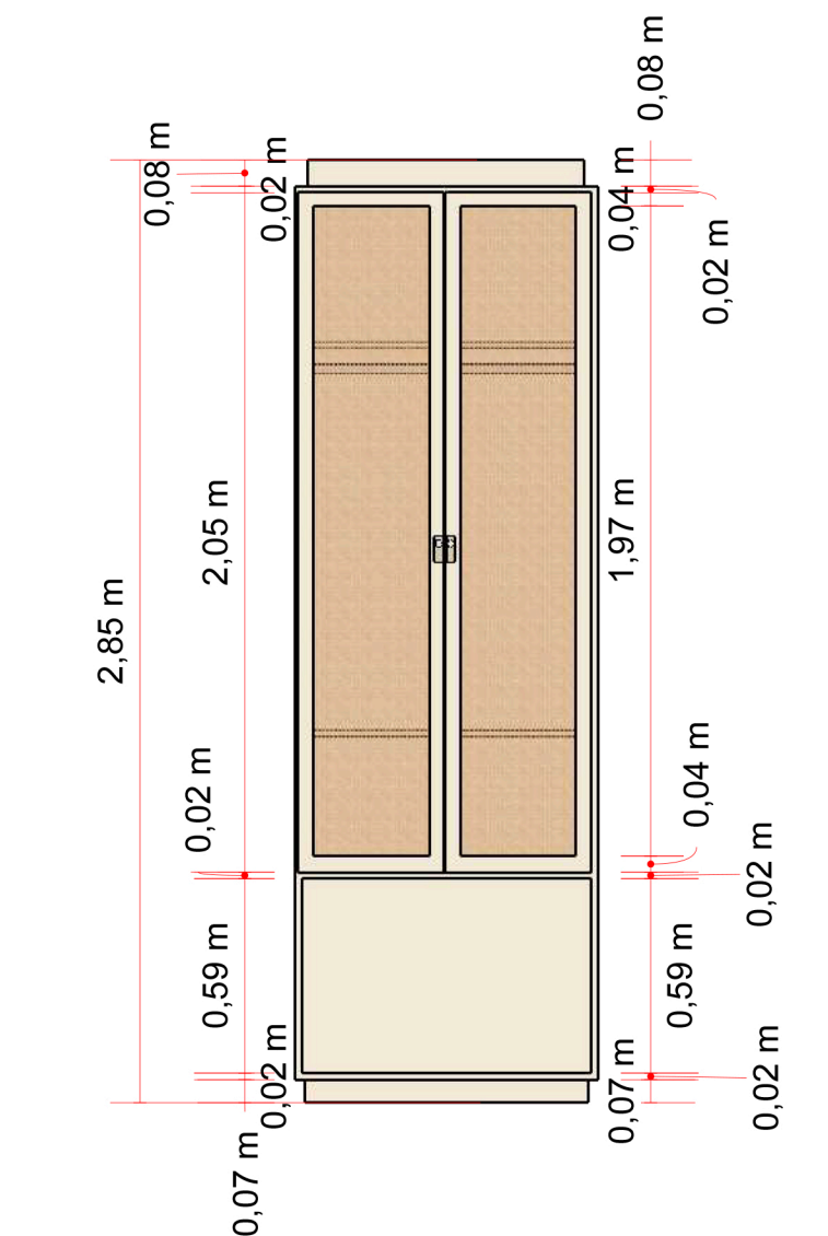
VISTA FRONTAL - GUARDA ROUPA C/ PORTA FECHADA Esc: 1/25
