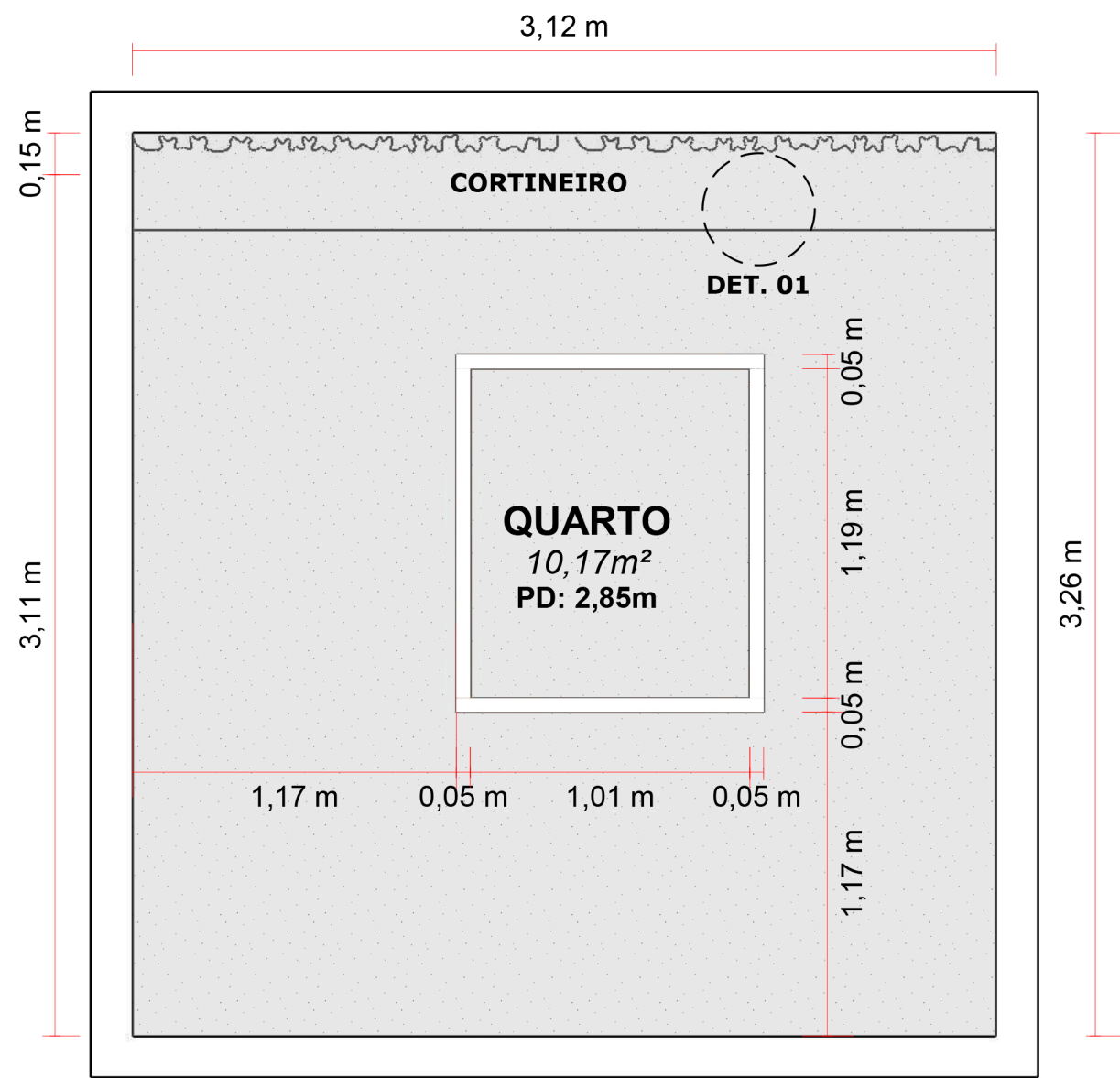
PLANTA DE FORRO Esc: 1/25
