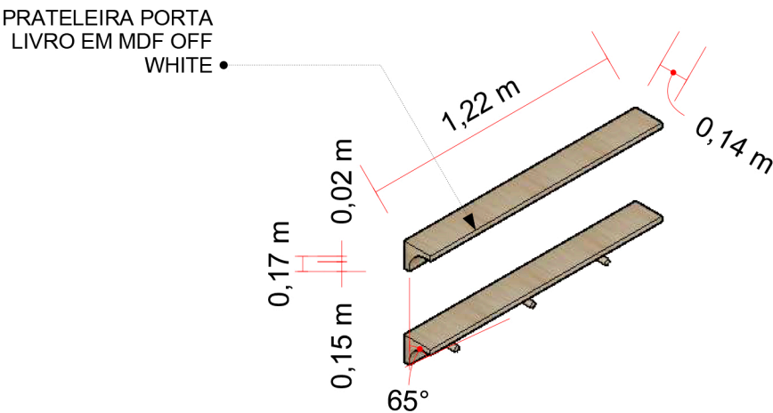
PERSPECTIVA - PRATELEIRAS Esc: 1/25
