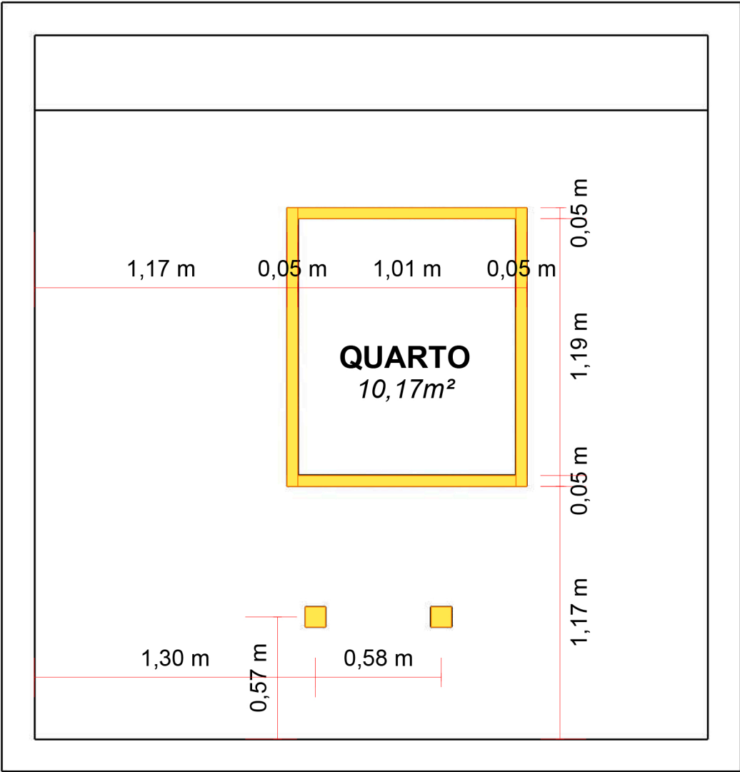
PLANTA DE ILUMINAÇÃO Esc: 1/25
