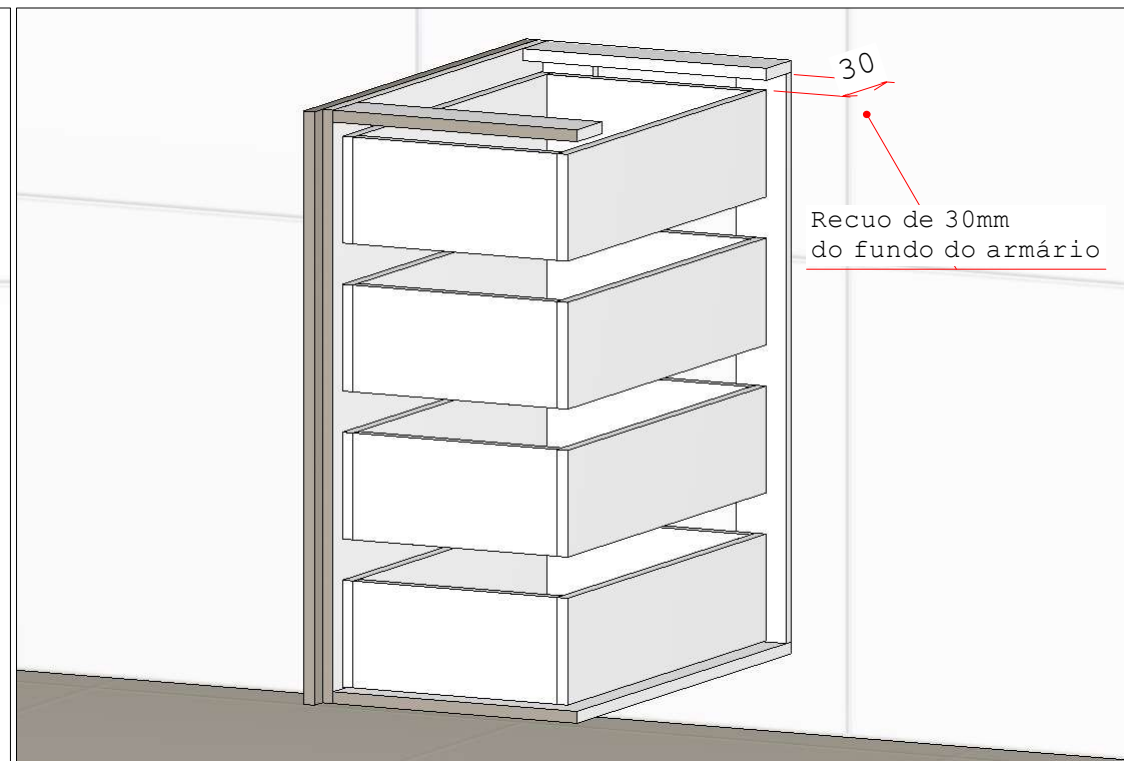
Detalhe A - Gaveteiro
