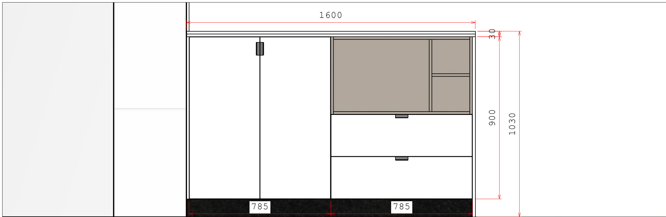
Detalhe B - Bancada
