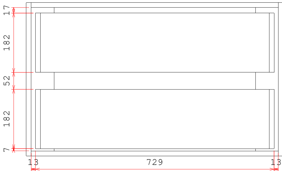
Detalhe B - Gaveta Bancada
