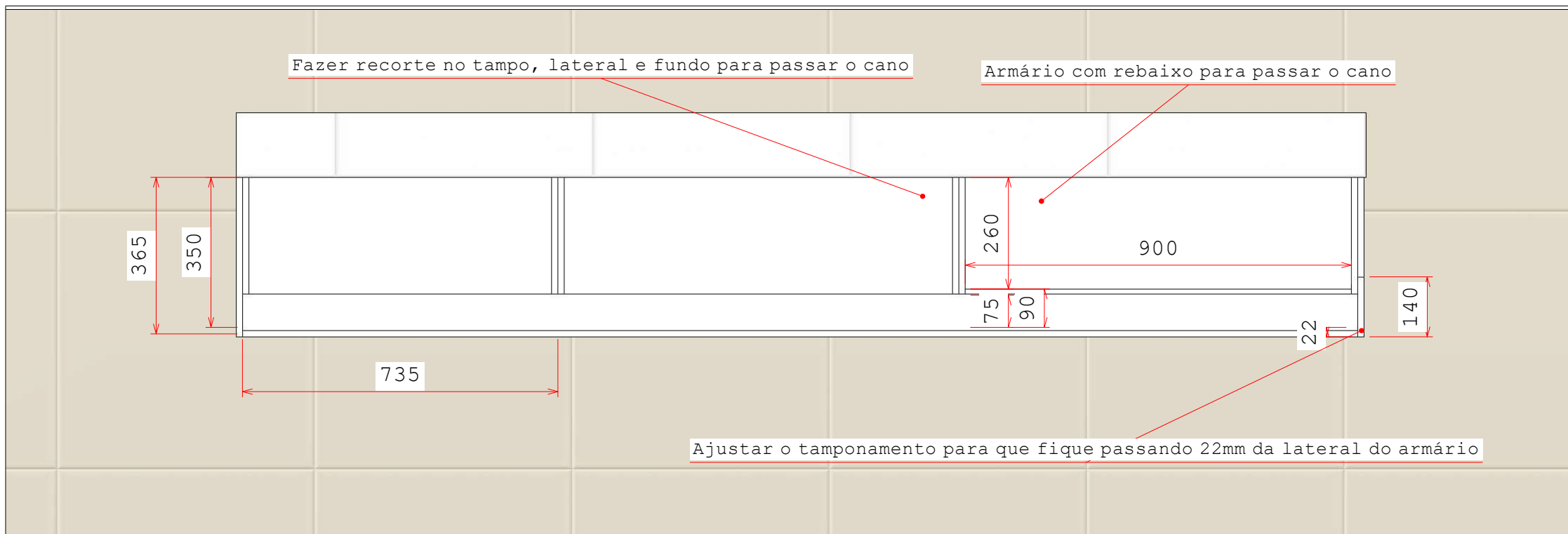
Detalhe A Superior s/ Cano
