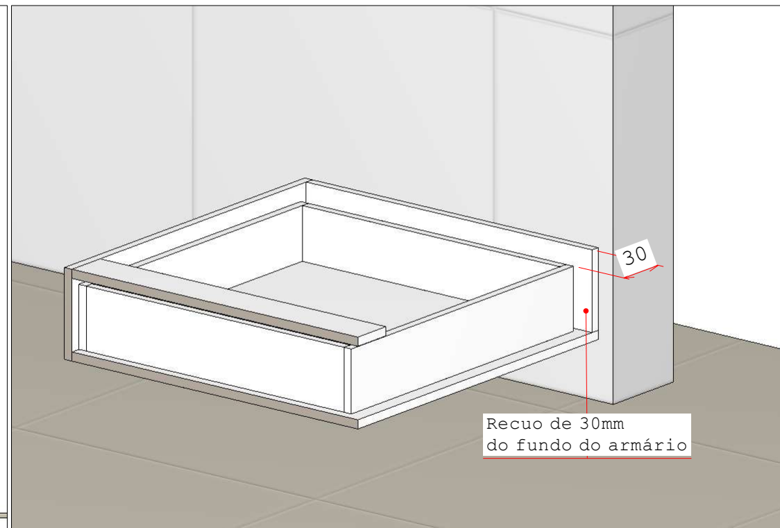
Detalhe A - Gaveta Forno
