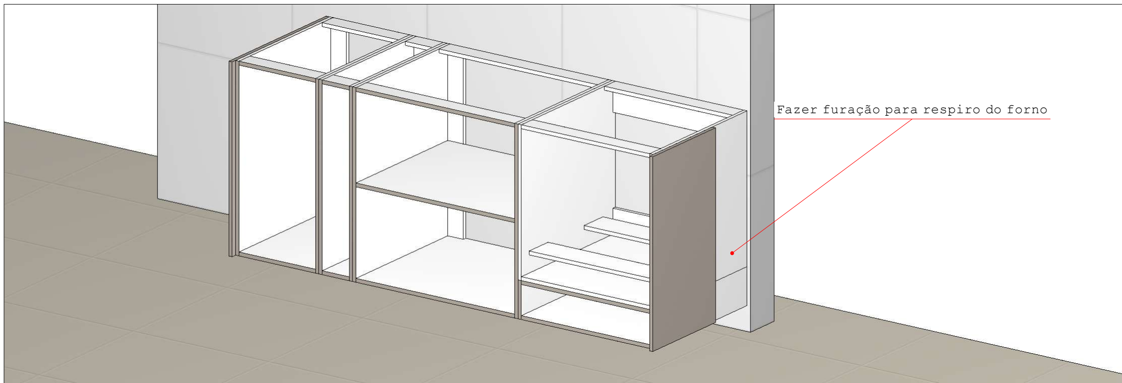
Detalhe A - Interno
