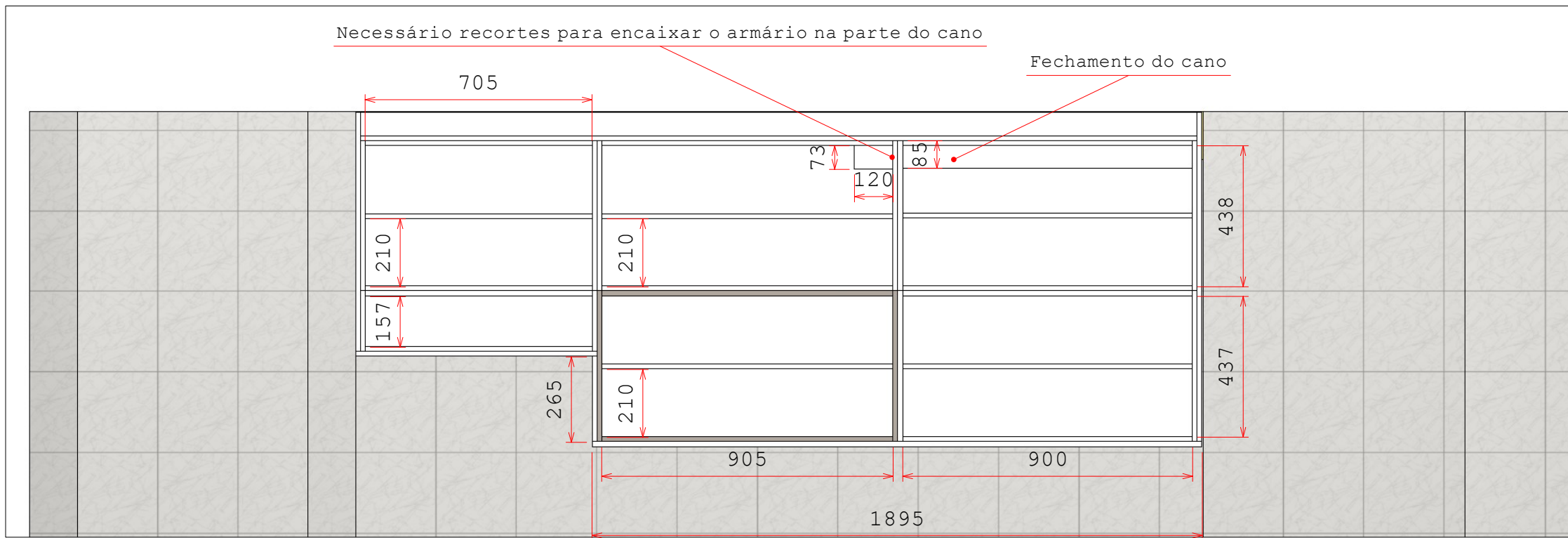
Detalhe A Superior Interno
