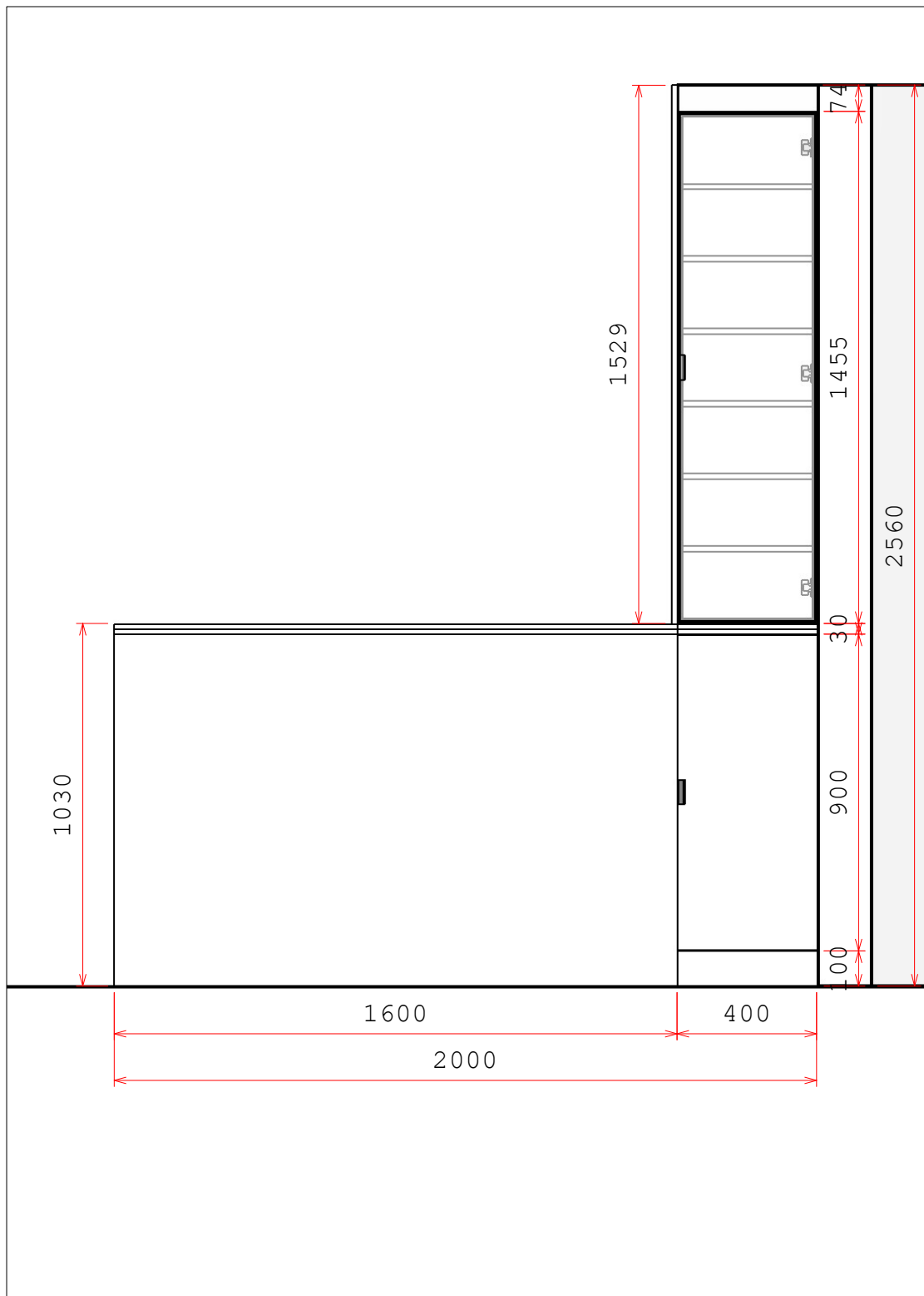
Detalhe C
