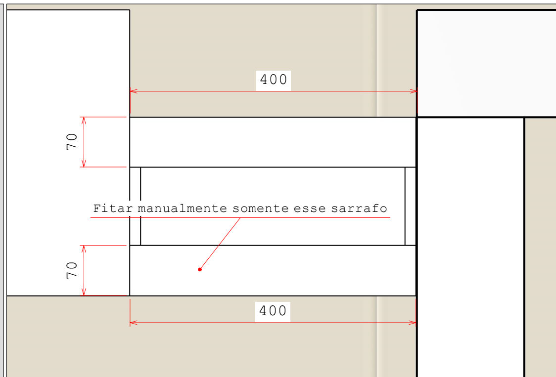
Detalhe C Sarrafo Bancada
