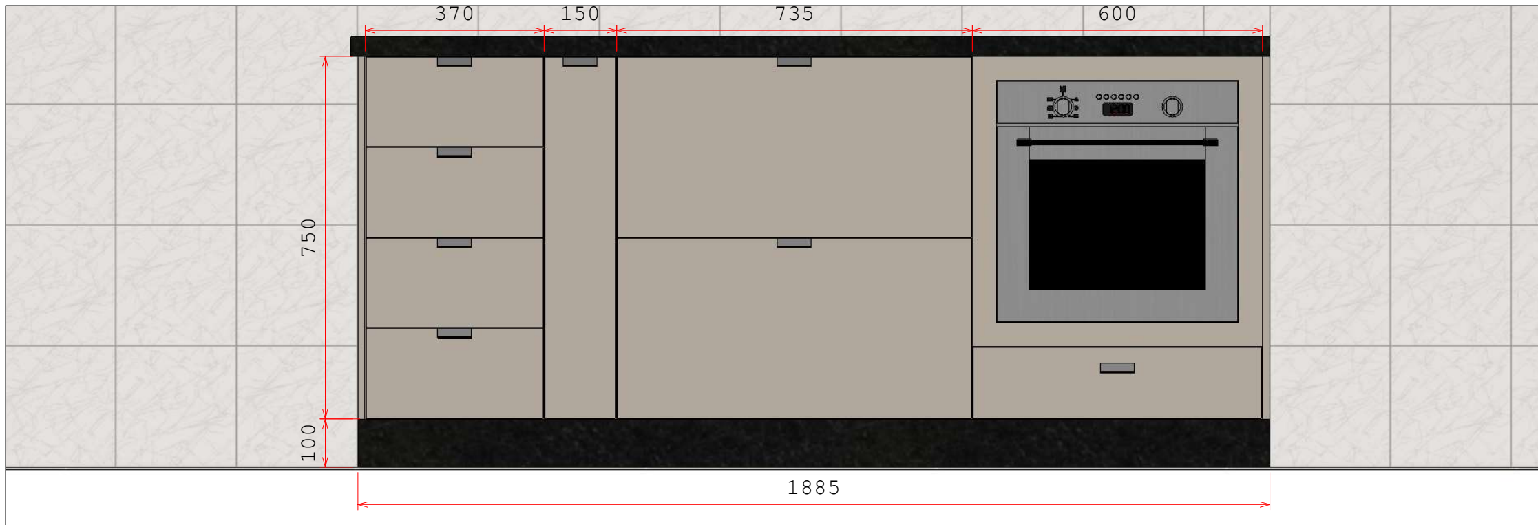
Detalhe A
