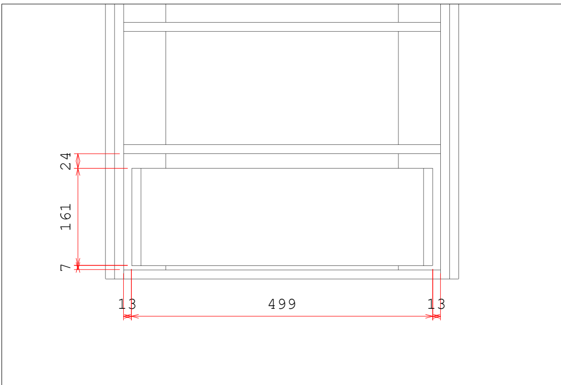
Armário Banheiro Interno Gaveta
