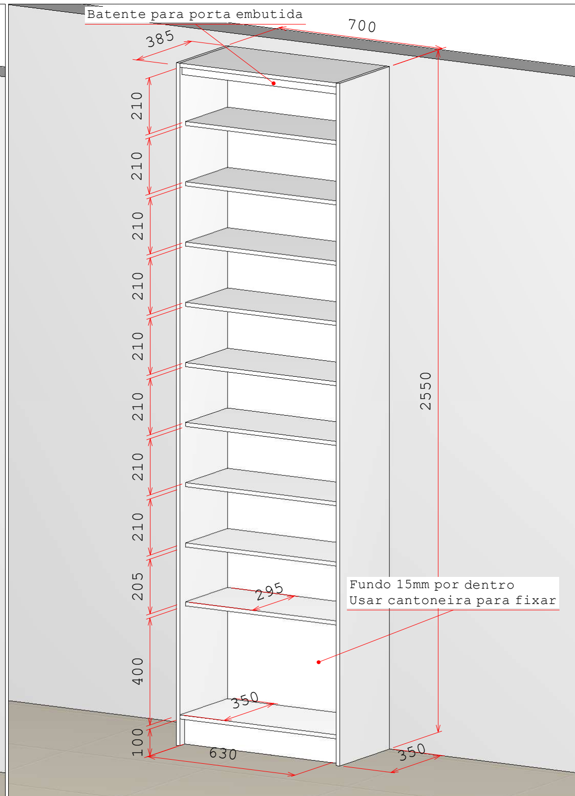
Sapateira Interno
