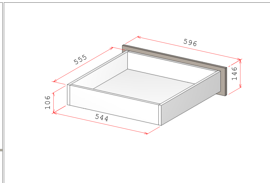
Detalhe Gaveta
