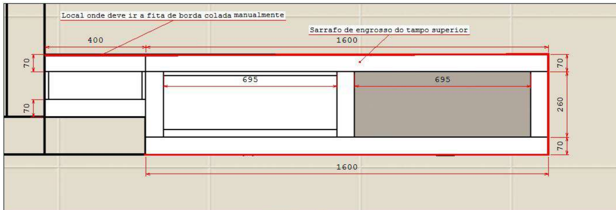
Detalhe Tampo da Bancada
