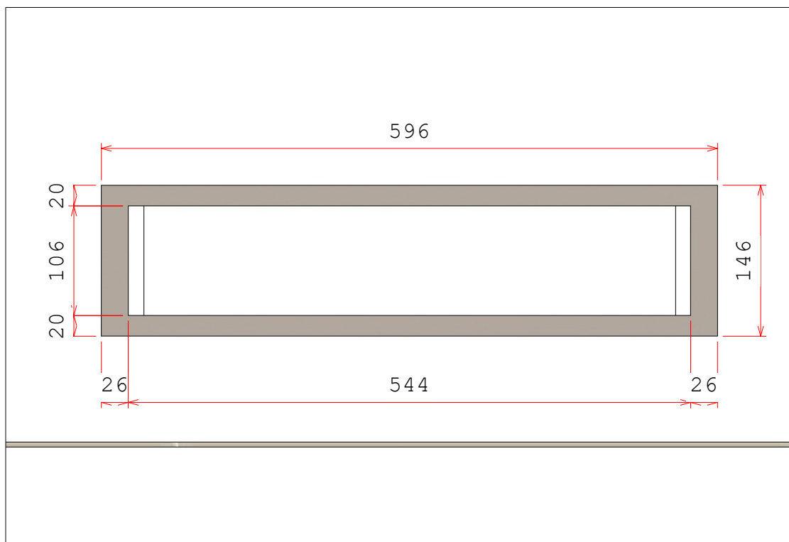
Detalhe Gaveta
