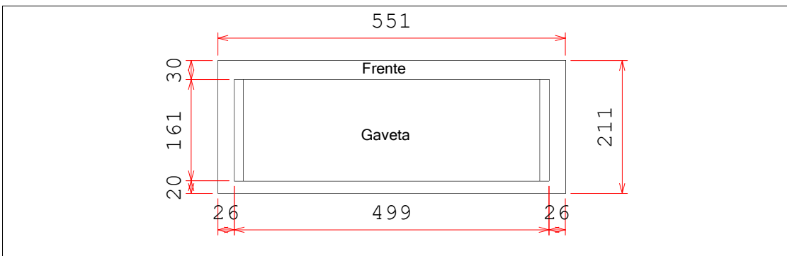
Detalhe Gaveta
