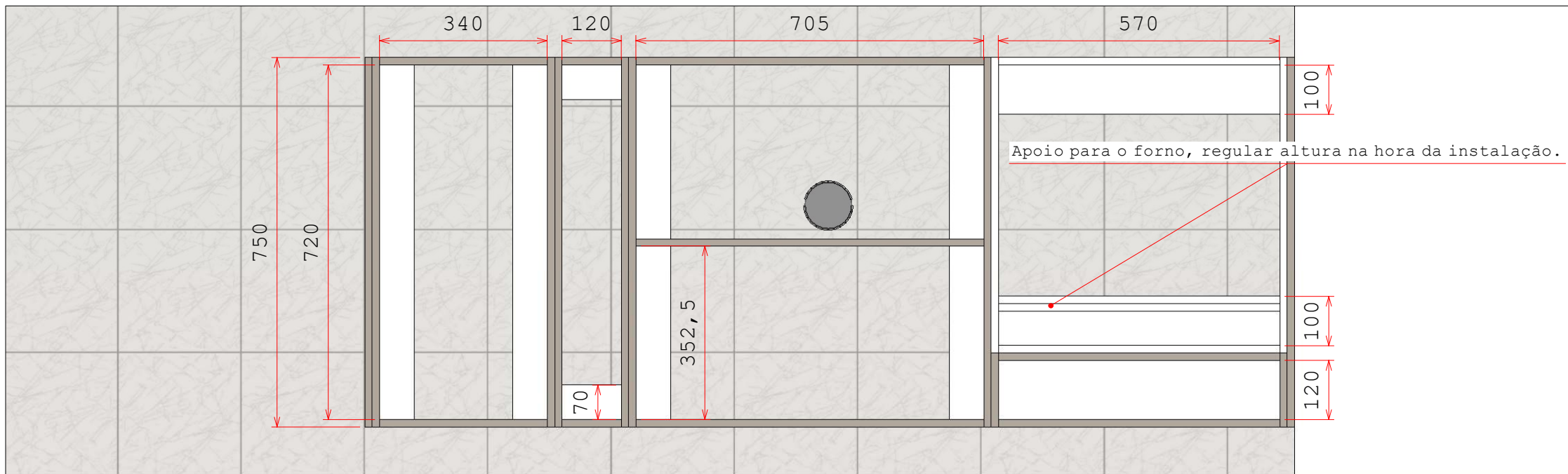
Detalhe A
