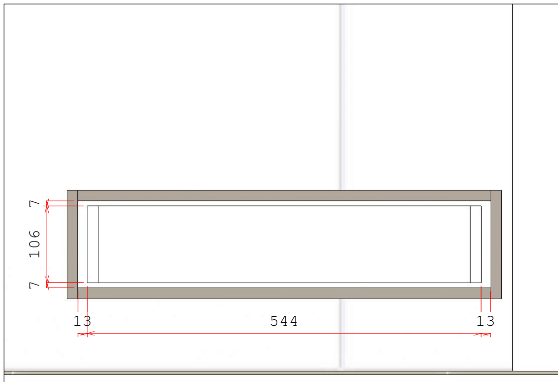
Detalhe A - Gaveta Forno
