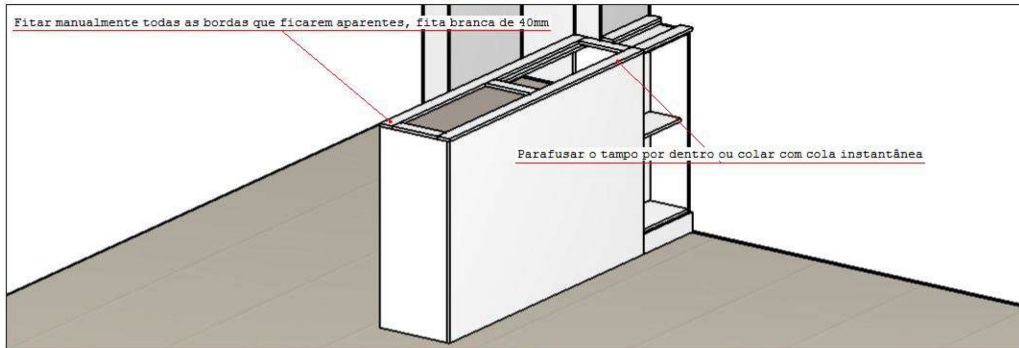
Detalhe Tampo Bancada
