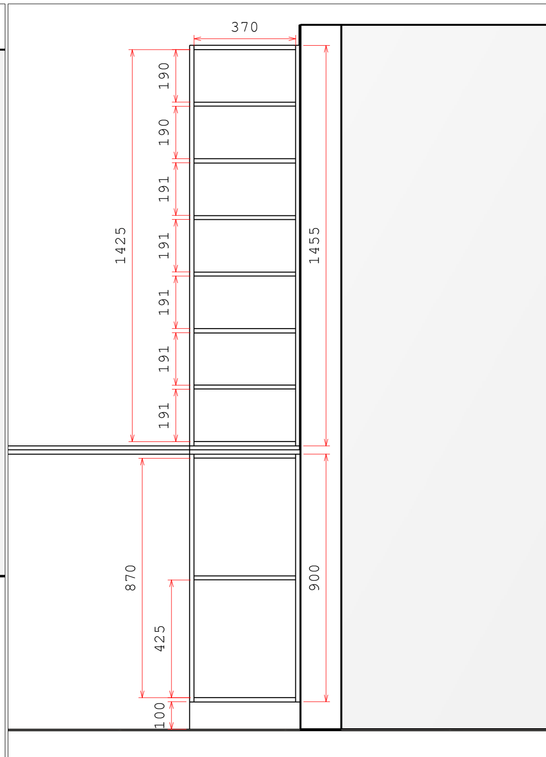
Detalhe C Interno
