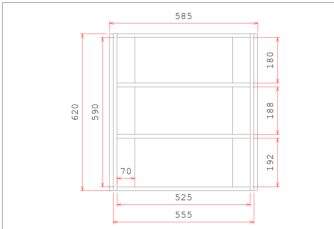
Armário Banheiro Interno
