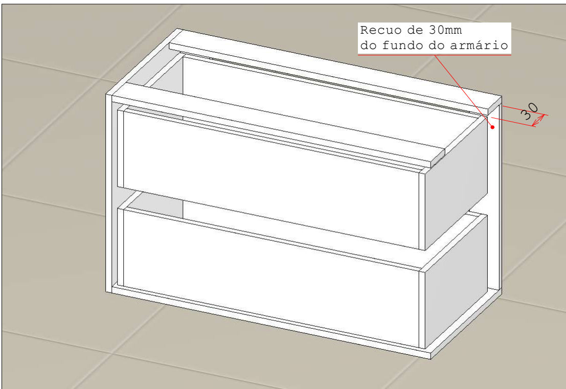
Detalhe B - Gaveta Bancada
