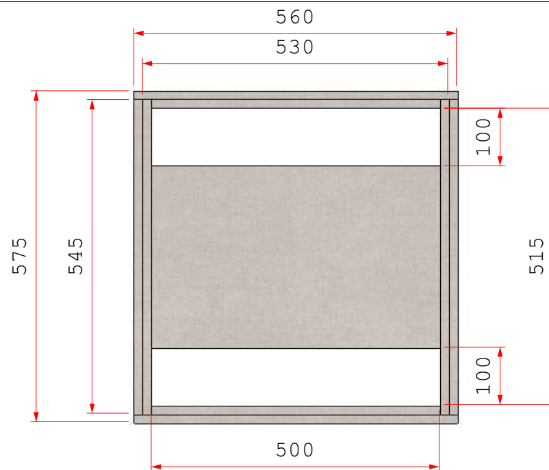
Vista B - Módulo 3
