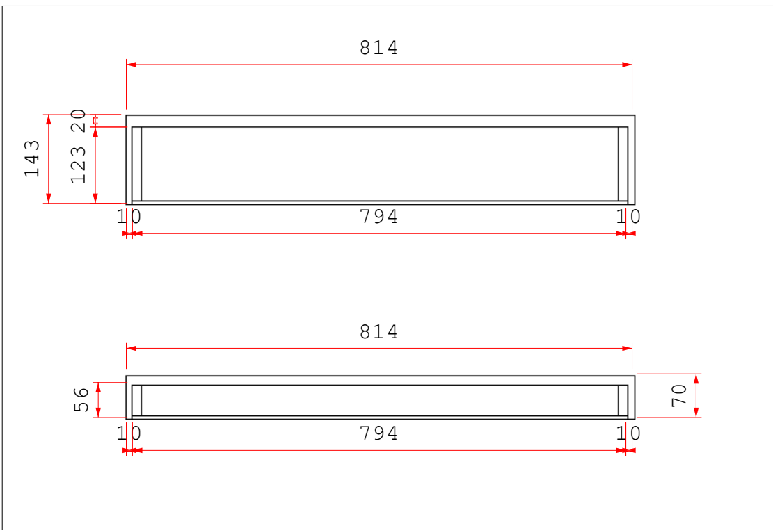
Vista A - Gaveta e Sapateira
