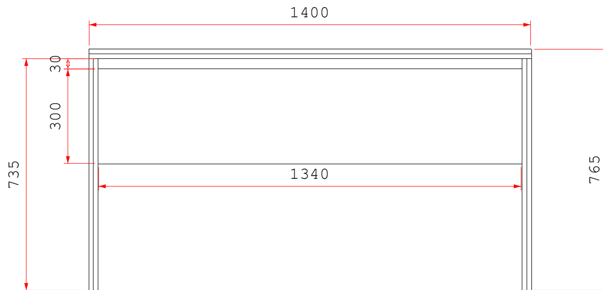
Vista B - Mesa Estudo
