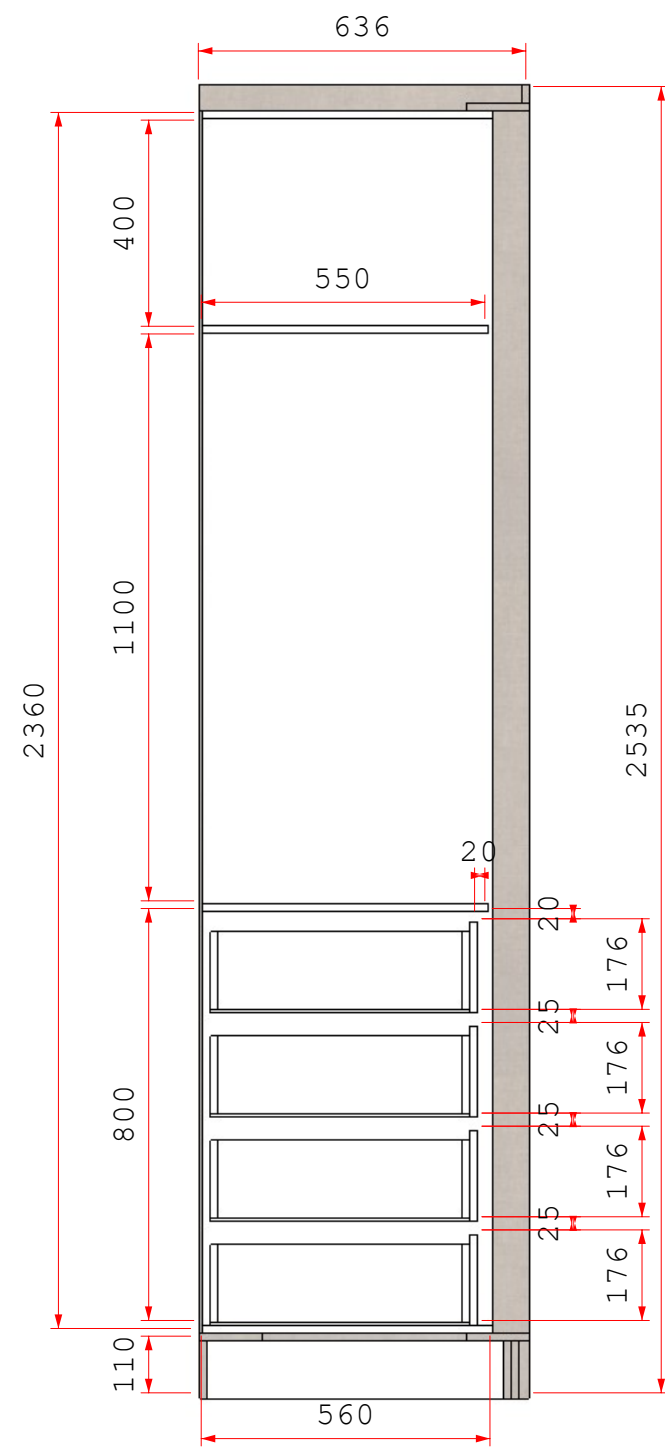
Vista A - Roupeiro Lado Dir.
