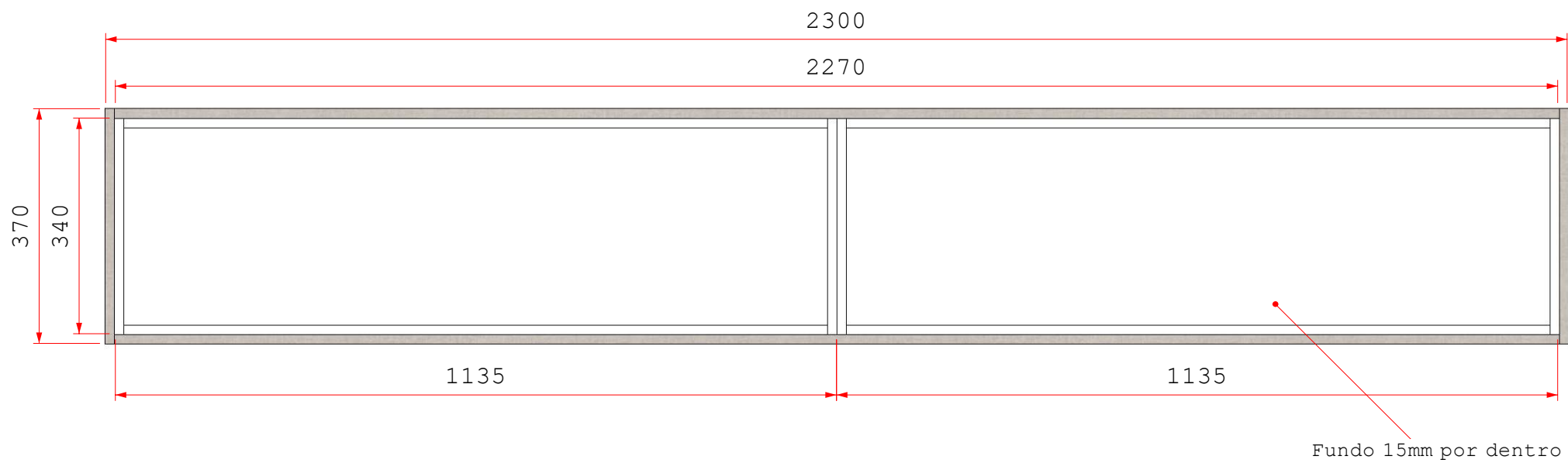
Vista B - Mód. Aéreo
