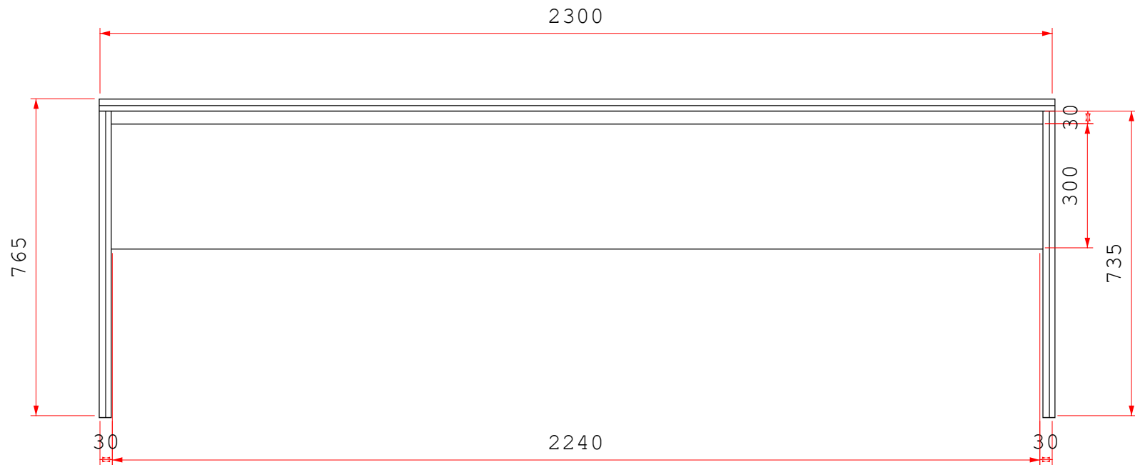
Vista B - Mesa Estudo
