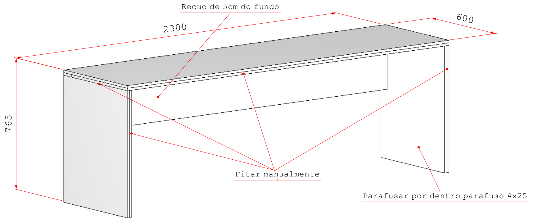
Vista B - Mesa Estudo
