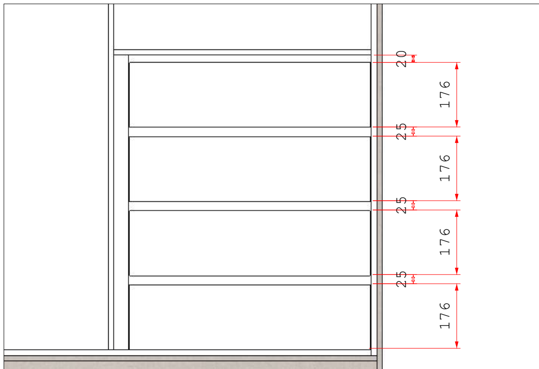
Vista A - Gaveta Roupeiro
