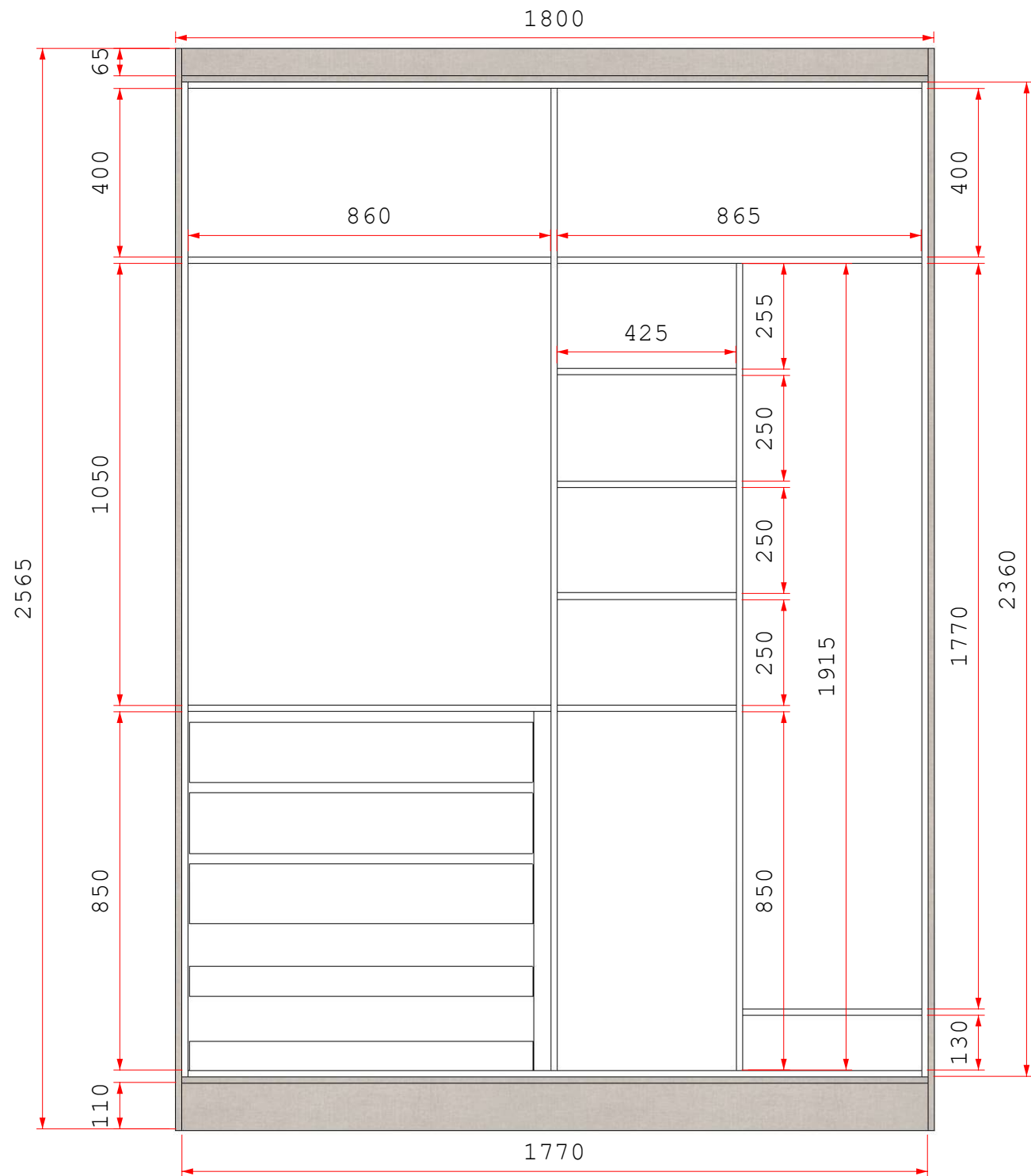
Vista A - Roupeiro
