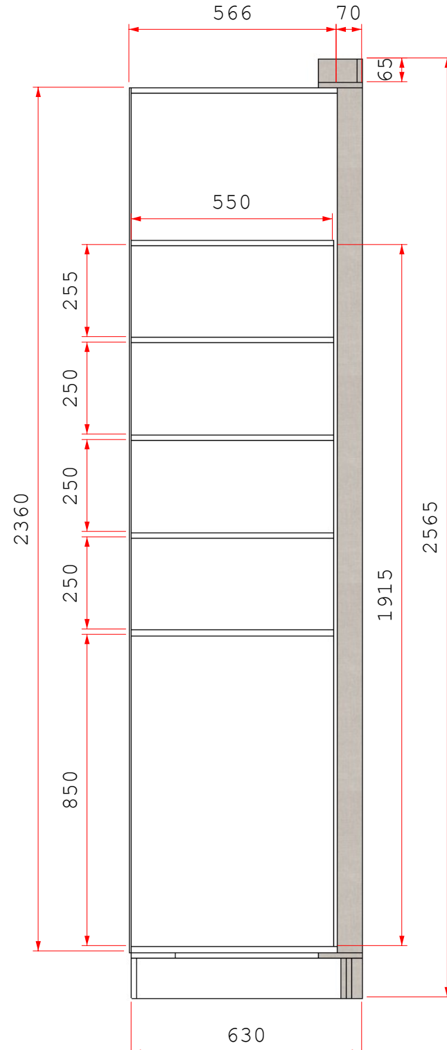
Vista A - Roupeiro Lado Dir.
