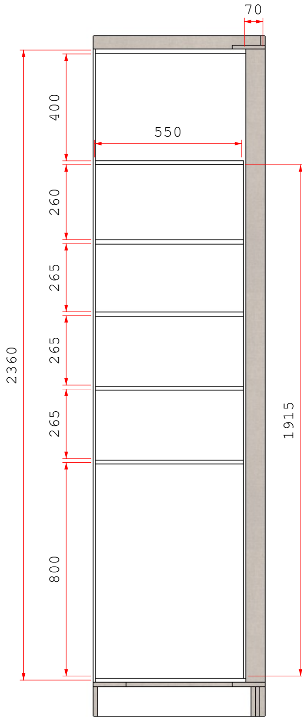
Vista A - Roupeiro Centro
