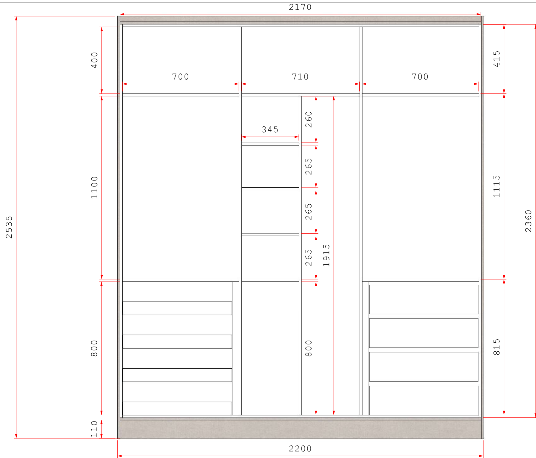
Vista A - Roupeiro Interno
