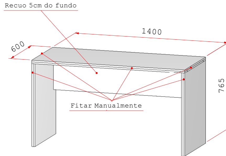
Vista B - Mesa Estudo
