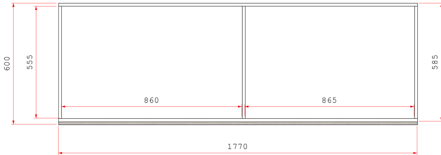
Vista A - Base Roupeiro
