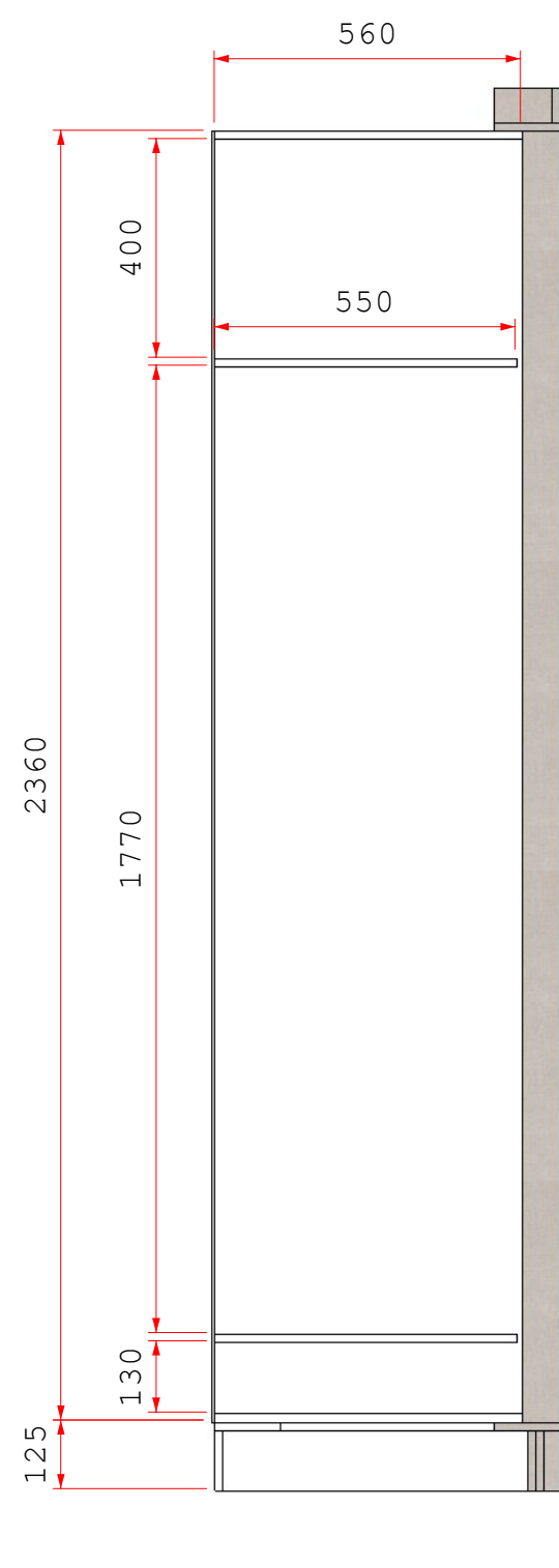
Vista A - Roupeiro Lado Dir.
