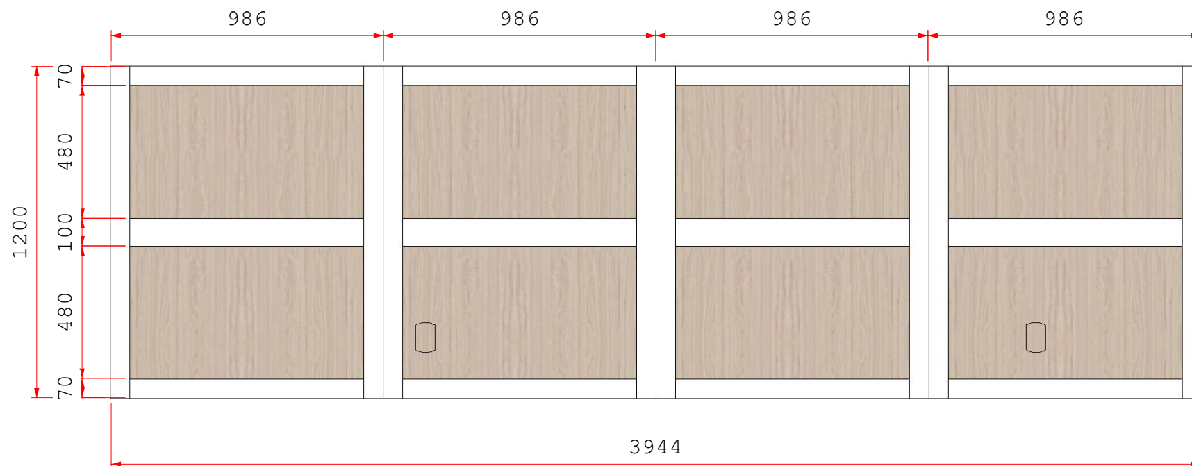
Vista A - Painel Cabeceira
