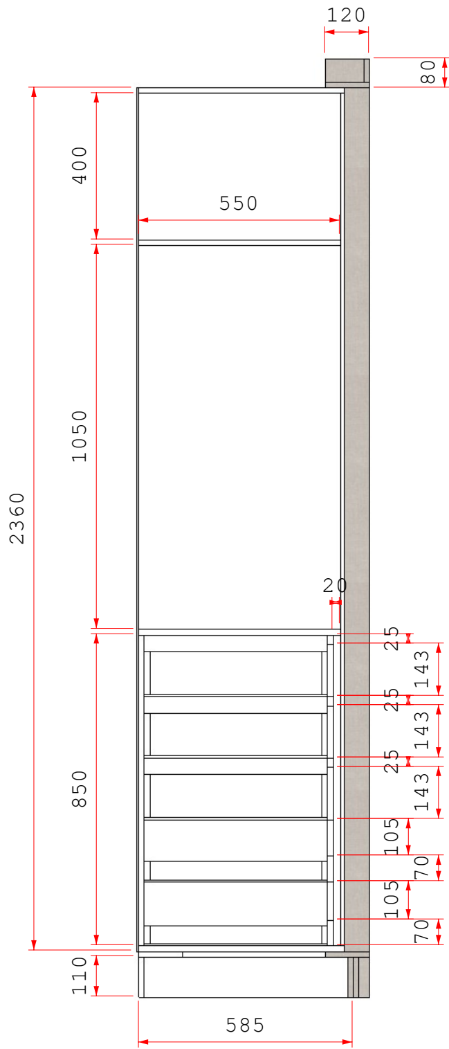
Vista A - Roupeiro Lado Esq.
