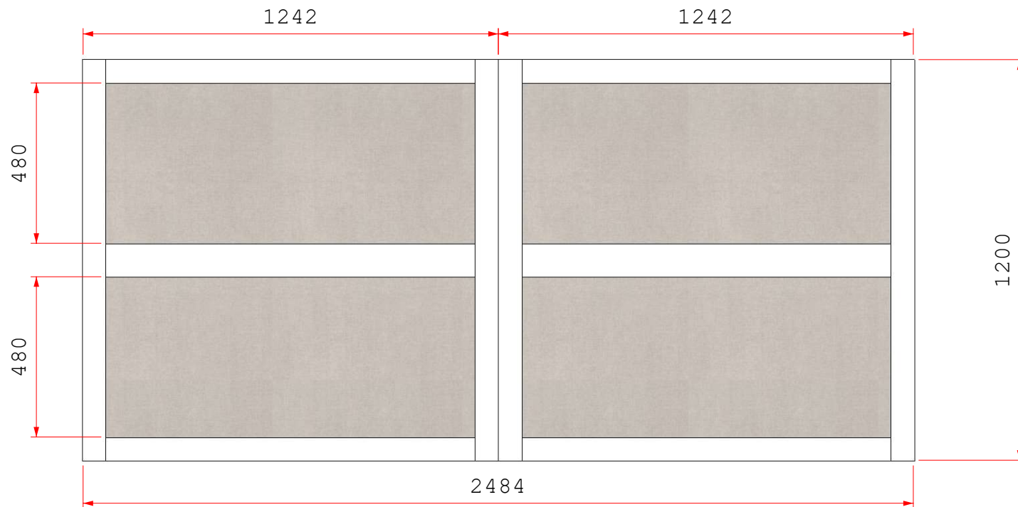
Vista C - Painel Cabeceira
