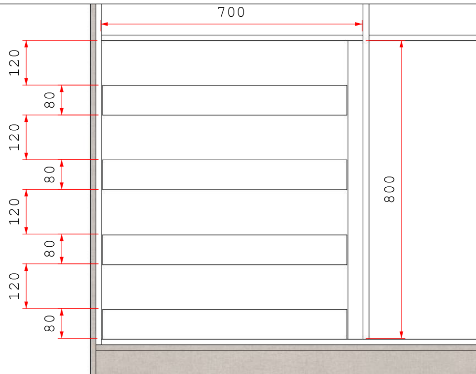
Vista A - Sapateira Roupeiro
