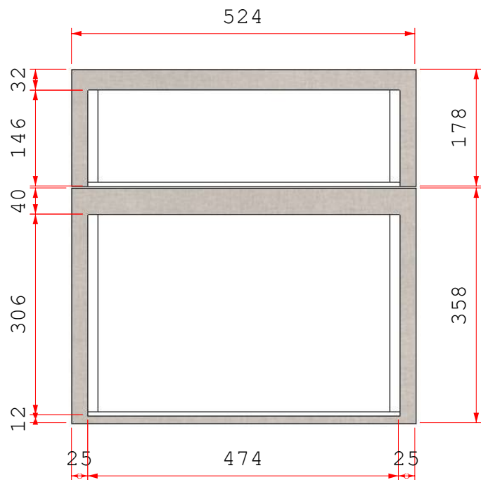
Vista B - Módulo 4
