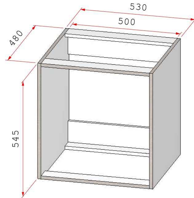
Vista B - Módulo 4
