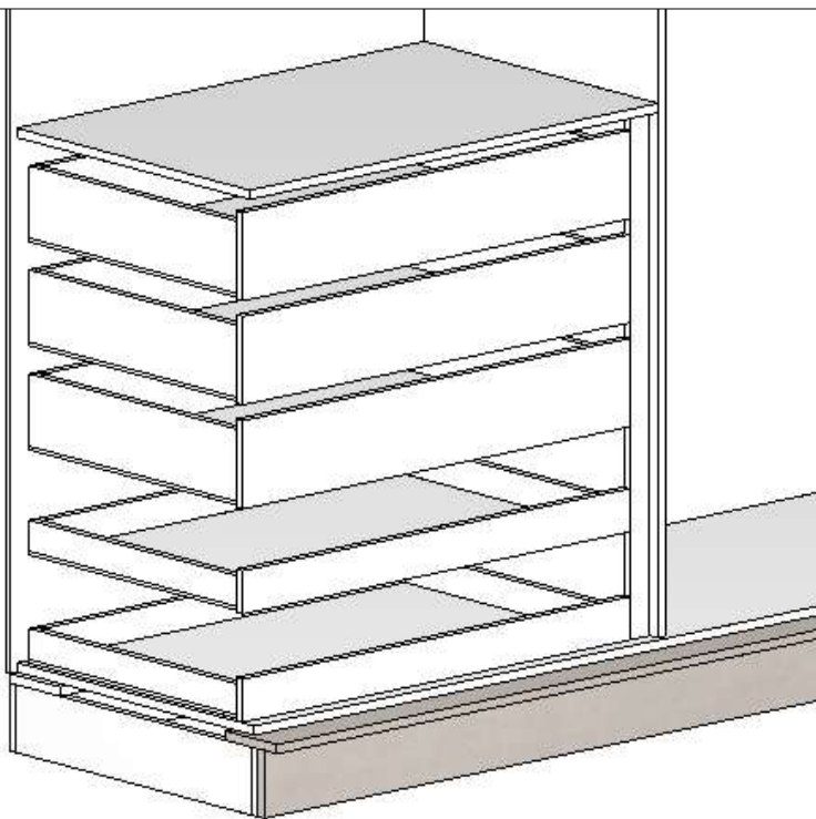
Vista A - Gaveta e Sapateira
