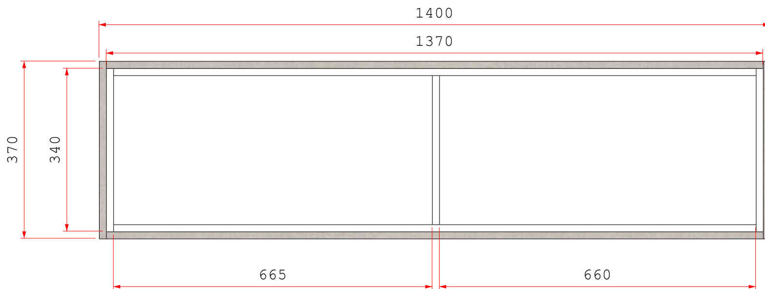
Vista B - Arm. Aéreo
