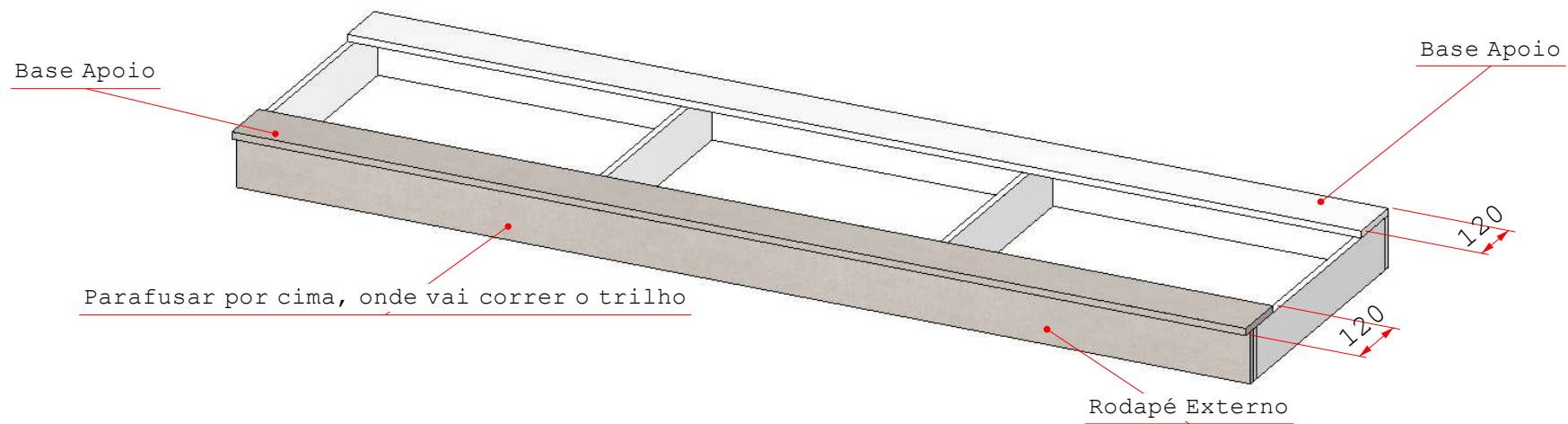
Vista A - Base Roupeiro
