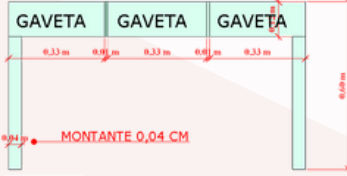
FRENTE
