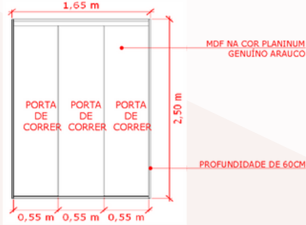
VISTA FRONTAL PORTAS
