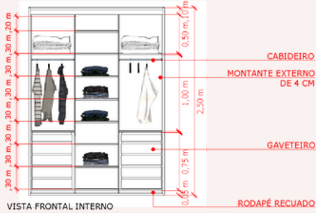
VISTA FRONTAL INTERNO
