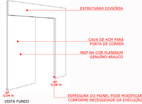
VISTA FUNDO
