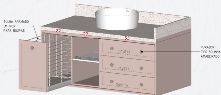
0101 MÓVEL - INTERNO PERSPECTIVA
