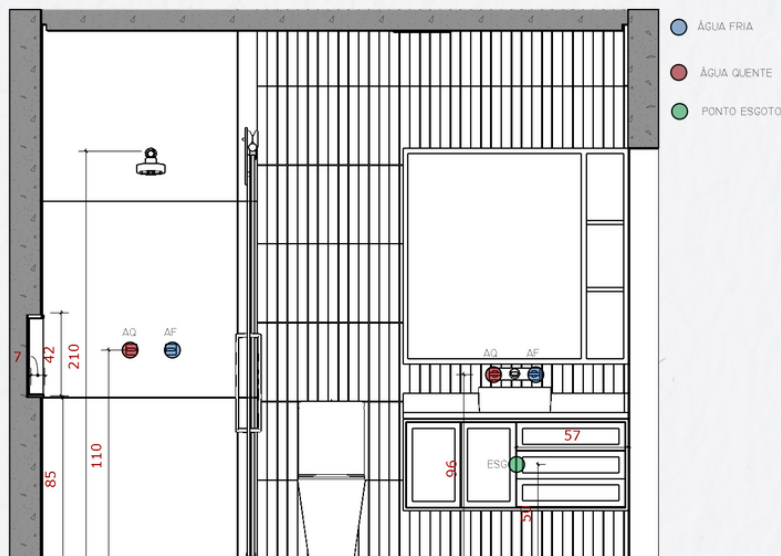
2 CORTE TÉCNICO ESCALA 1/20
