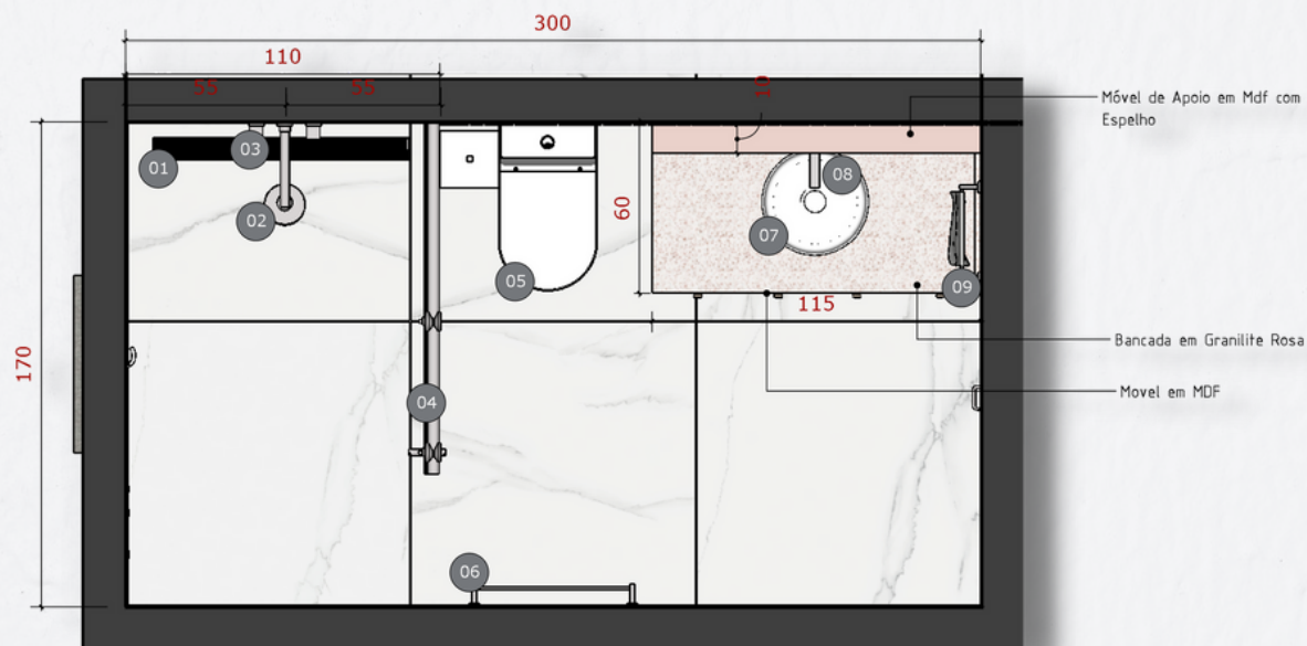
1 LAYOUT - Banheiro Olivia ESCALA 1/20
