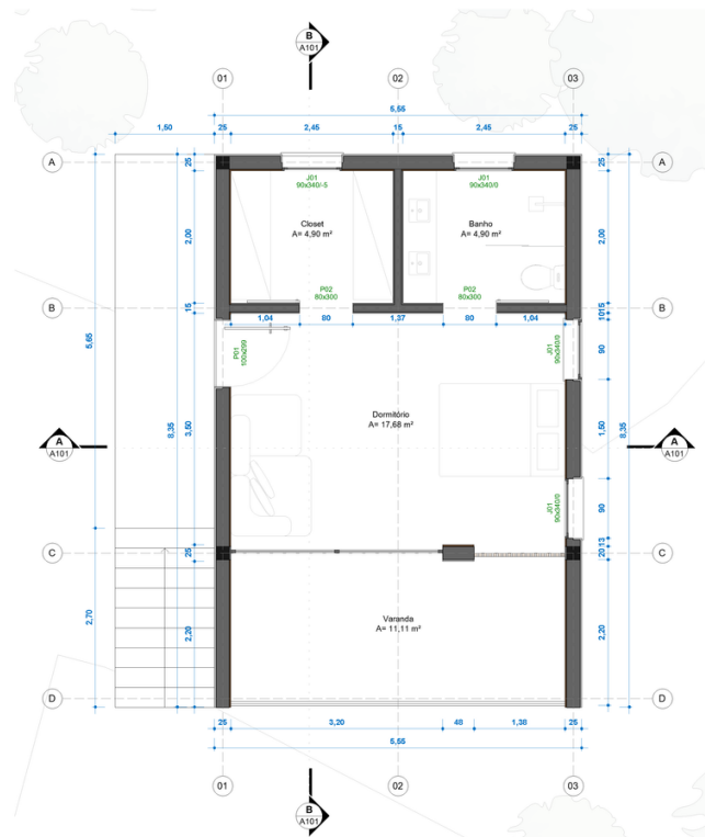
PLANTA BAIXA TÉRREO ESC: 1 : 50
