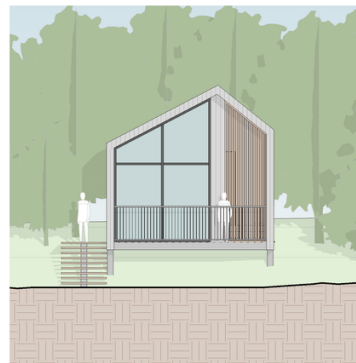
FACHADA SUL ESC: 1 : 100
