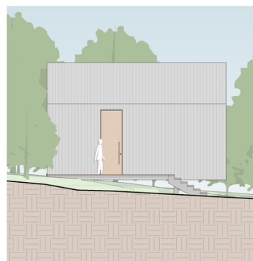
FACHADA OESTE ESC: 1 : 100
