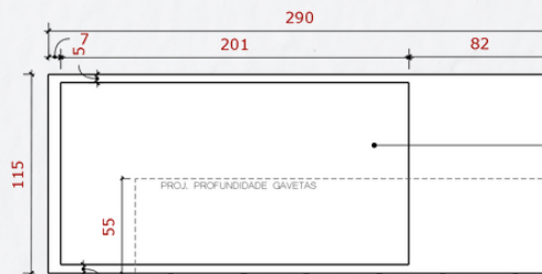
003 DET 03 - BASE CAMA VISTA PLANTA ESCALA 1/25
