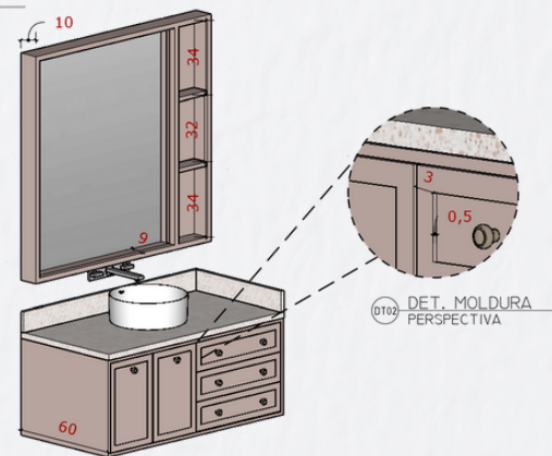
2 VISTA GERAL - BANHEIRO ESCALA 1/20
