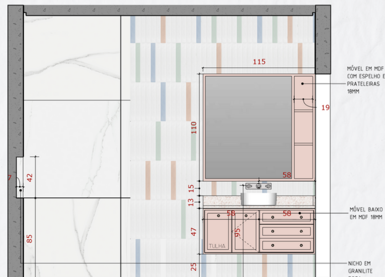
2 VISTA GERAL - BANHEIRO ESCALA 1/20
