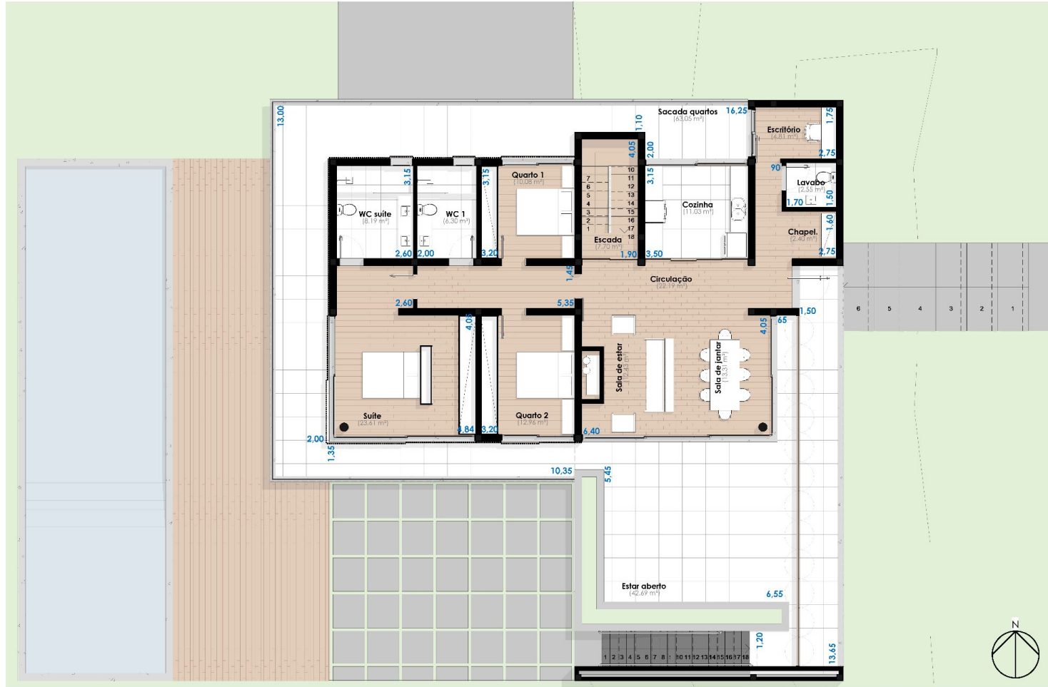
Planta Térreo
