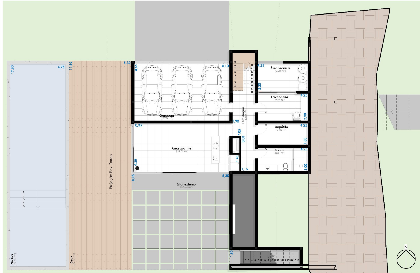
Planta Subsola
