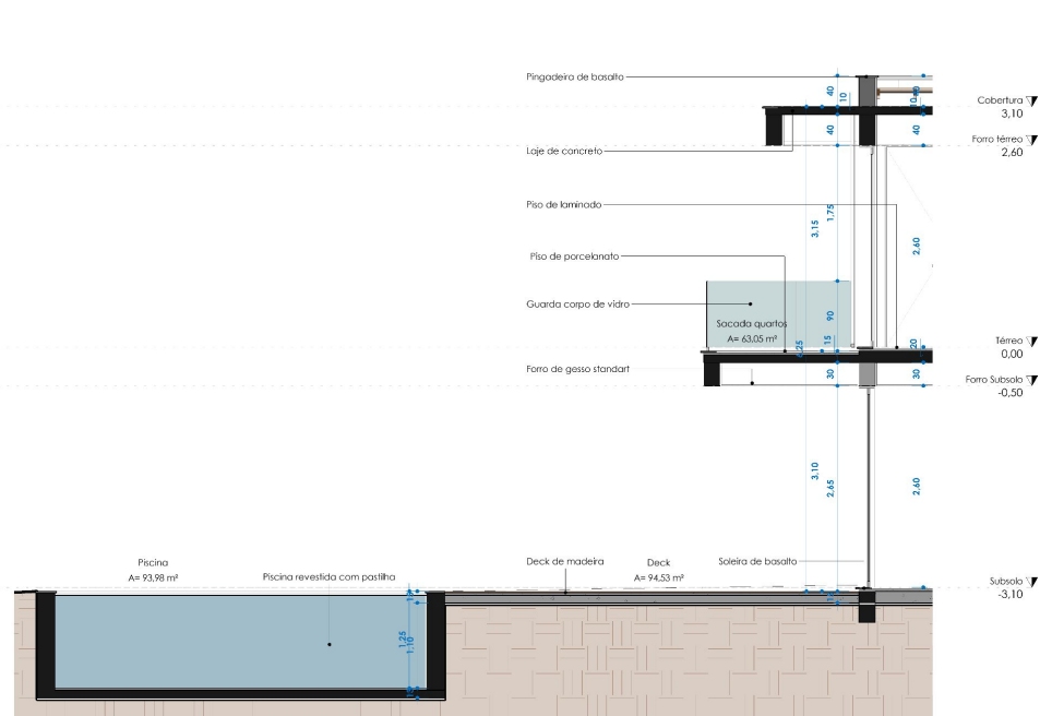
Detalhamento com corte perspectivado
