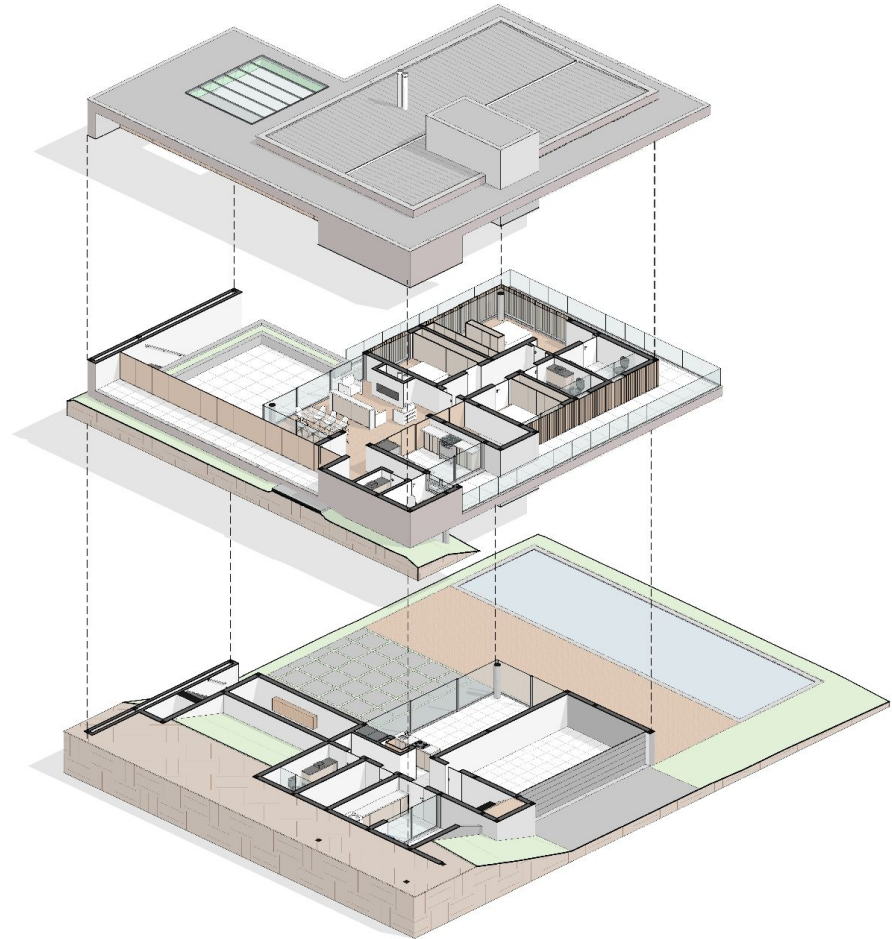
Cortes Isométricos
