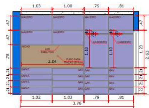
ELEVÇÃO 03 - INT. ESCALA 1: 50
