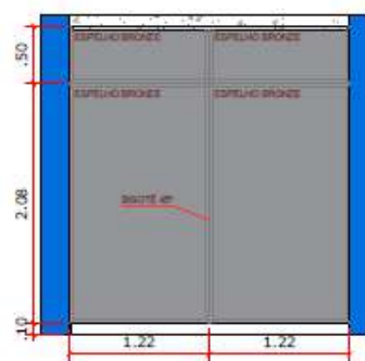
ELEVAÇÃO 03 ESCALA 1: 50
