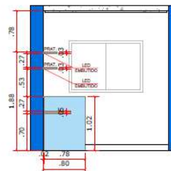
ELEVÇÃO 03 ESCALA 1: 50
