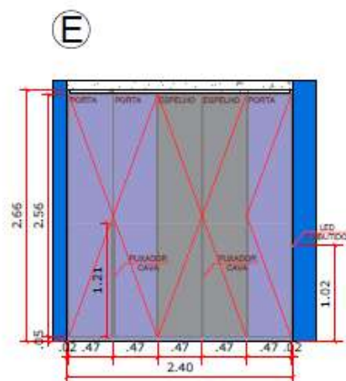
ELEVÇÃO 01 ESCALA 1: 50
