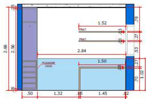
ELEVÇÃO 02 ESCALA 1: 50
