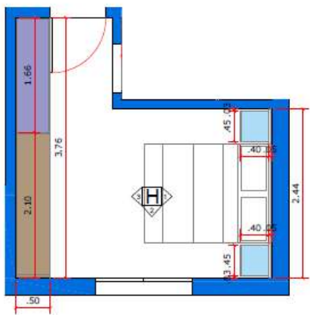
PLANTA ESCALA 1: 50
