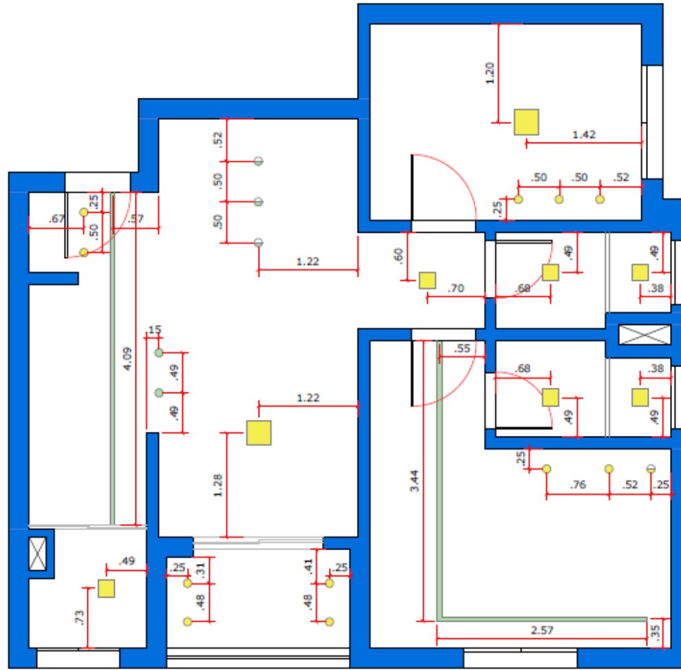
PLANTA ESCALA 1: 50
