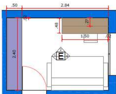
PLANTA ESCALA 1: 50
