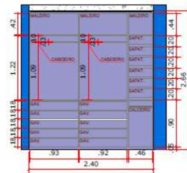
ELEVÇÃO 01 - INT. ESCALA 1: 50
