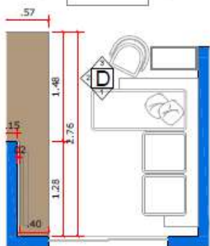
PLANTA ESCALA 1: 50
