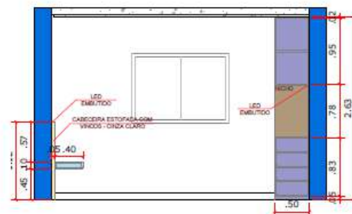
ELEVÇÃO 02 ESCALA 1: 50
