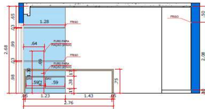
ELEVAÇÃO 02 ESCALA 1: 50
