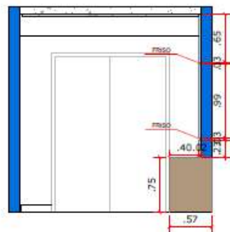
ELEVAÇÃO 01 ESCALA 1: 50
