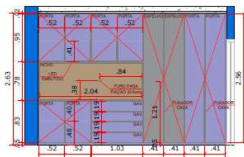
ELEVÇÃO 03 ESCALA 1: 50
