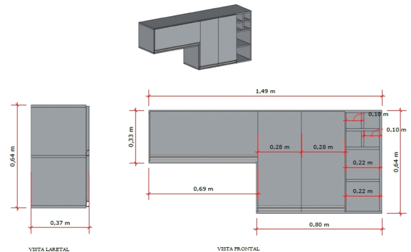
LayOut / Detalhamneto
