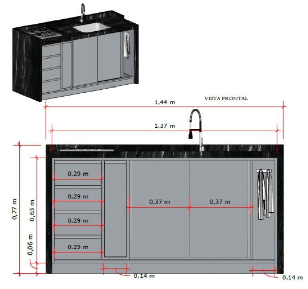
LayOut / Detalhamneto
