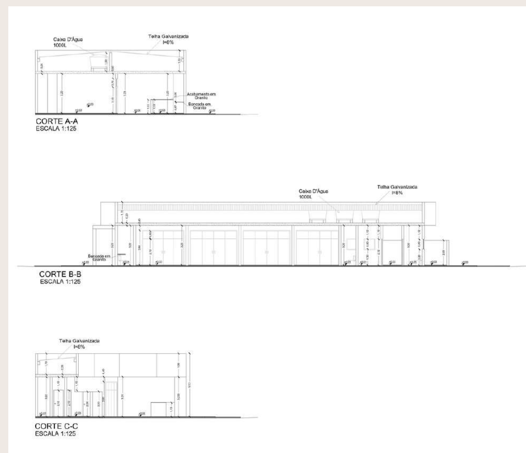
Cortes
