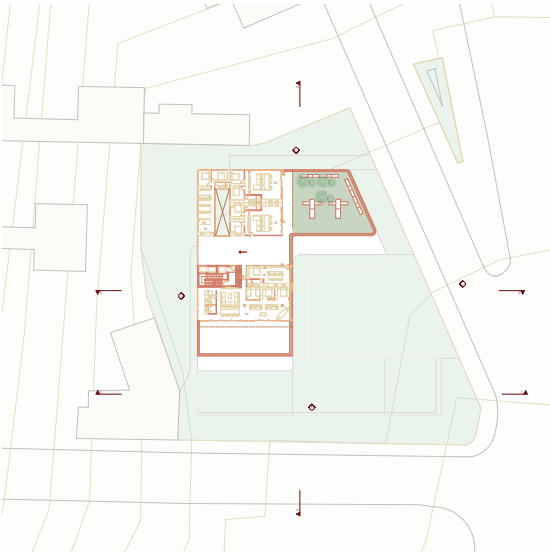
Planta - terceiro pavimento - sem escala
