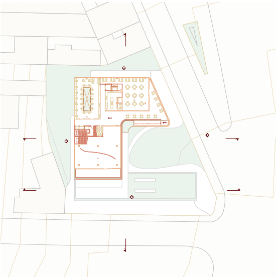
Planta - segundo pavimento - sem escala
