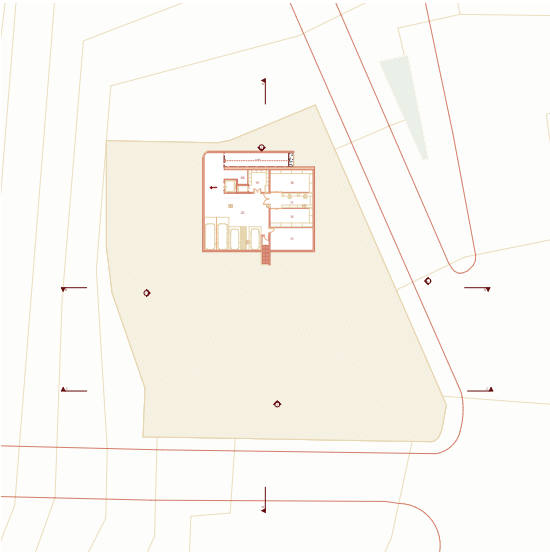
Planta - subsolo para carga e descarga - sem escala
