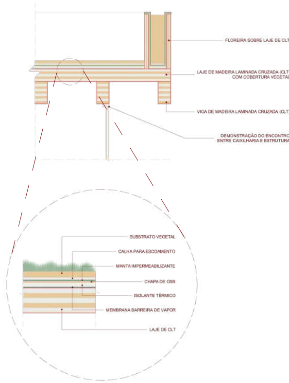
Diagrama - detalhe construtivo da estrutura de madeira com jardim - sem escala
