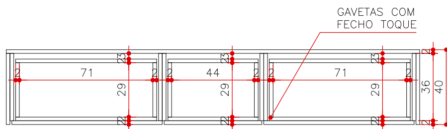
CORTE EE MA 07 ESCALA 1:20
