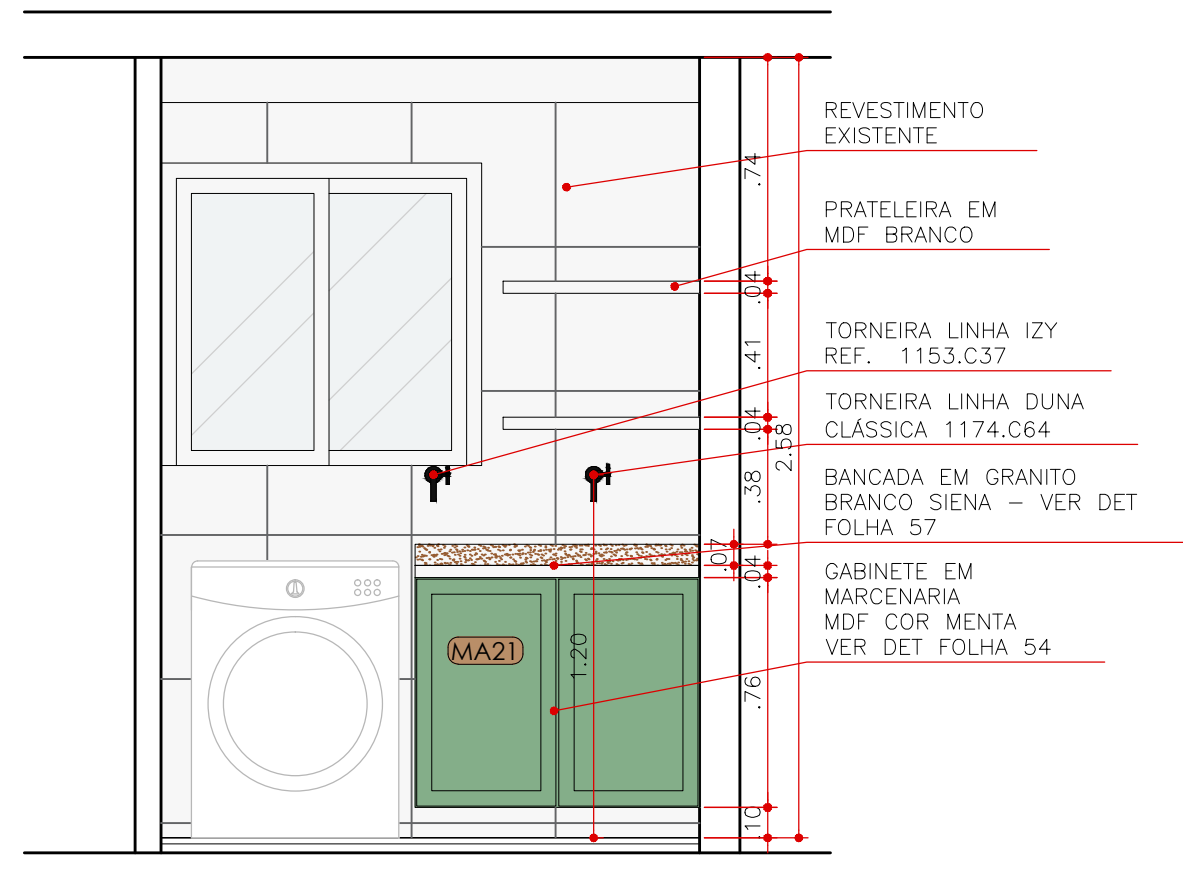
ELEVAÇÃO 12 LAVANDERIA ESCALA 1:25
