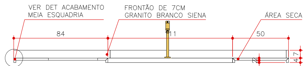
CORTE AA PE 01 ESCALA 1:20
