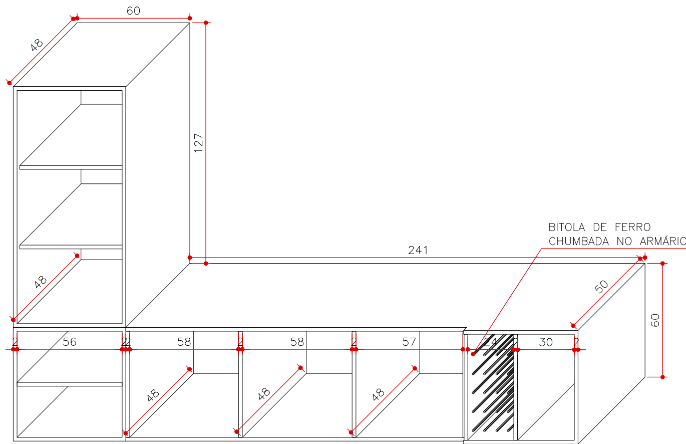
PERSPECTIVA SEM PORTAS MA 05 ESCALA 1:20 (MEDIDAS EM CM)
