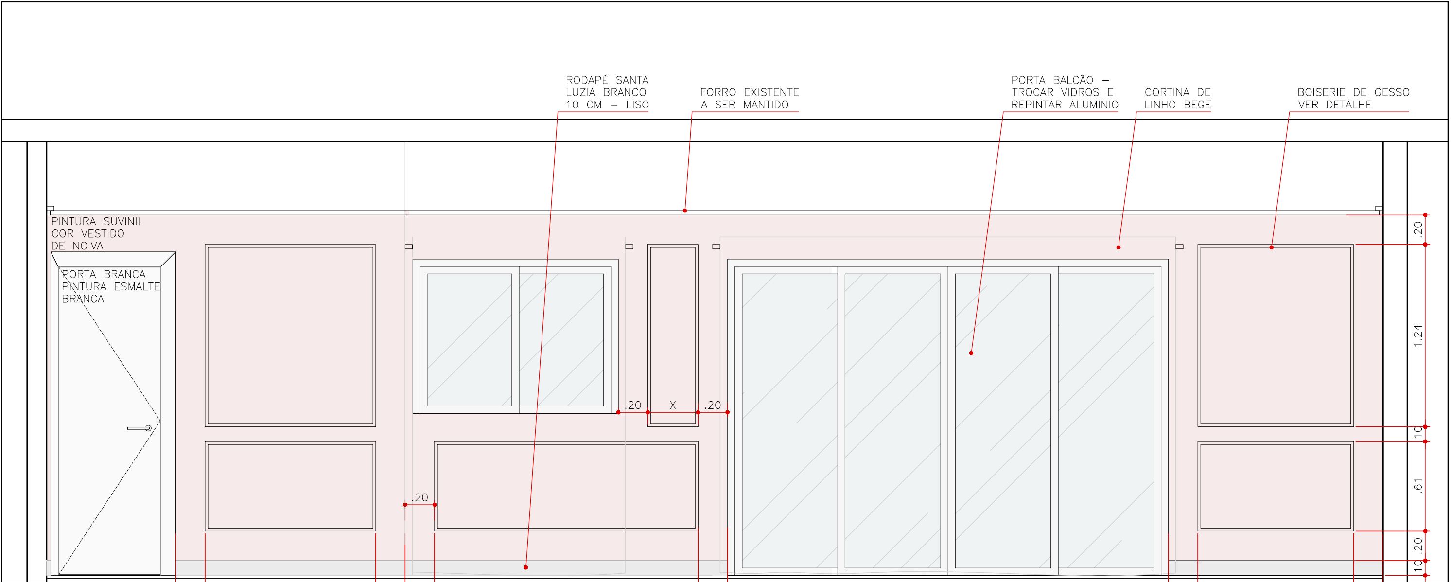
ELEVAÇÃO 2 SALA ESTAR E JANTAR ESCALA 1:25
