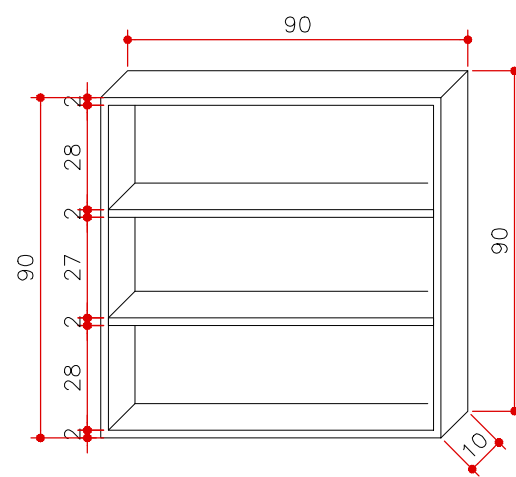
PERSPECTIVA SEM PORTA MA 10 ESCALA 1:20 (MEDIDAS EM CM)
