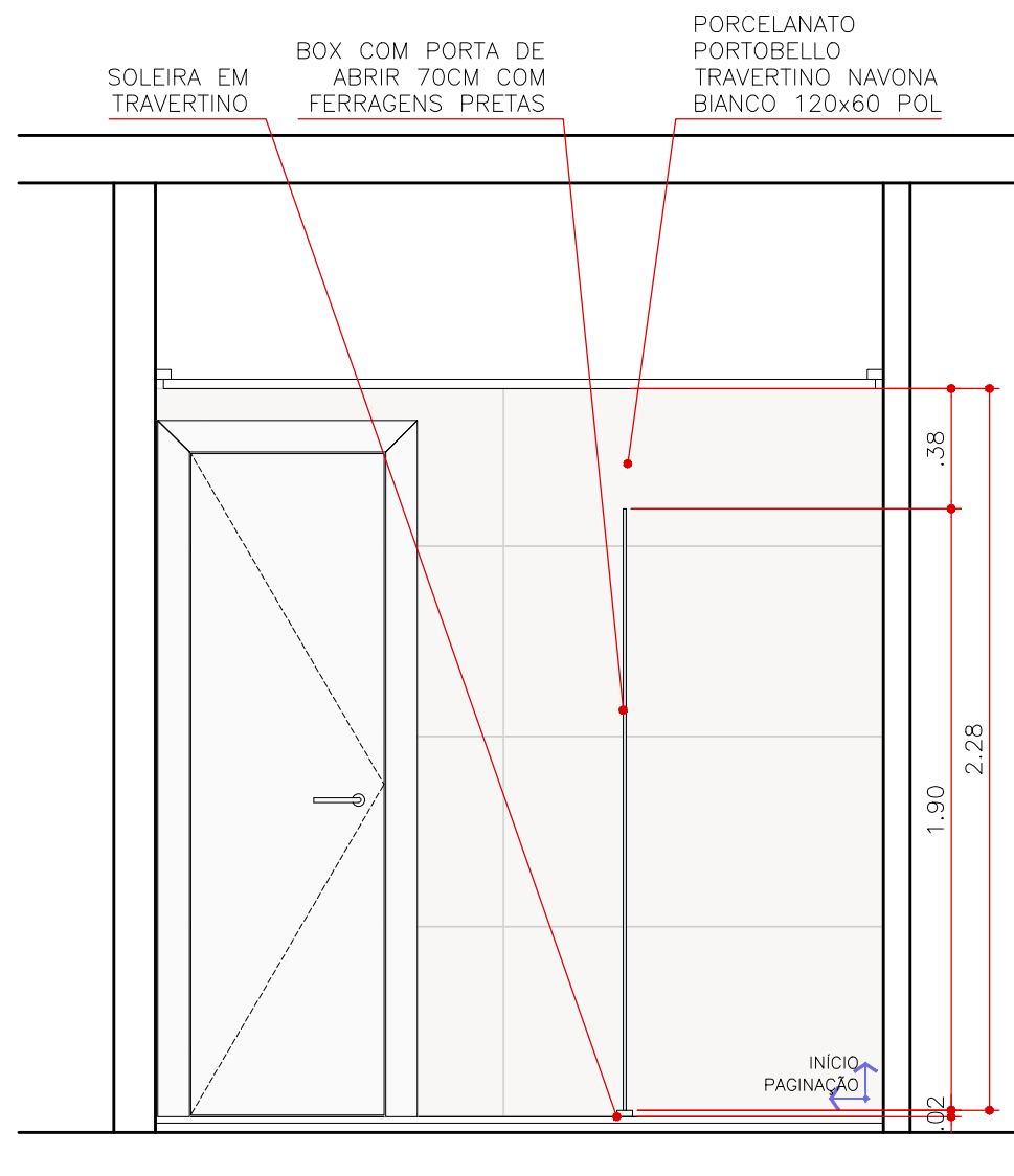
ELEVAÇÃO 38 BANHO MENINOS ESCALA 1:25
