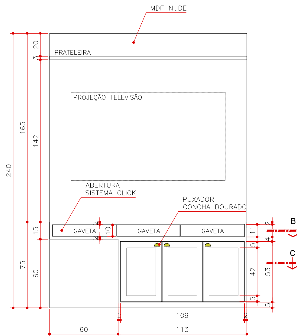
VISTA 1 MA 11 ESCALA 1:20 (MEDIDAS EM CM)
