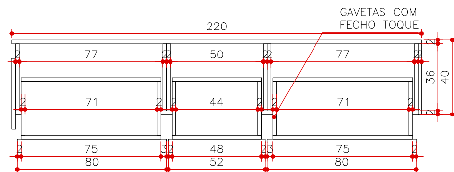
CORTE EE MA 07 ESCALA 1:20
