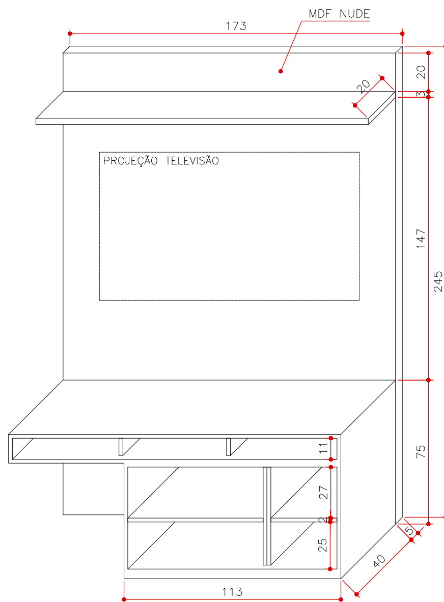
PERSPECTIVA SEM PORTAS MO 11 ESCALA 1:20 (MEDIDAS EM CM)
