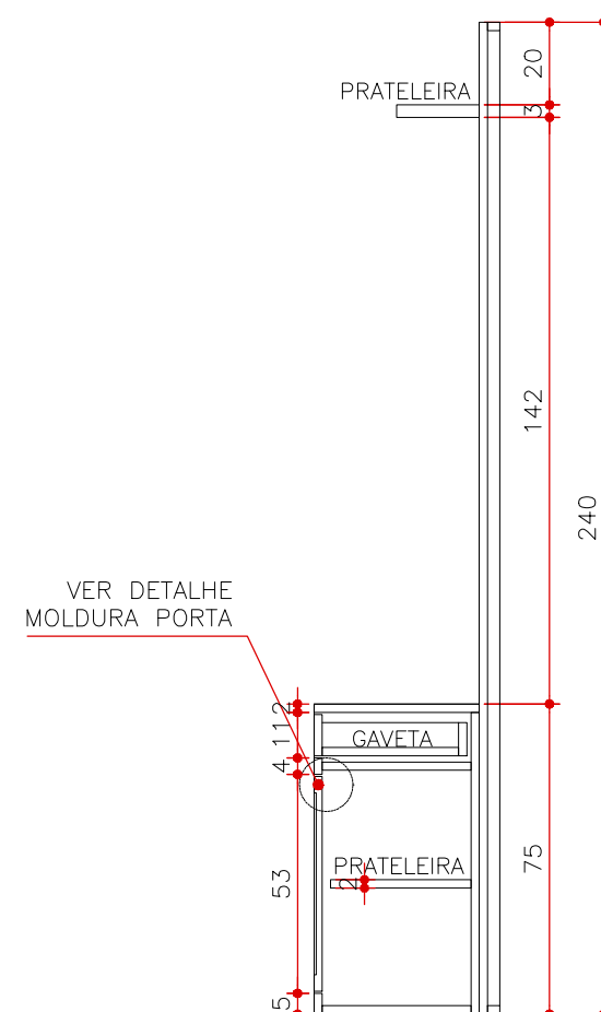
CORTE A MA 11 ESCALA 1:20 (MEDIDAS EM CM)
