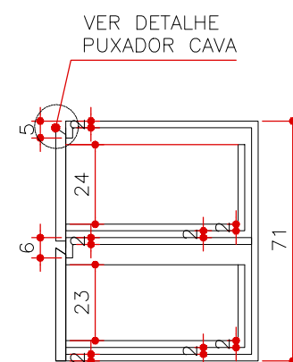
CORTE A MA 10 ESCALA 1:20 (MEDIDAS EM CM)
