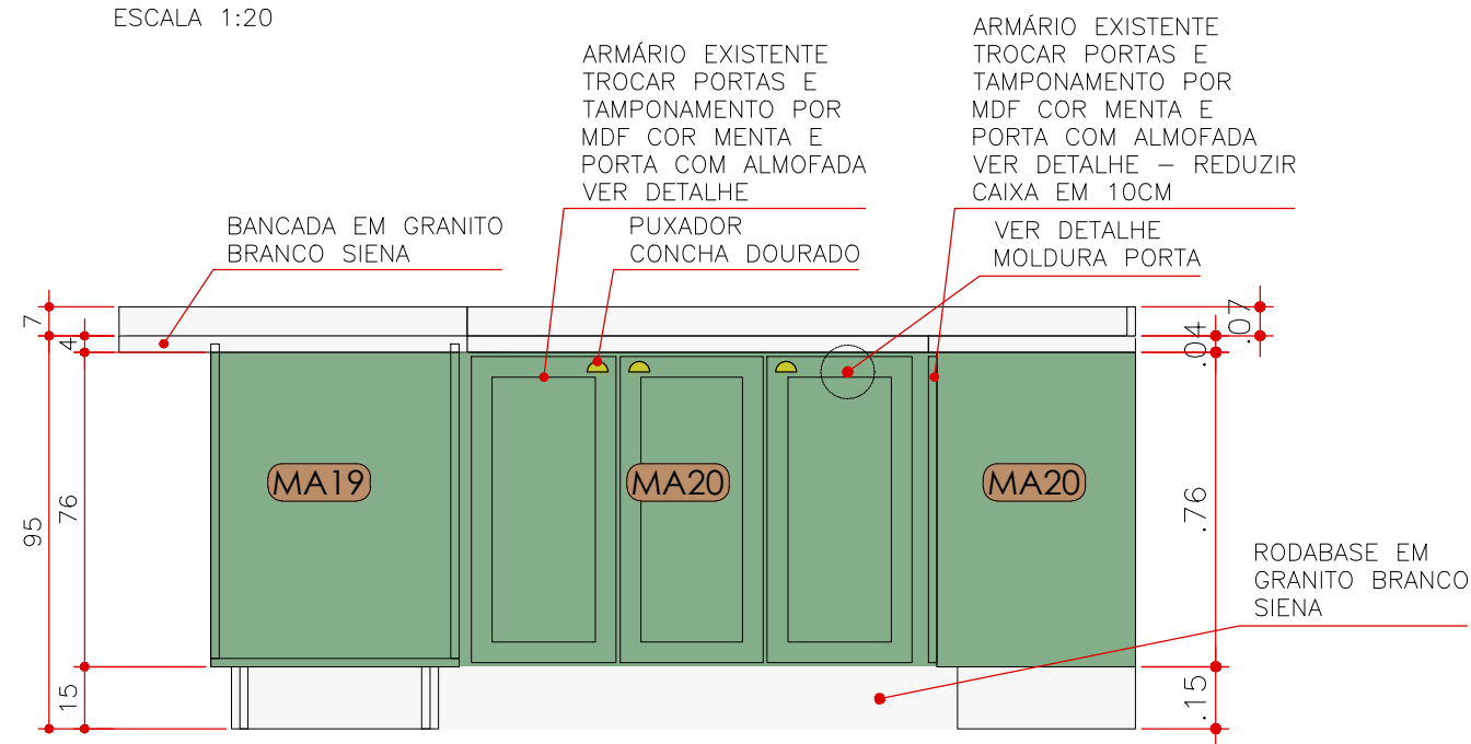
ELEVAÇÃO 1 MA 19 ESCALA 1:20
