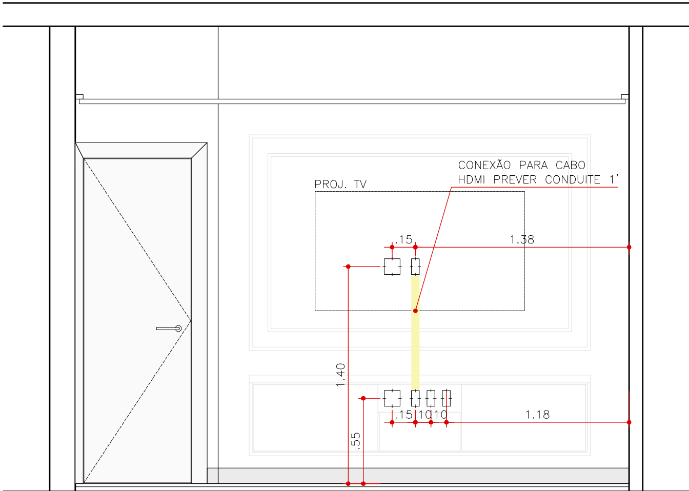
ELEVAÇÃO 1 – ELÉTRICA SALA ESTAR E JANTAR ESCALA 1:25
