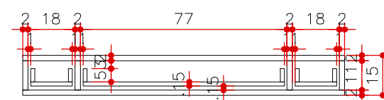
CORTE BB MA 04 ESCALA 1:20
