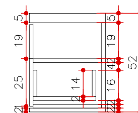
CORTE AA MA 07 ESCALA 1:20
