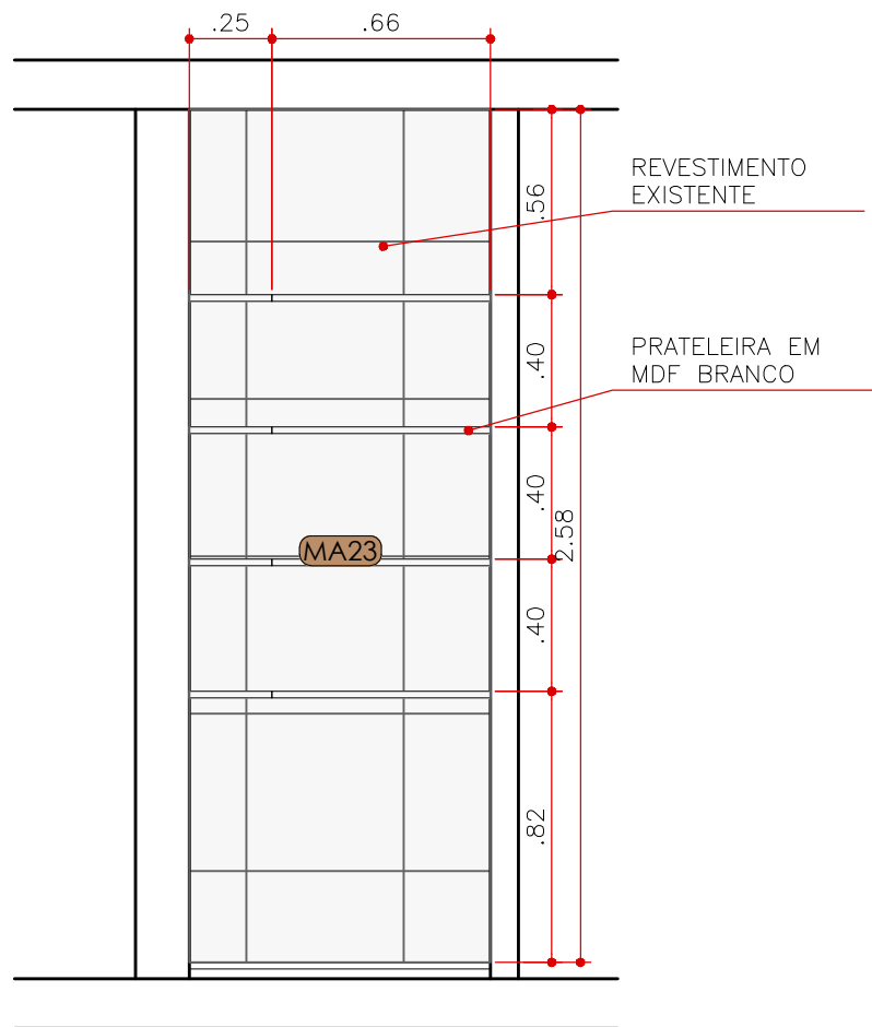
ELEVAÇÃO 13 DESPENSA ESCALA 1:25
