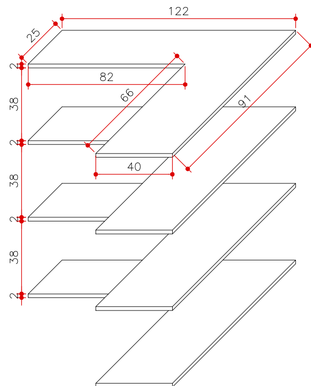
PERSPECTIVA MA 23 ESCALA 1:20
