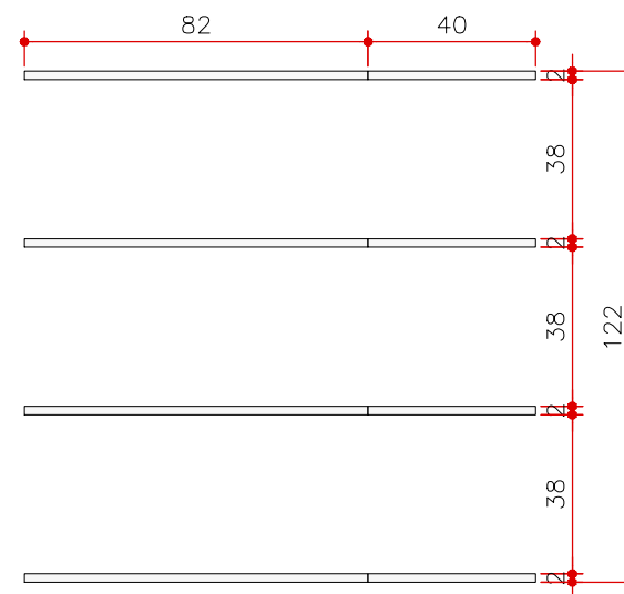
ELEVAÇÃO 1 MA 23 ESCALA 1:20
