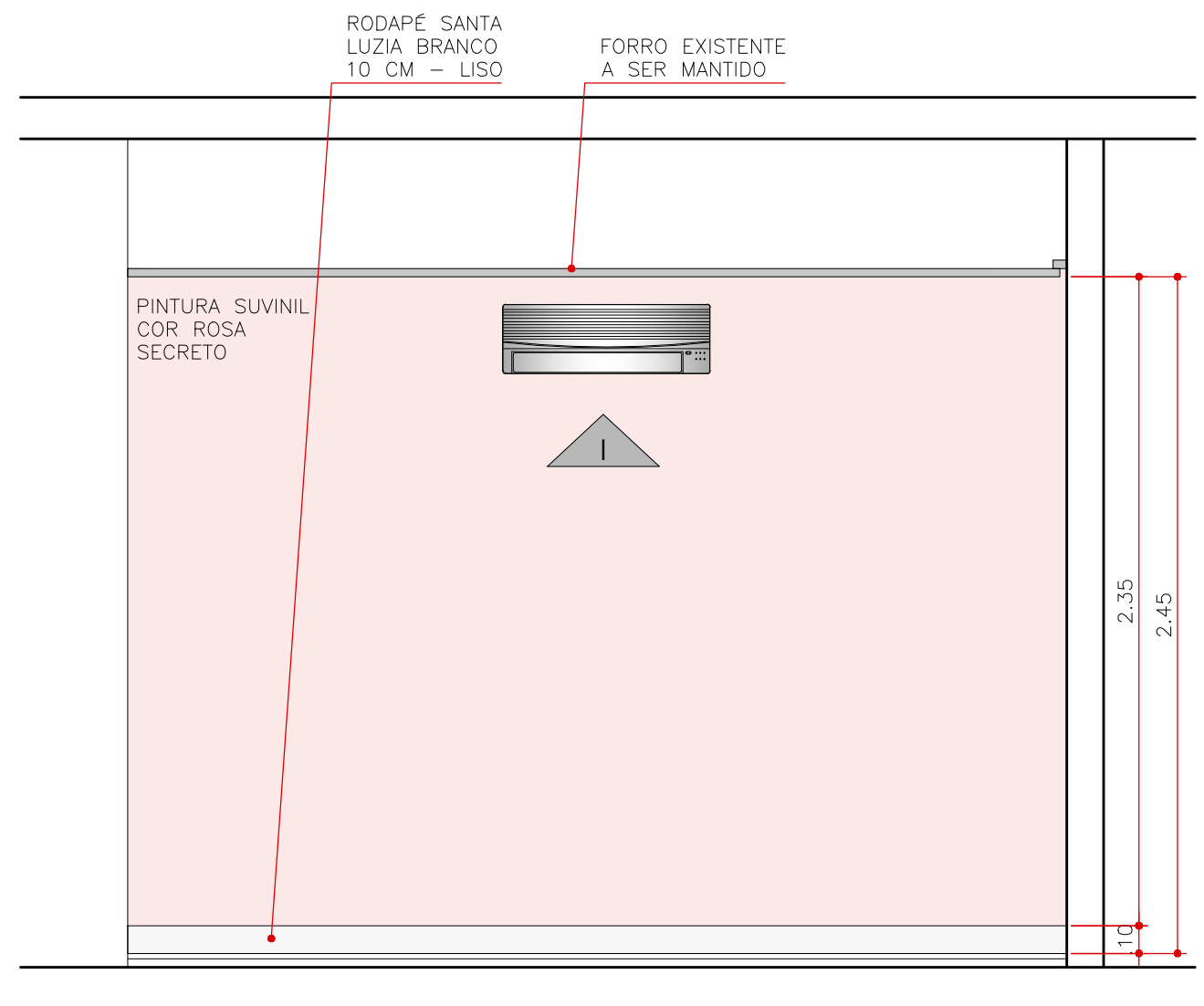
ELEVAÇÃO 22 QUARTO CASAL ESCALA 1:25
