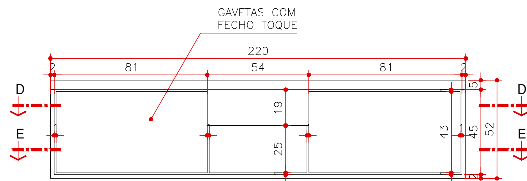
ELEVAÇÃO 1 MA 07 ESCALA 1:20
