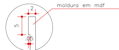
DETALHE MOLDURA PORTA ESCALA 1:5 (MEDIDAS EM CM)
