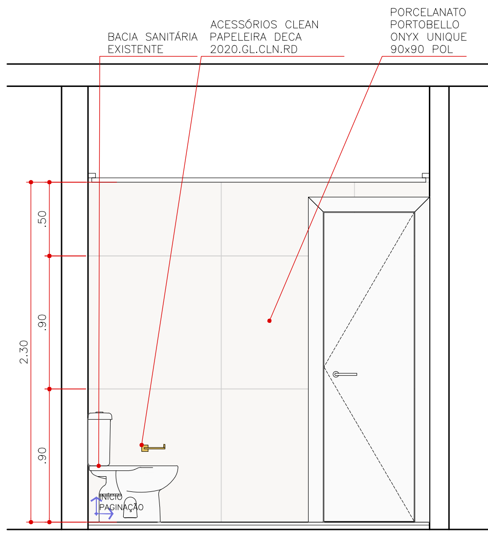
ELEVAÇÃO 26 BANHO CASAL ESCALA 1:25
