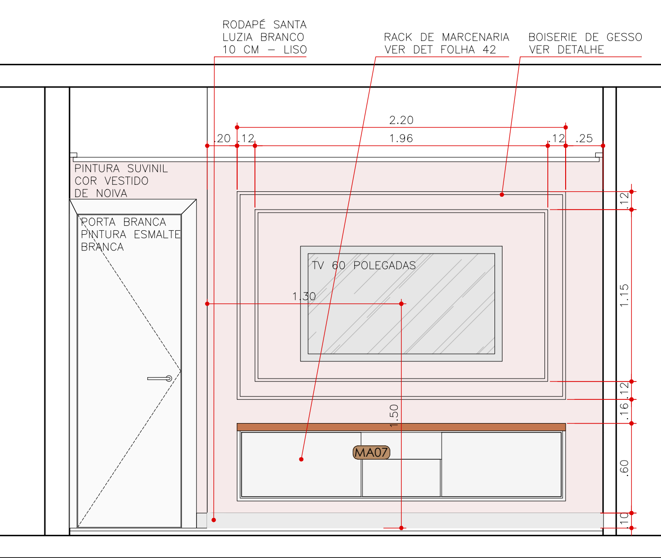
ELEVAÇÃO 1 SALA ESTAR E JANTAR ESCALA 1:25
