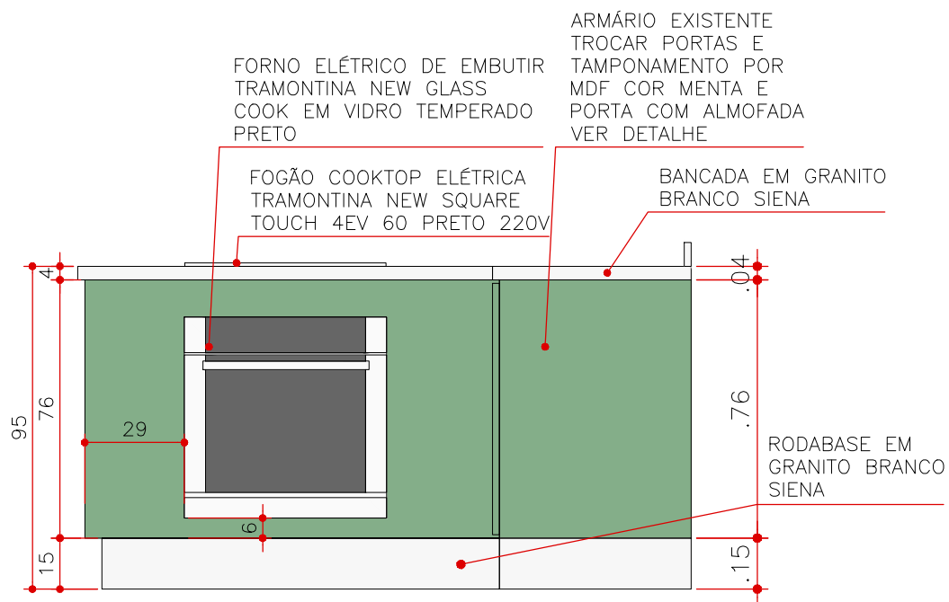
ELEVAÇÃO 3 MA 19 ESCALA 1:20
