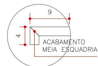
DETALHE MEIA ESQUADRIA ESCALA 1:5
