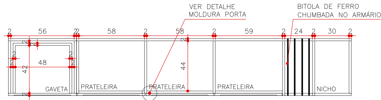
CORTE BB MA 05 ESCALA 1:20 (MEDIDAS EM CM)
