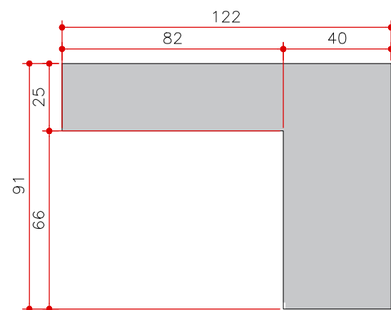
PLANTA MA 23 ESCALA 1:20
