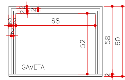
CORTE B MA 18 ESCALA 1:20 (MEDIDAS EM CM)
