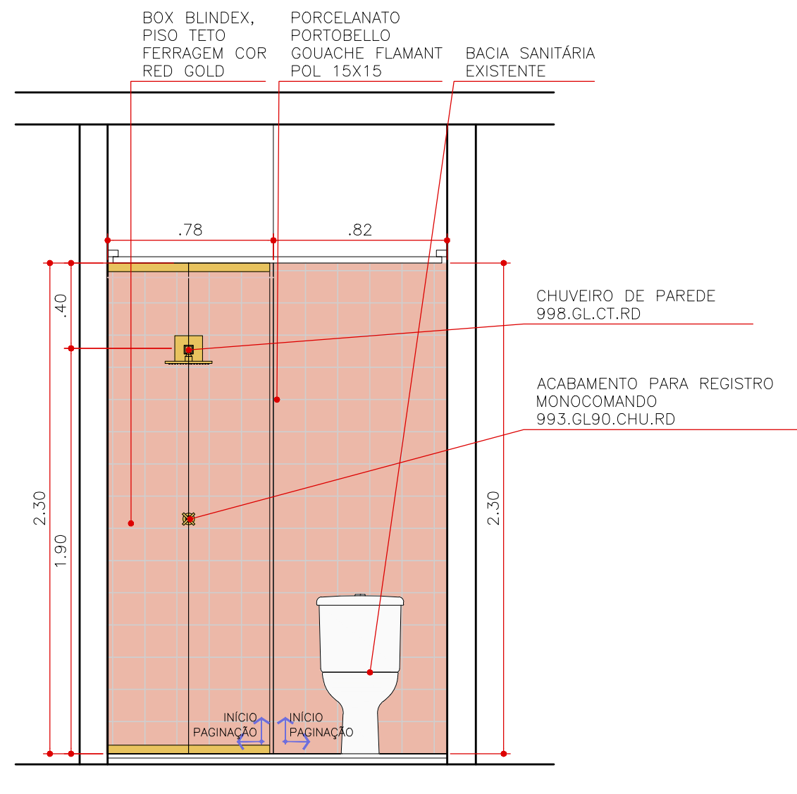
ELEVAÇÃO 25 BANHO CASAL ESCALA 1:25
