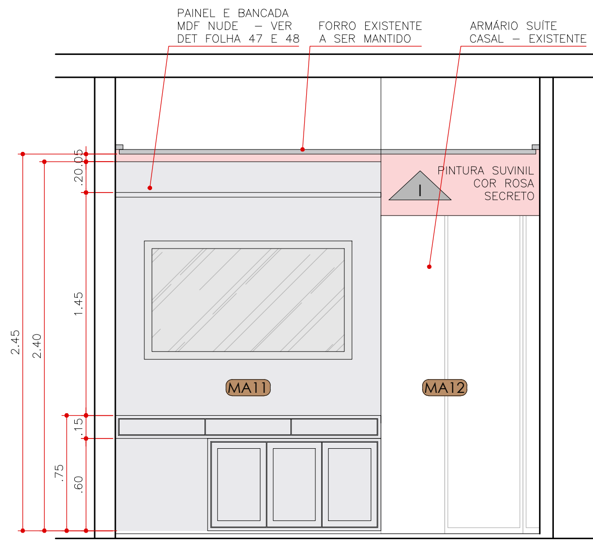
ELEVAÇÃO 21 QUARTO CASAL ESCALA 1:25
