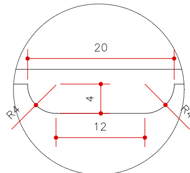
DETALHE PUXADOR GAVETA ESCALA 1:5 (MEDIDAS EM CM)
