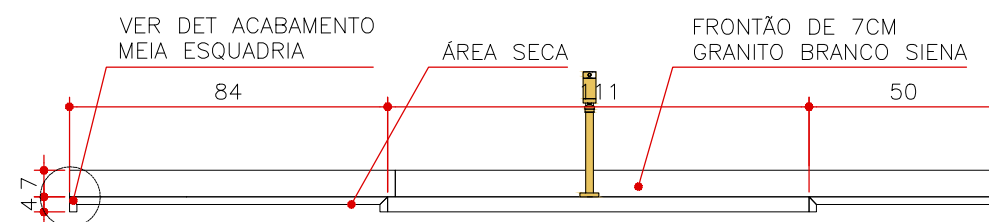
CORTE BB PE 01 ESCALA 1:20
