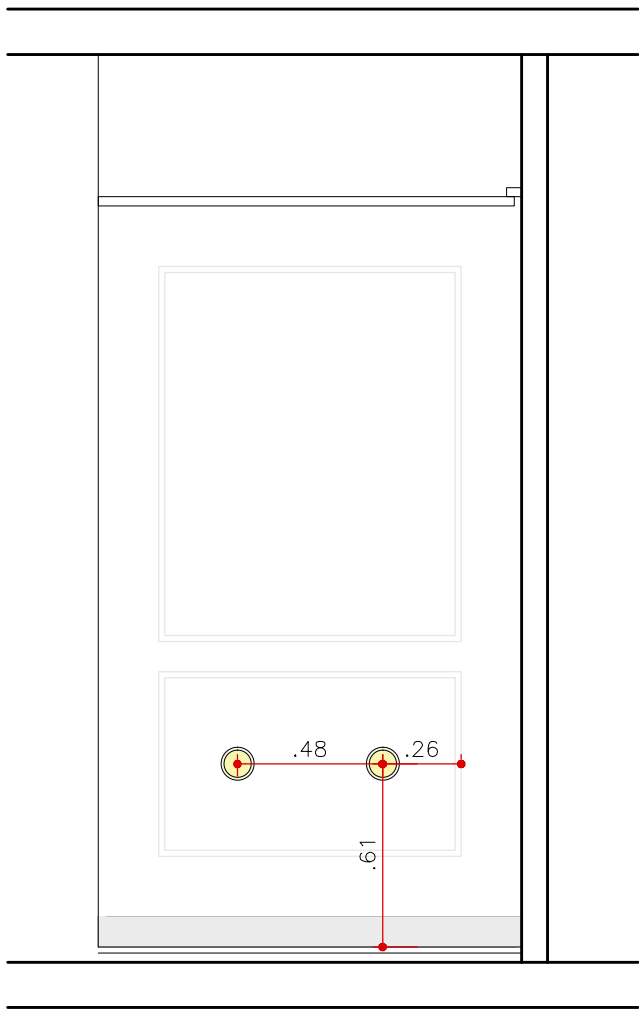
ELEVAÇÃO 40 – ELÉTRICA HALL BANHEIROS ESCALA 1:25
