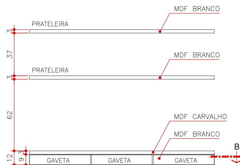
VISTA 1 MA 16 ESCALA 1:20 (MEDIDAS EM CM)
