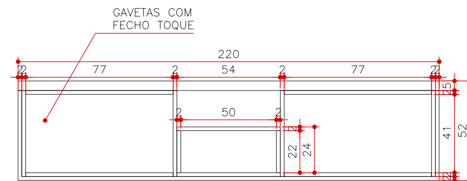
CORTE CC MA 07 ESCALA 1:20
