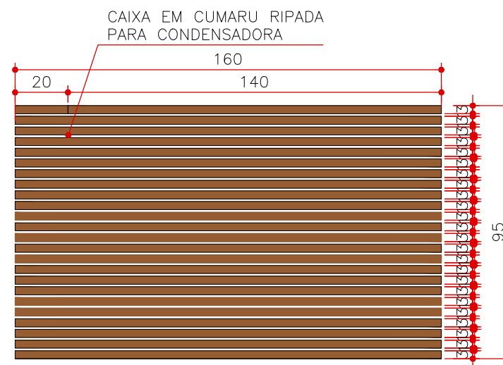
CORTE BB MA 09 ESCALA 1:20
