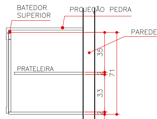
CORTE AA MA 08 ESCALA 1:20
