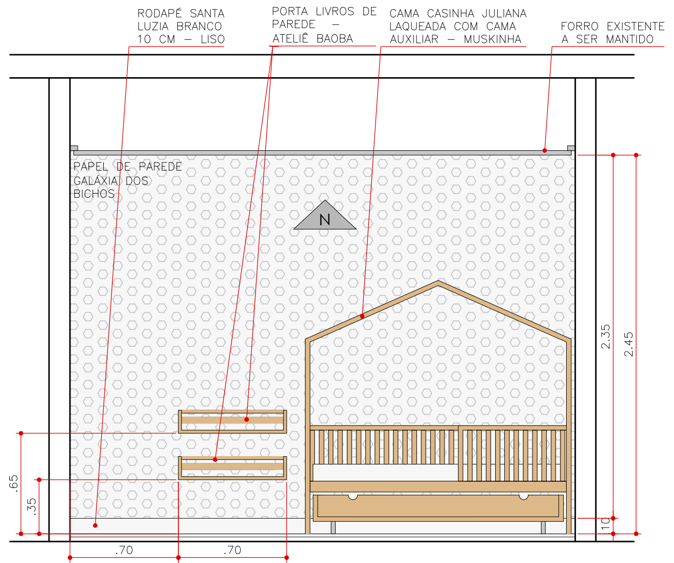
ELEVAÇÃO 30 QUARTO MIGUEL ESCALA 1:25
