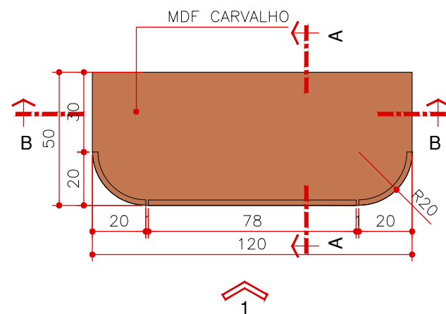
PLANTA MA 04 ESCALA 1:20
