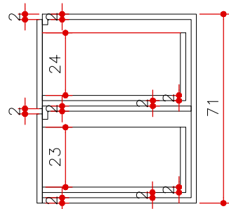
CORTE A MA 18 ESCALA 1:20 (MEDIDAS EM CM)
