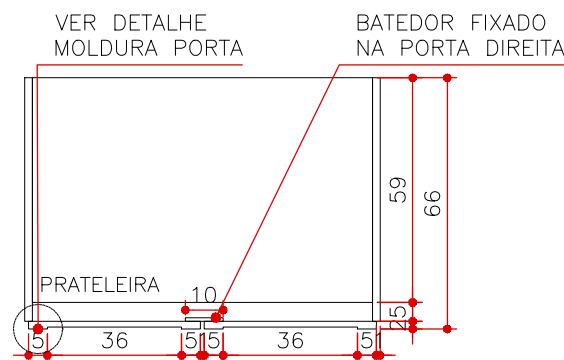
CORTE BB MA 21 ESCALA 1:20
