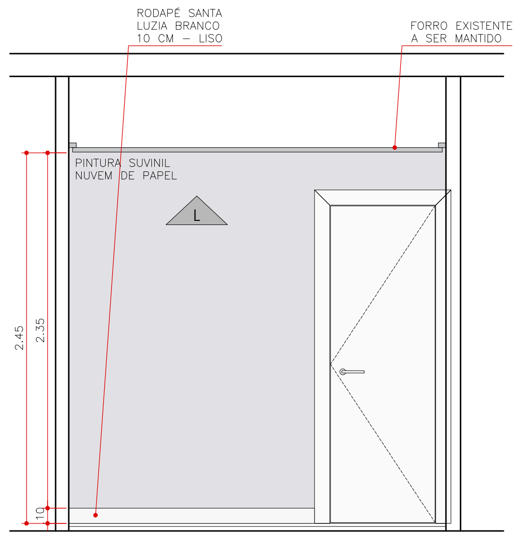
ELEVAÇÃO 31 QUARTO MIGUEL ESCALA 1:25
