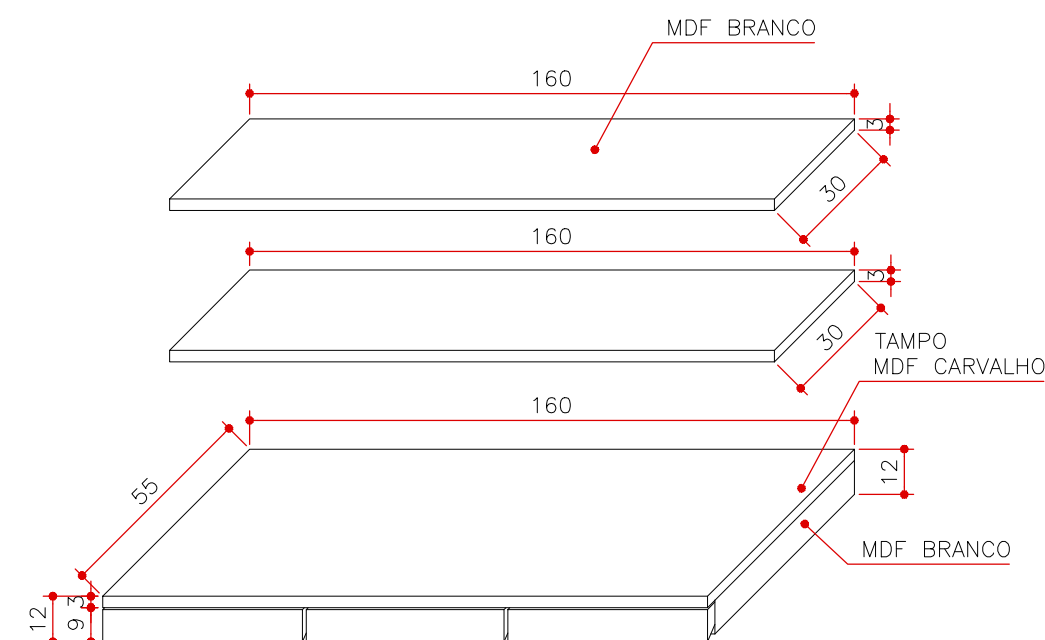
PERSPECTIVA MA 16 ESCALA 1:20 (MEDIDAS EM CM)
