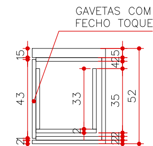
CORTE BB MA 07 ESCALA 1:20
