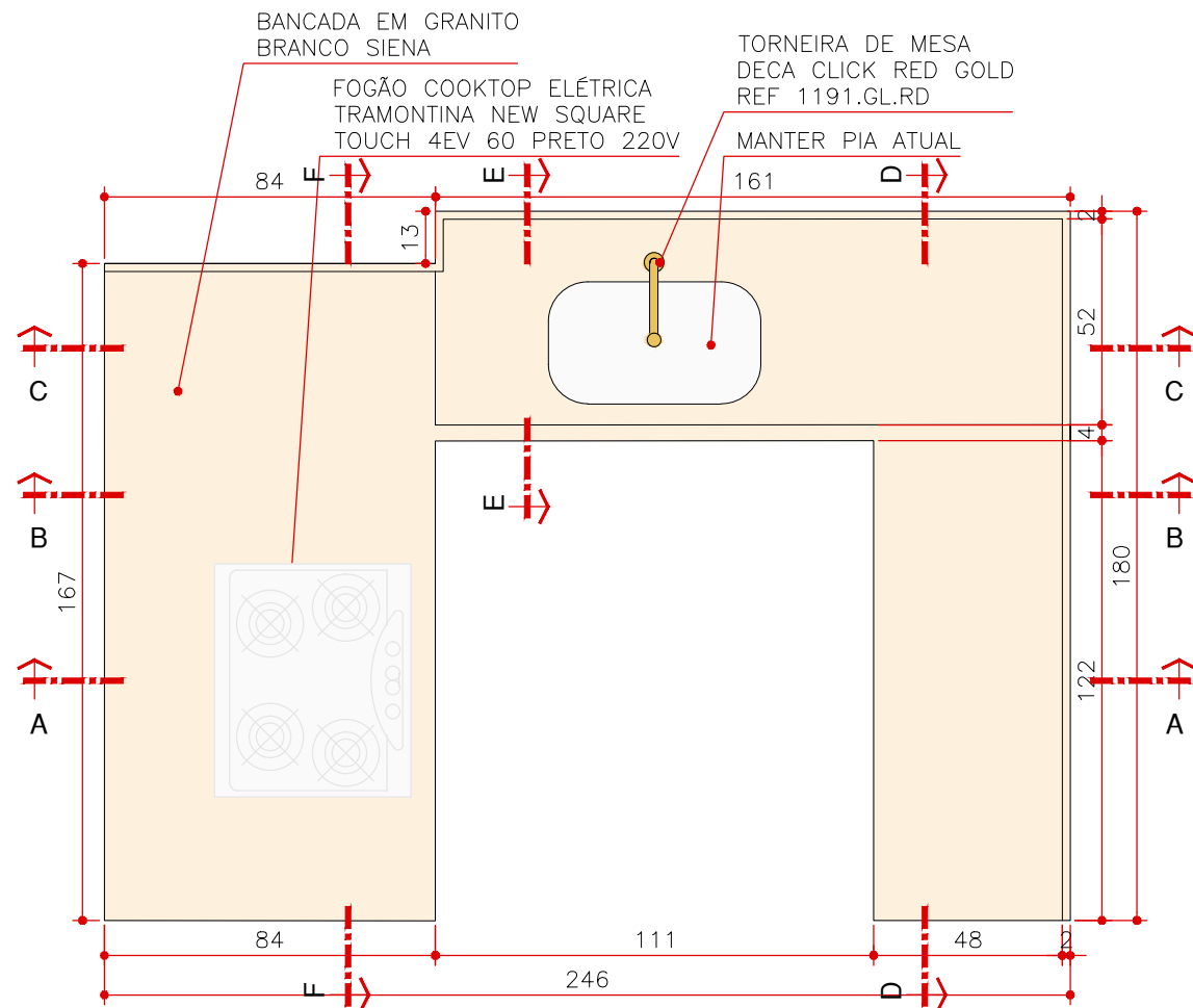
PLANTA PE 01 ESCALA 1:20
