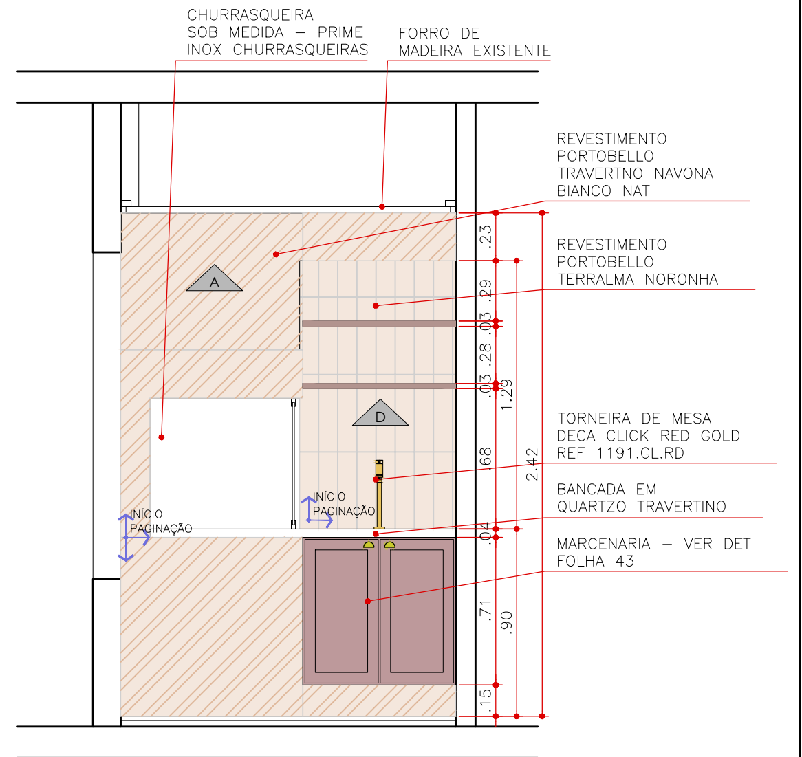
ELEVAÇÃO 15 VARANDA ESCALA 1:25
