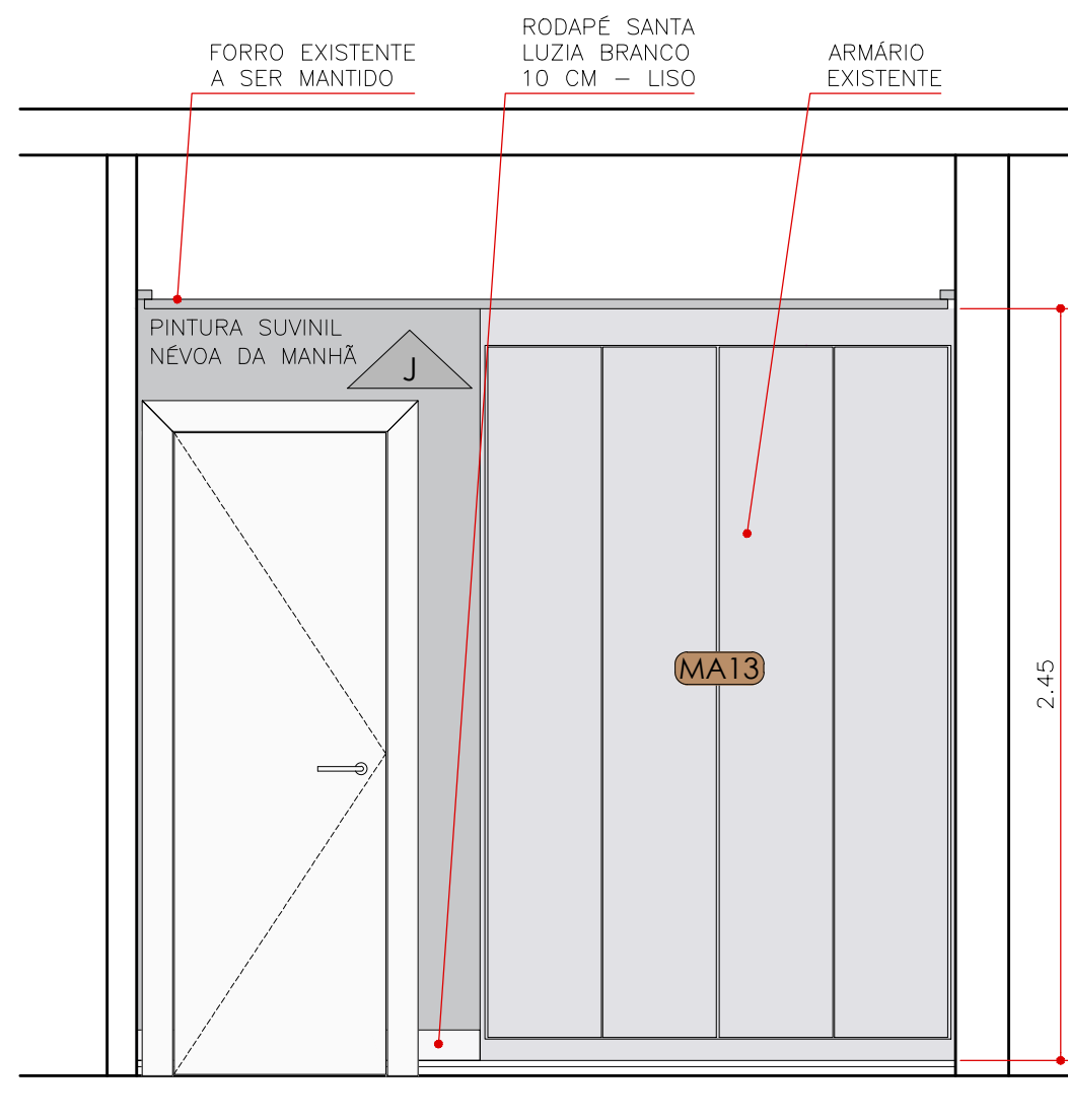
ELEVAÇÃO 35 QUARTO GUSTAVO ESCALA 1:25
