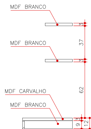
VISTA 2 MA 16 ESCALA 1:20 (MEDIDAS EM CM)
