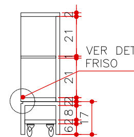
CORTE AA MA 06 ESCALA 1:20
