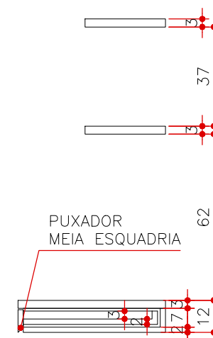
CORTE A MA 16 ESCALA 1:20 (MEDIDAS EM CM)
