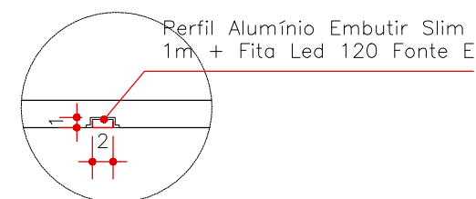
DETALHE PERFIL LED EMBUTIDO ESCALA 1:5 (MEDIDAS EM CM)
