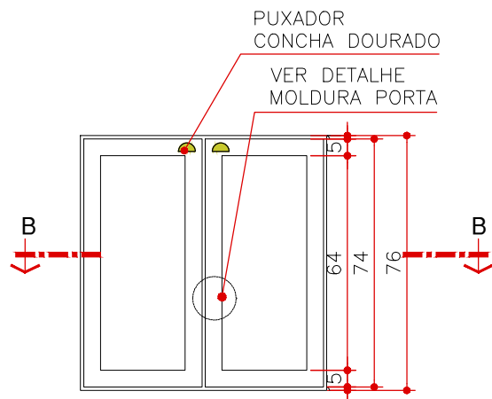
ELEVAÇÃO 1 MA 21 ESCALA 1:20
