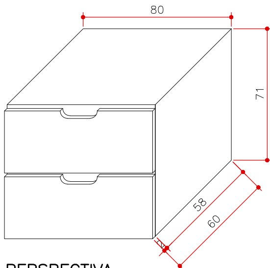
PERSPECTIVA MA 18 ESCALA 1:20 (MEDIDAS EM CM)
