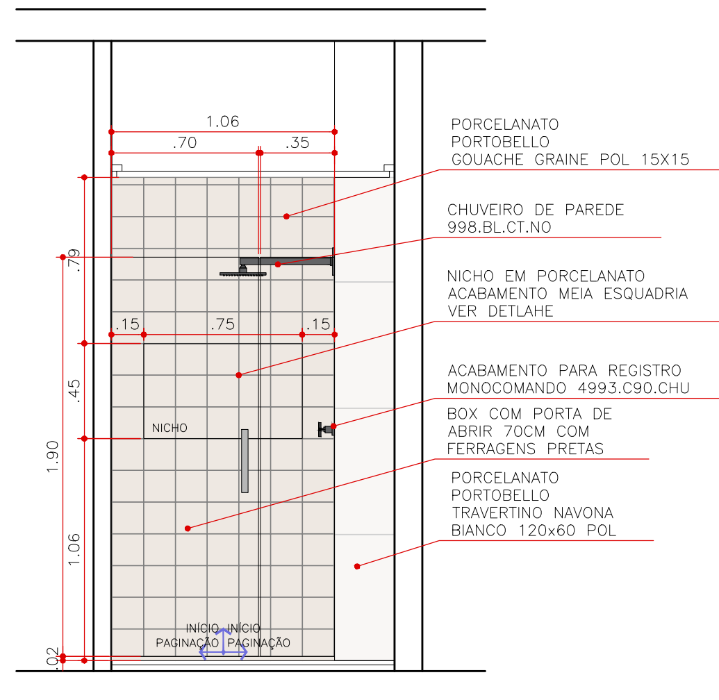
ELEVAÇÃO 39 BANHO MENINOS ESCALA 1:25
