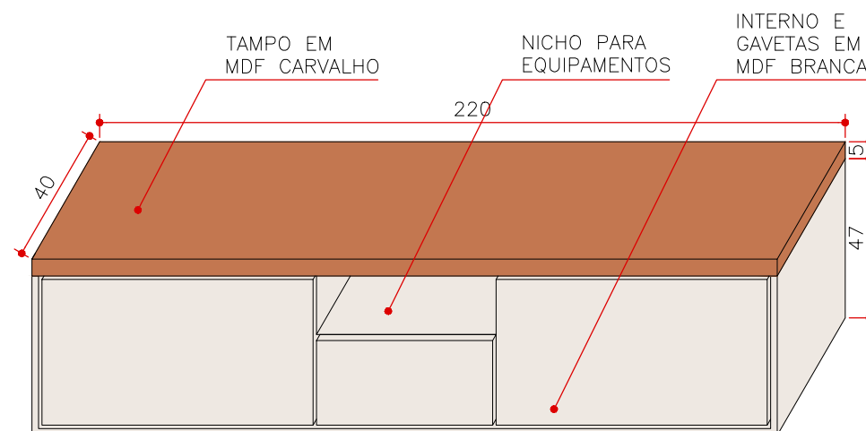
PERSPECTIVA MA 07 ESCALA 1:20
