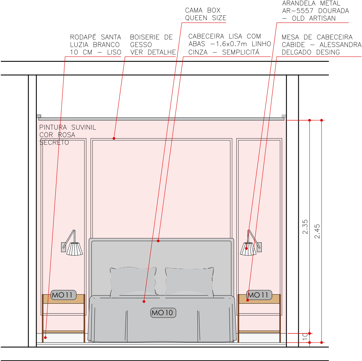
ELEVAÇÃO 19 QUARTO CASAL ESCALA 1:25
