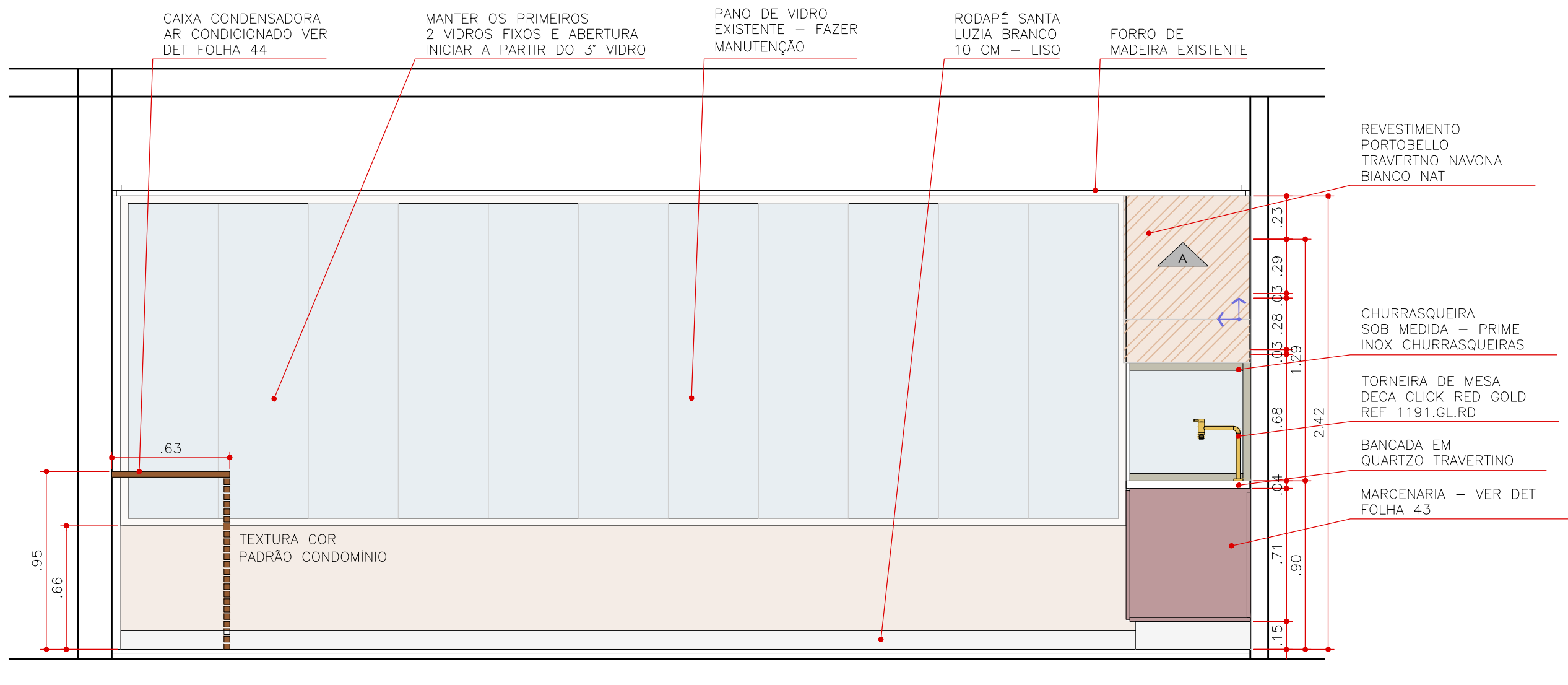
ELEVAÇÃO 18 VARANDA ESCALA 1:25
