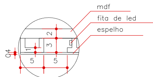
DETALHE ESPELHO ESCALA 1:5 (MEDIDAS EM CM)
