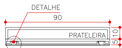
CORTE B MA 10 ESCALA 1:20 (MEDIDAS EM CM)
