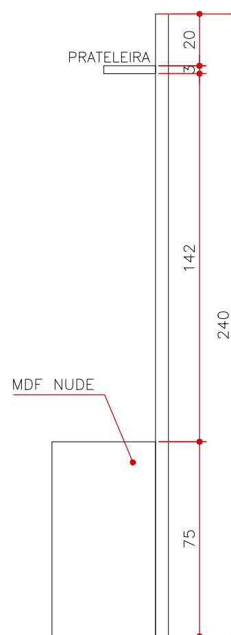
VISTA 2 MA 11 ESCALA 1:20 (MEDIDAS EM CM)
