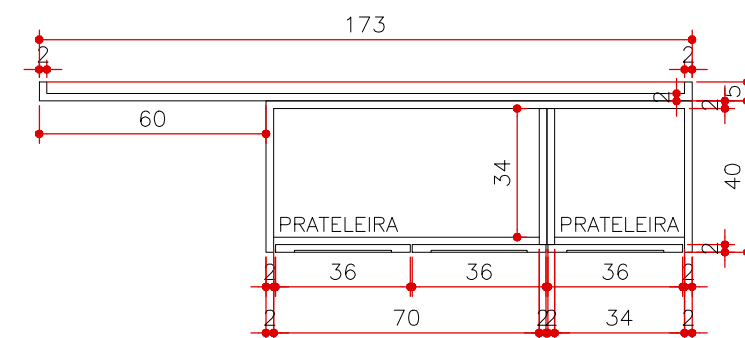
CORTE B MA 11 ESCALA 1:20 (MEDIDAS EM CM)
