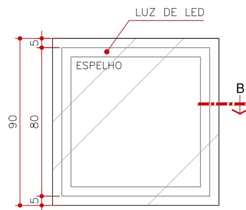
VISTA 1 MA 10 ESCALA 1:20 (MEDIDAS EM CM)
