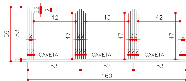
CORTE B MA 16 ESCALA 1:20 (MEDIDAS EM CM)
