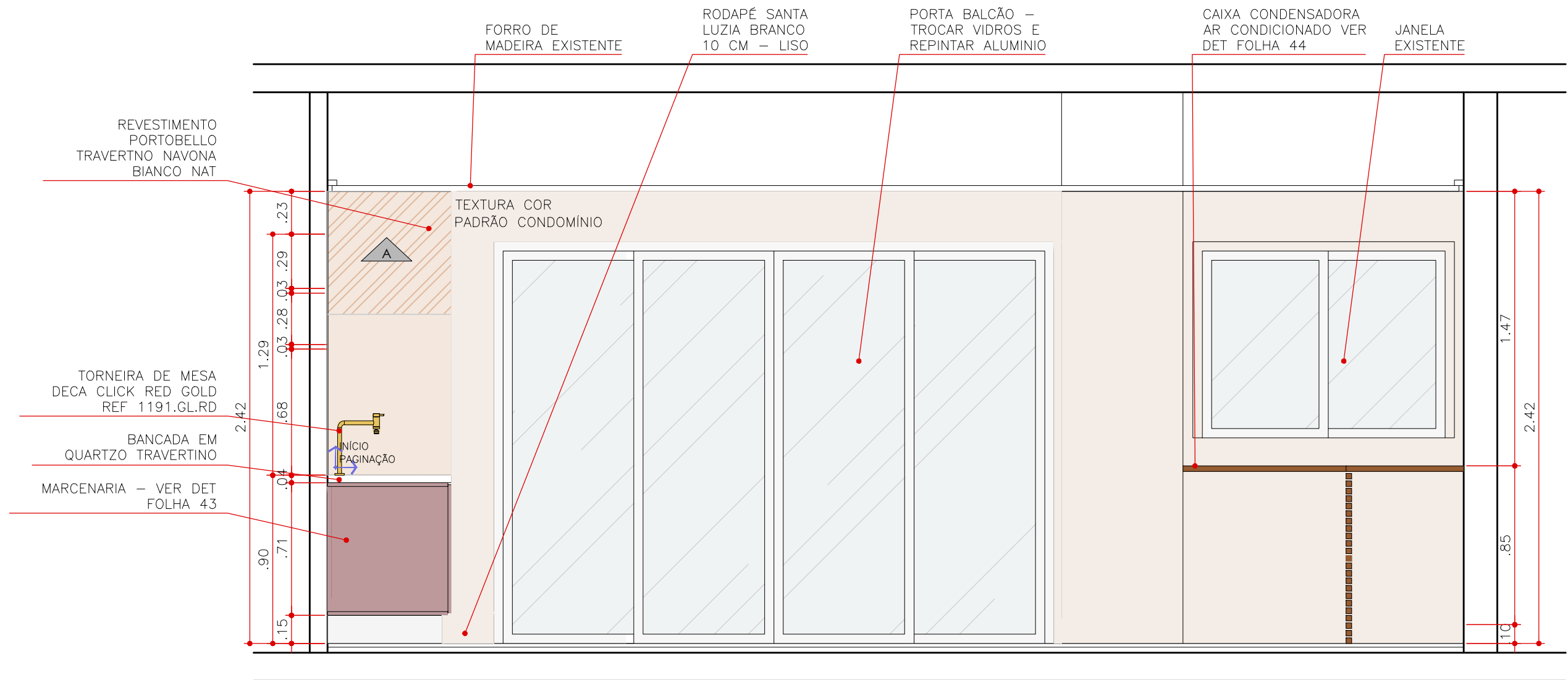
ELEVAÇÃO 16 VARANDA ESCALA 1:25
