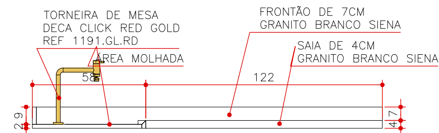
CORTE EE PE 01 ESCALA 1:20
