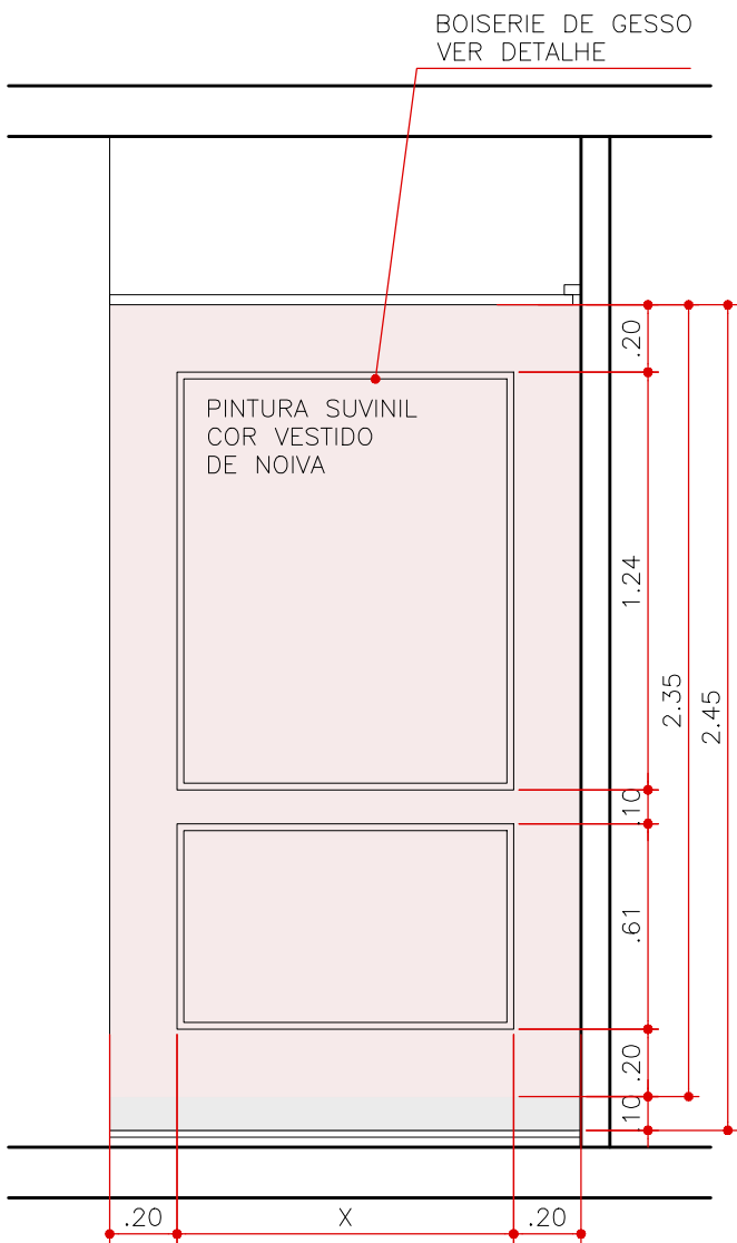
ELEVAÇÃO 40 HALL BANHEIROS ESCALA 1:20
