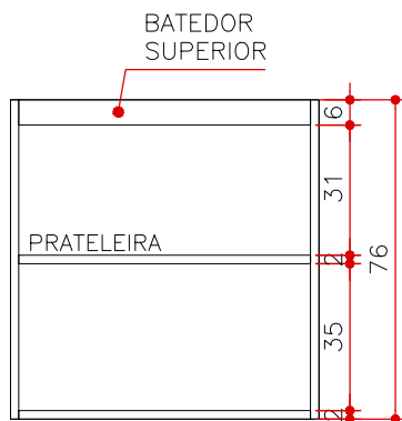
ELEVAÇÃO 1 - S/ PORTA MA 21 ESCALA 1:20
