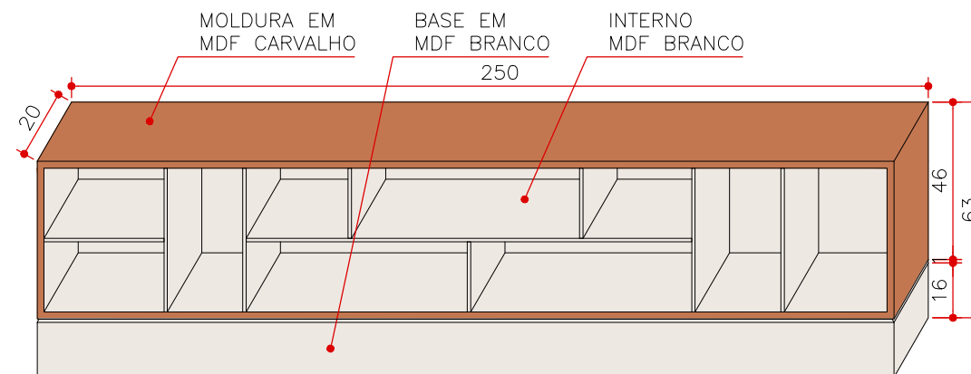
PERSPECTIVA MA 06 ESCALA 1:20
