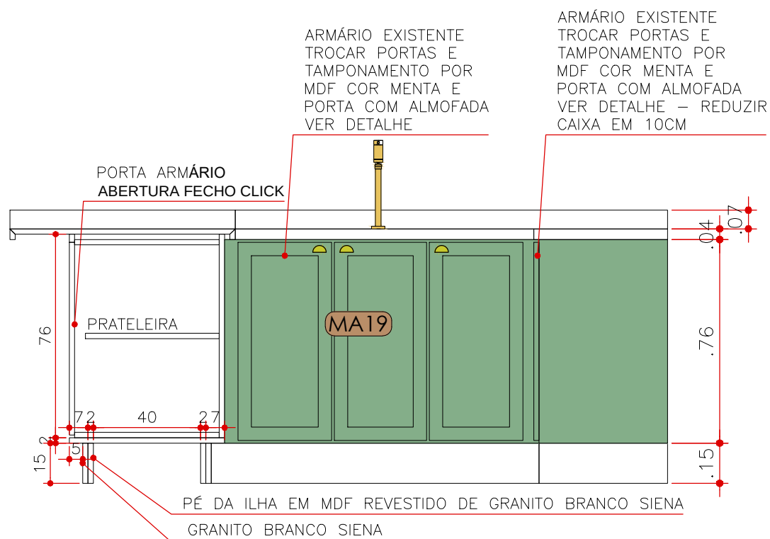
CORTE BB MA 19 ESCALA 1:20
