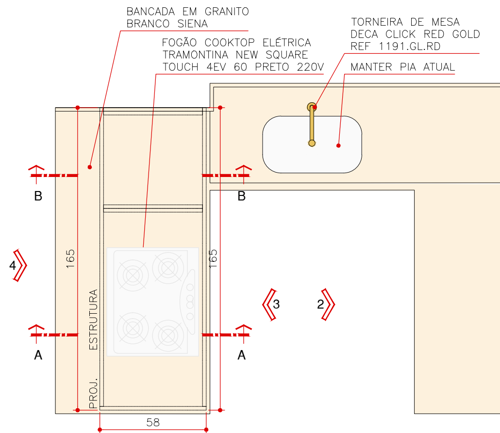
PLANTA MA 19 ESCALA 1:20
