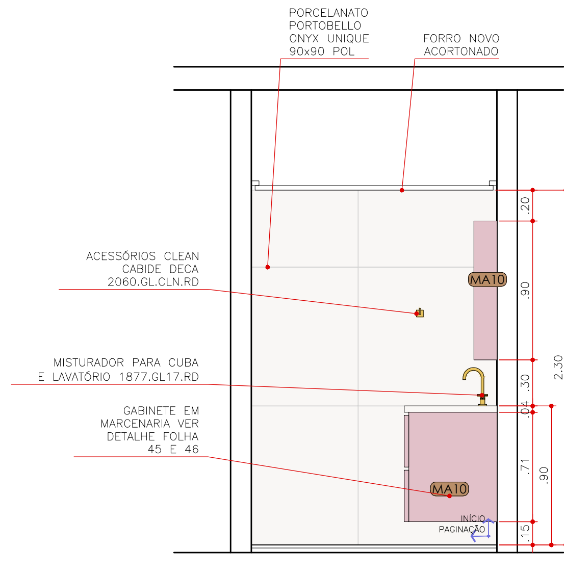
ELEVAÇÃO 27 BANHO CASAL ESCALA 1:25
