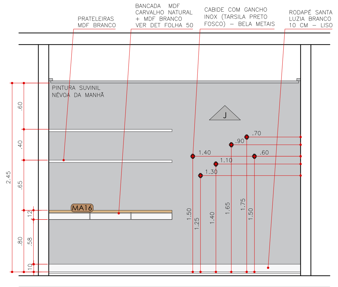
ELEVAÇÃO 32 QUARTO GUSTAVO ESCALA 1:25
