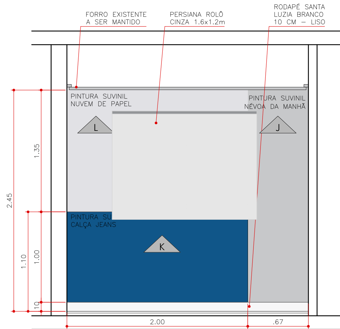
ELEVAÇÃO 33 QUARTO GUSTAVO ESCALA 1:25
