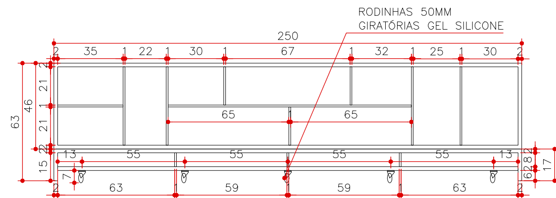
CORTE BB MA 06 ESCALA 1:20
