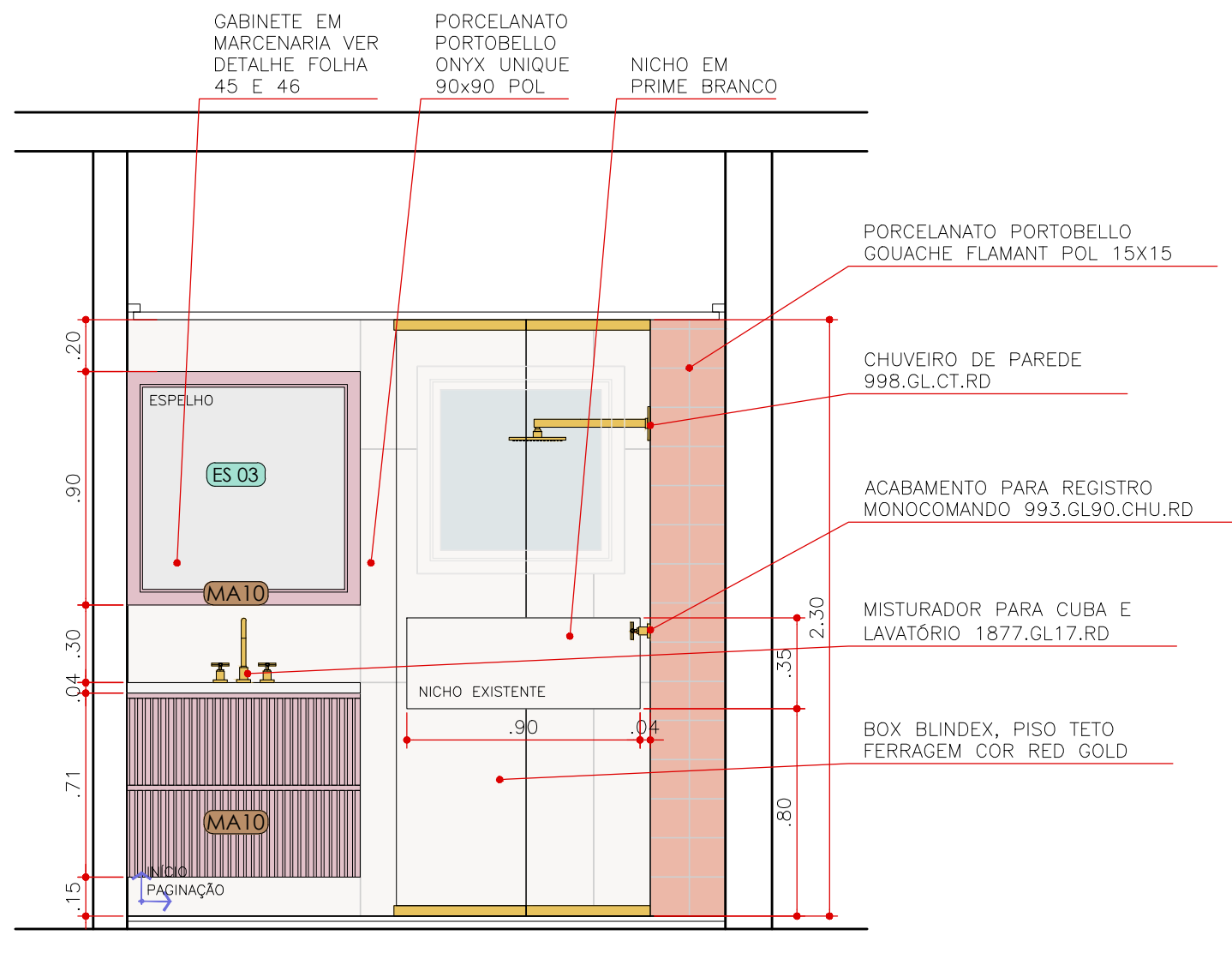
ELEVAÇÃO 24 BANHO CASAL ESCALA 1:25
