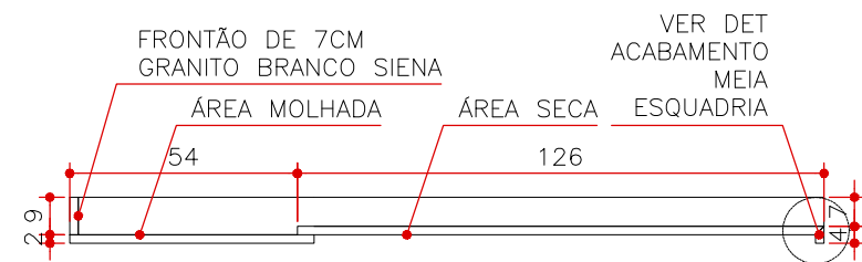
CORTE DD PE 01 ESCALA 1:20
