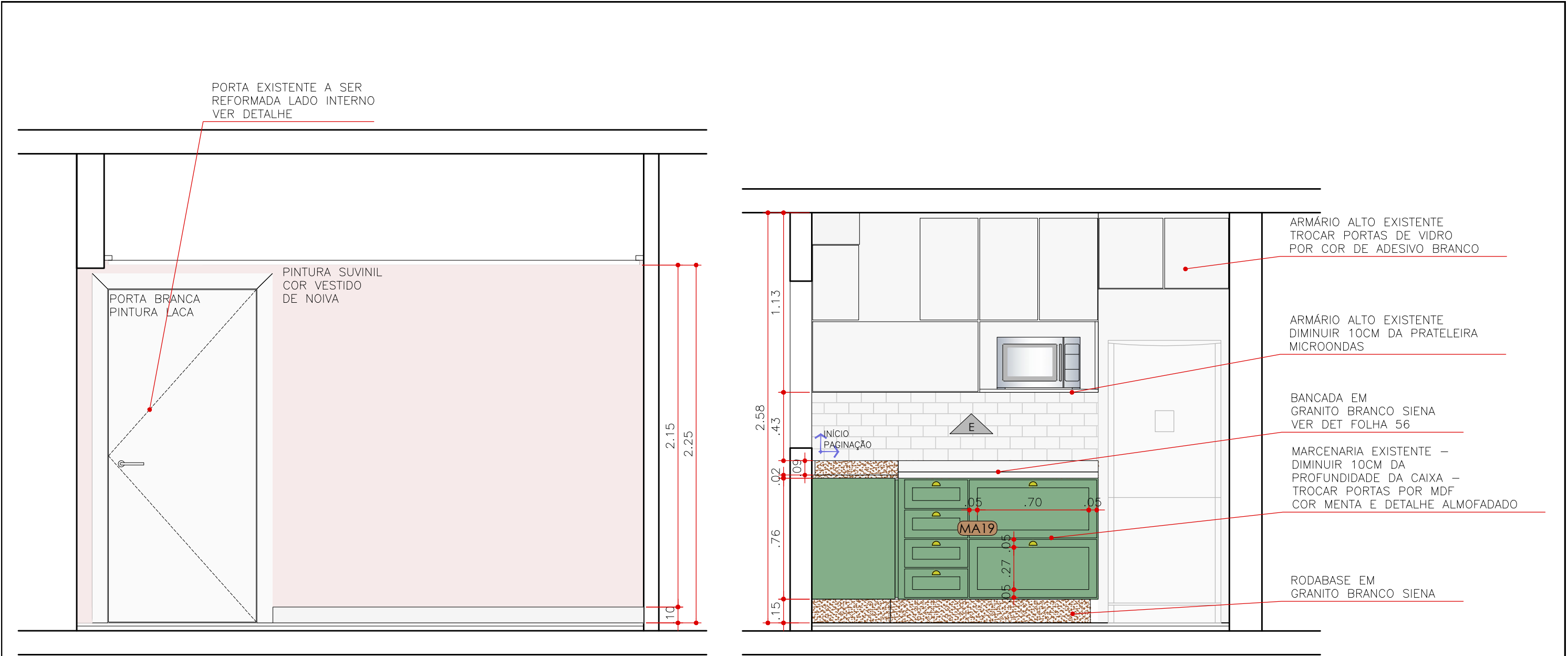
ELEVAÇÃO 7 HALL DE ENTRADA / HOME OFFICE ESCALA 1:25
