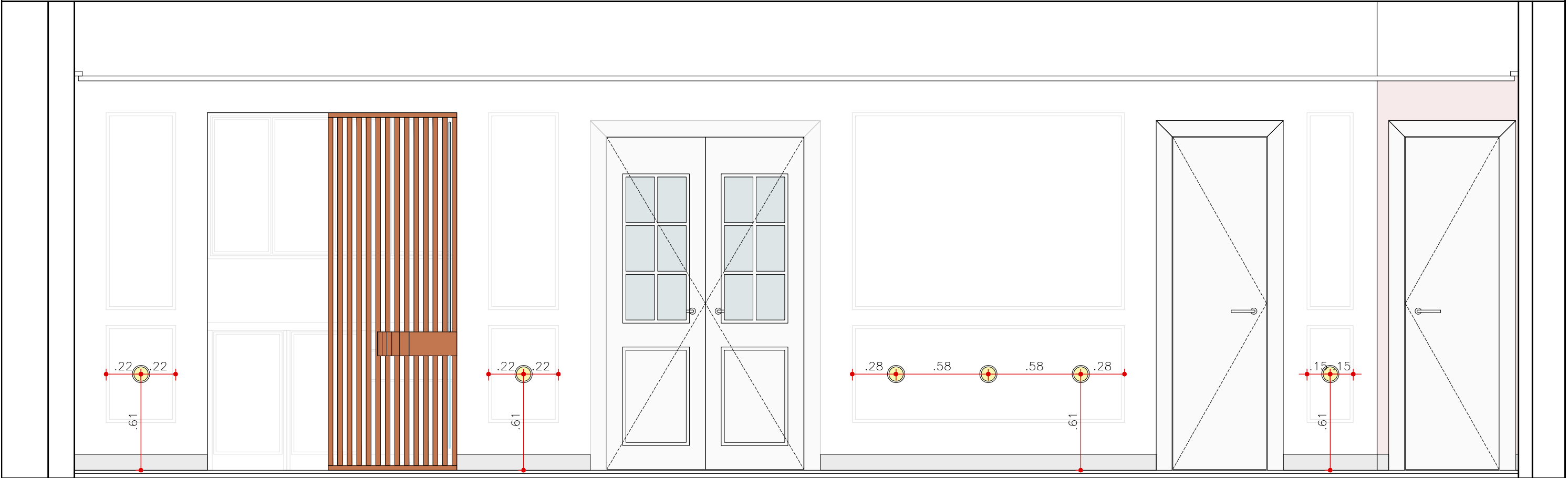
ELEVAÇÃO 4 – ELÉTRICA SALA ESTAR E JANTAR ESCALA 1:25
