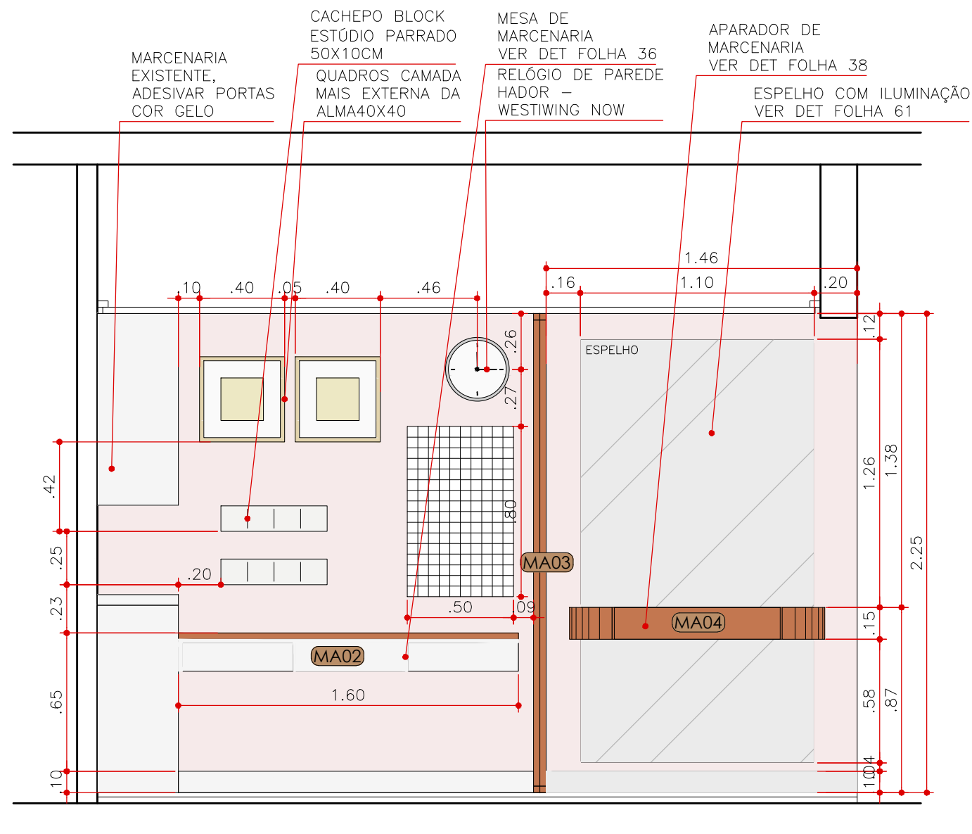
ELEVAÇÃO 5 HALL DE ENTRADA / HOME OFFICE ESCALA 1:25
