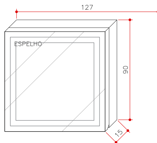
PERSPECTIVA MA 10 ESCALA 1:20 (MEDIDAS EM CM)
