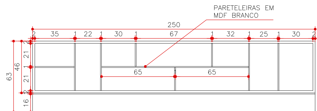
ELEVÇÃO 1 MA 06 ESCALA 1:20
