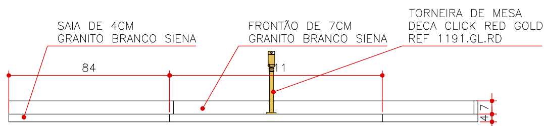
ELEVAÇÃO 1 PE 01 ESCALA 1:20
