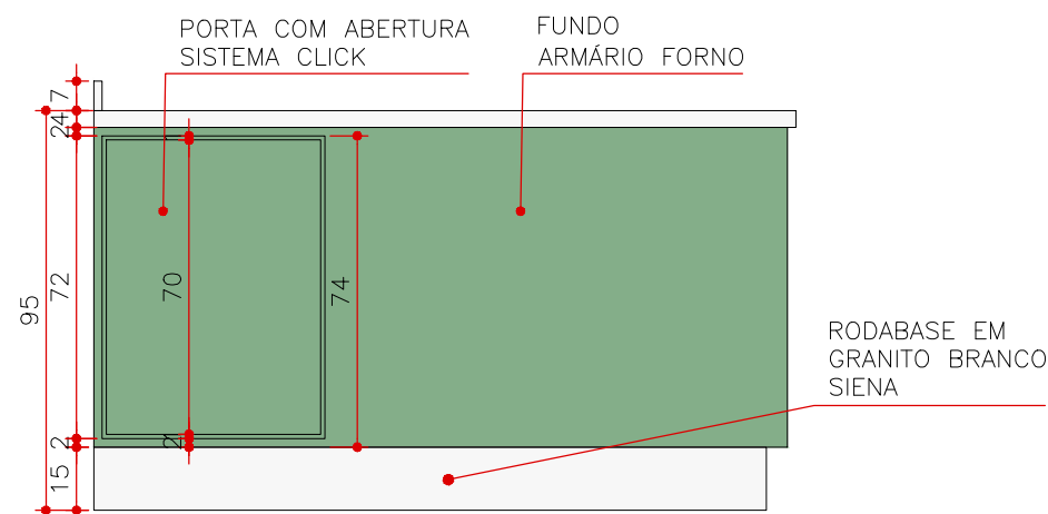
ELEVAÇÃO 4 MA 19 ESCALA 1:20
