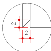
DETALHE PUXADOR CAVA ESCALA 1:5 (MEDIDAS EM CM)
