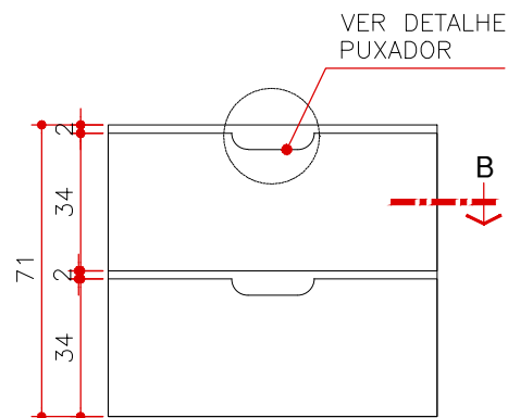
VISTA 1 MA 18 ESCALA 1:20 (MEDIDAS EM CM)
