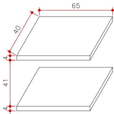
PERSPECTIVA PRAELEIRAS MA 21 ESCALA 1:20
