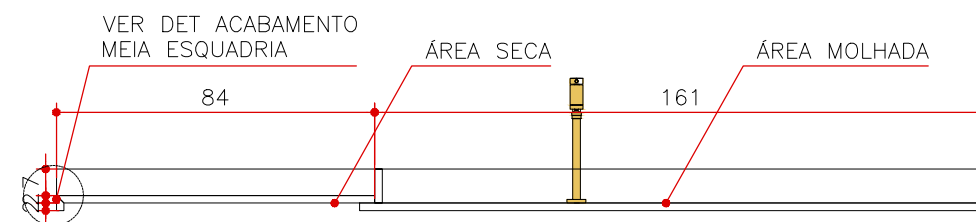
CORTE CC PE 01 ESCALA 1:20
