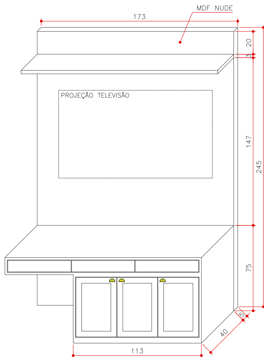
PERSPECTIVA MO 11 ESCALA 1:20 (MEDIDAS EM CM)
