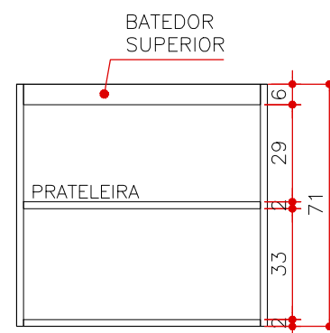
ELEVAÇÃO 1 - S/ PORTA MA 08 ESCALA 1:20
