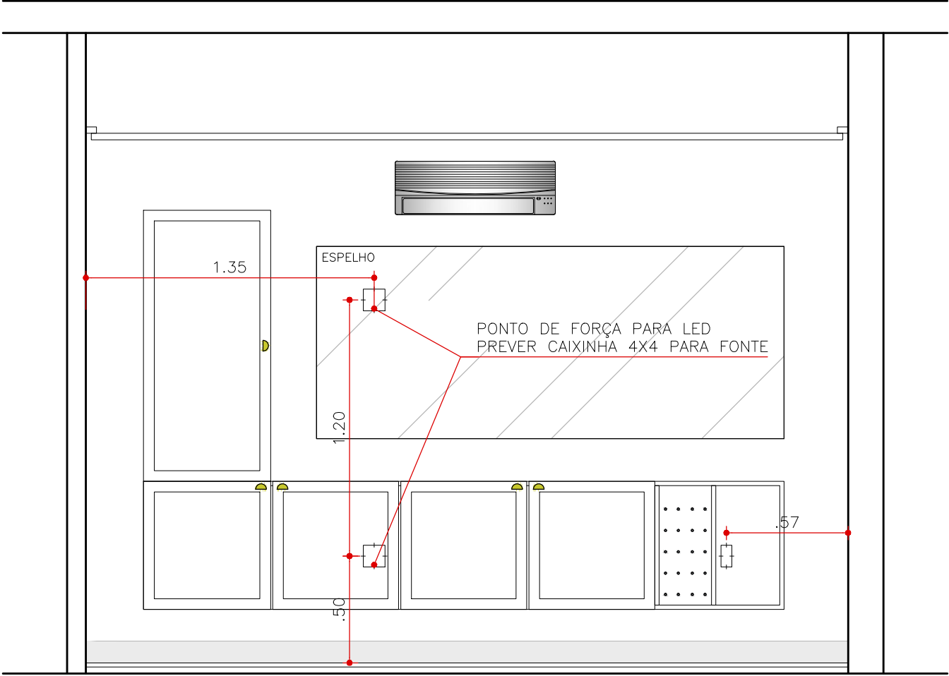
ELEVAÇÃO 3 – ELÉTRICA SALA ESTAR E JANTAR ESCALA 1:25
