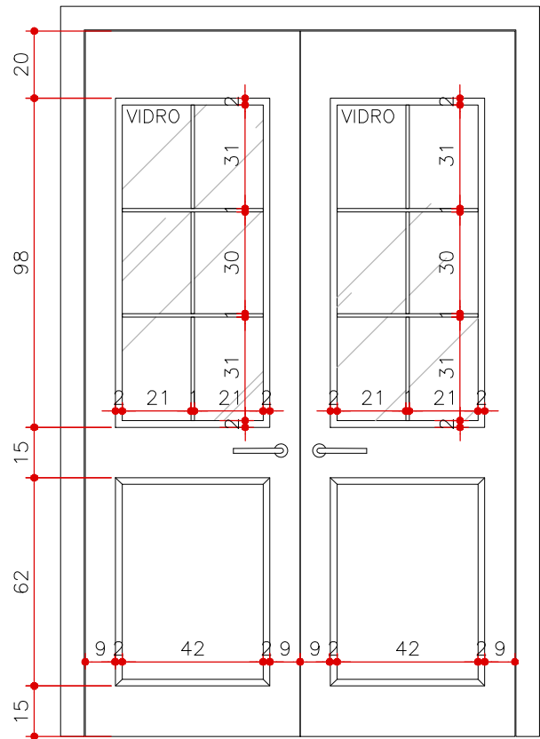
PORTA BALCÃO ESCALA 1:20 (MEDIDAS EM CM)
