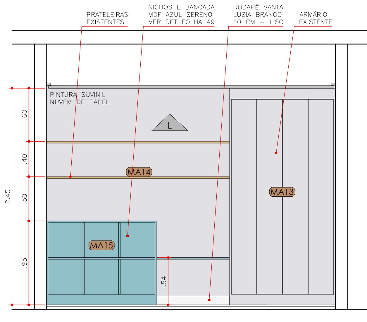
ELEVAÇÃO 28 QUARTO MIGUEL ESCALA 1:25
