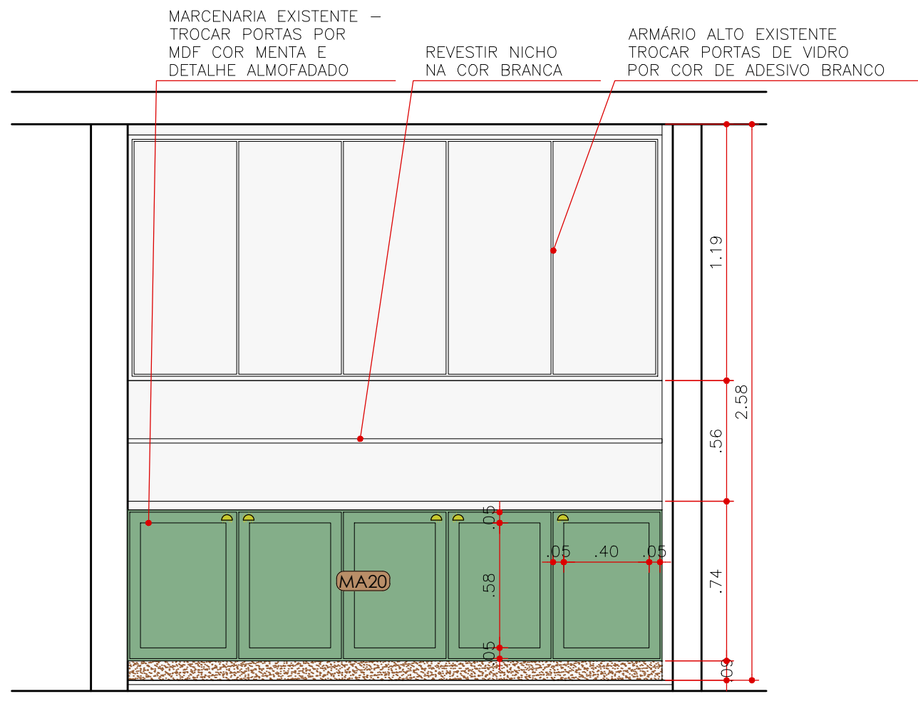
ELEVAÇÃO 10 COZINHA ESCALA 1:25
