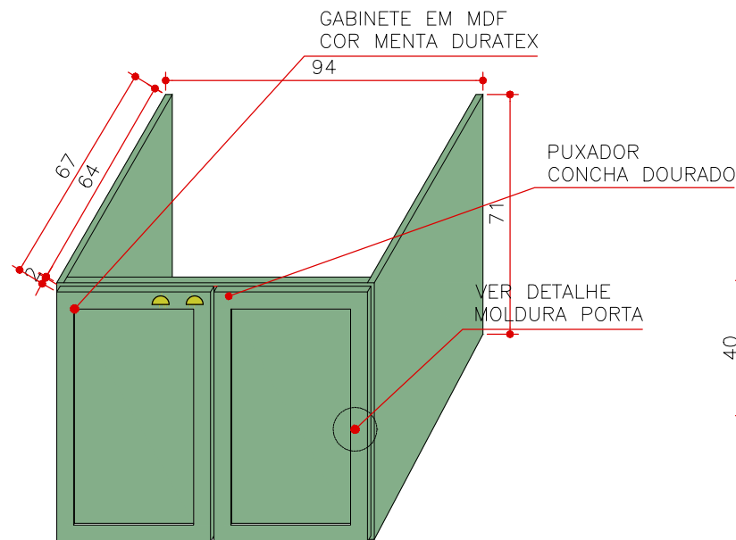
PERSPECTIVA MA 21 ESCALA 1:20
