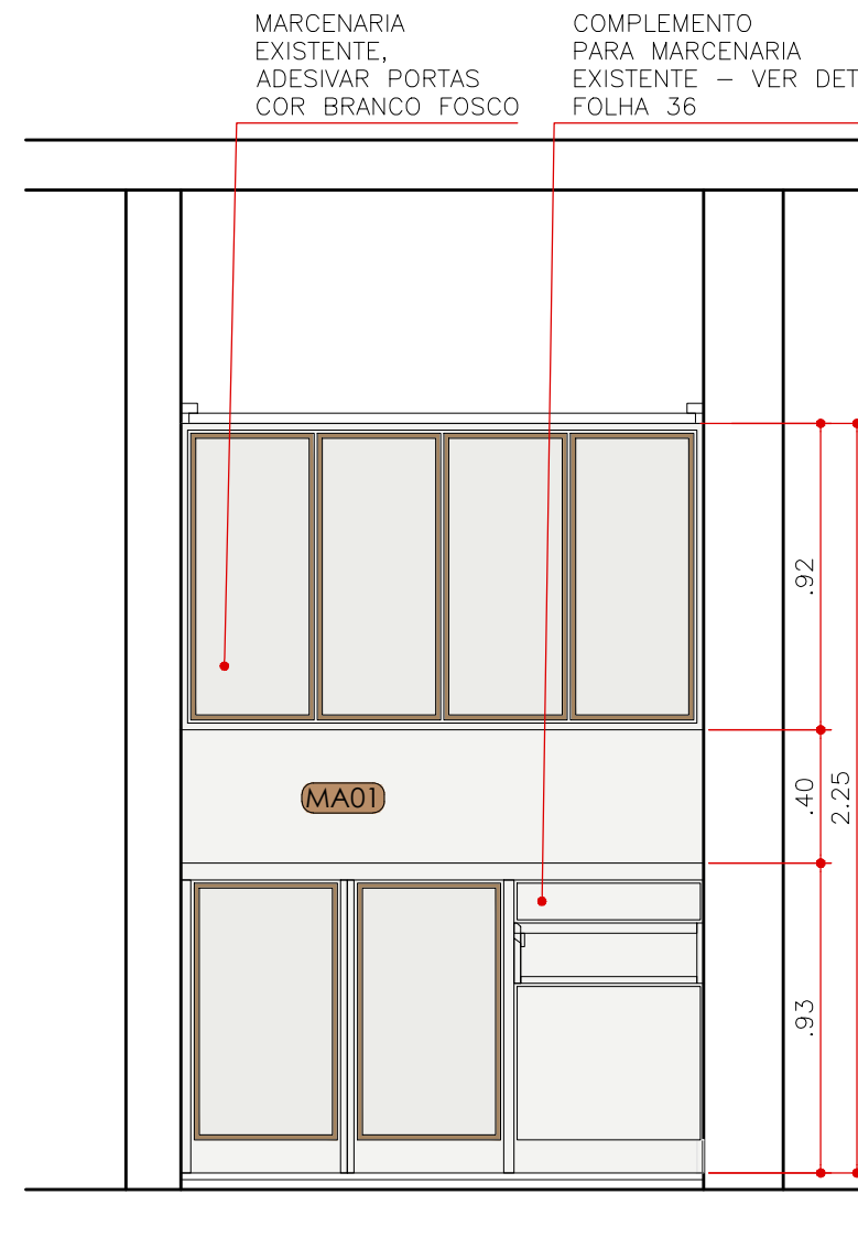
ELEVAÇÃO 6 HALL DE ENTRADA / HOME OFFICE ESCALA 1:25
