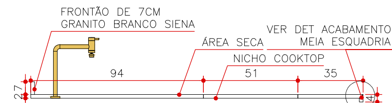
CORTE FF PE 01 ESCALA 1:20
