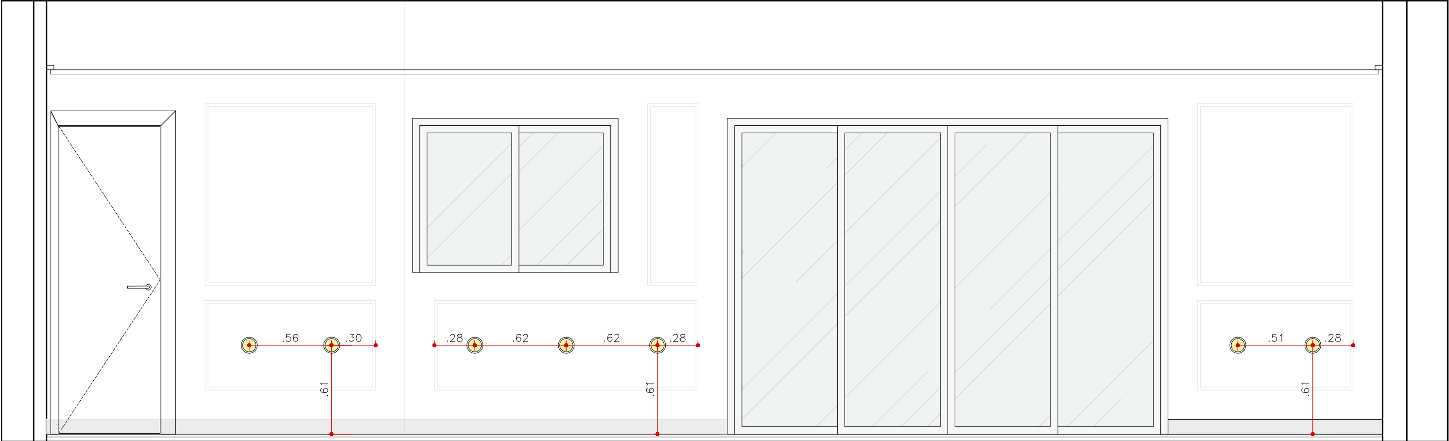
ELEVAÇÃO 2 – ELÉTRICA SALA ESTAR E JANTAR ESCALA 1:25
