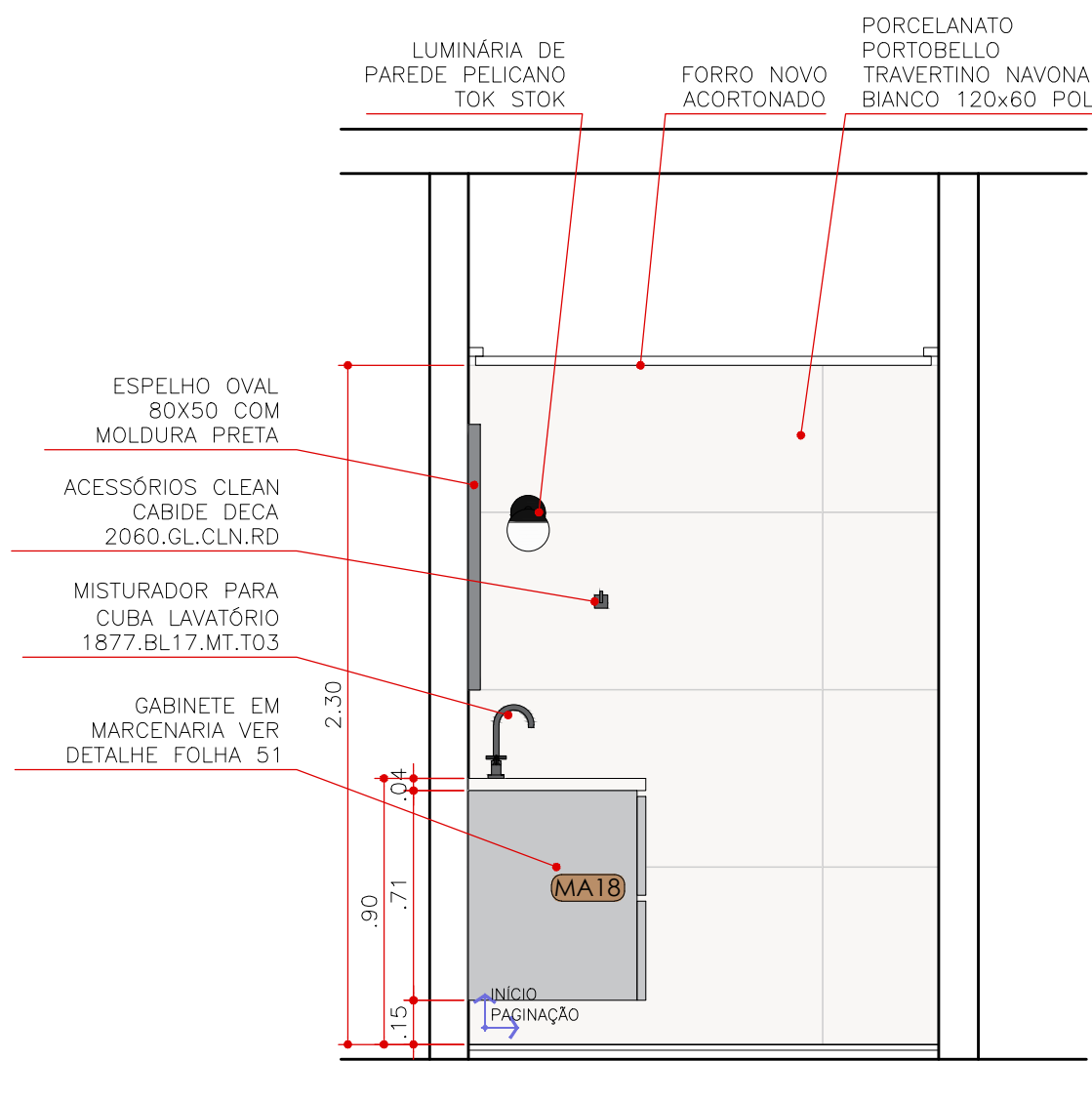
ELEVAÇÃO 37 BANHO MENINOS ESCALA 1:25
