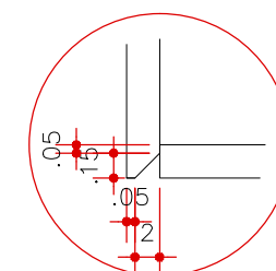
DETALHE PUXADOR CAVA ESCALA 1:5 (MEDIDAS EM CM)
