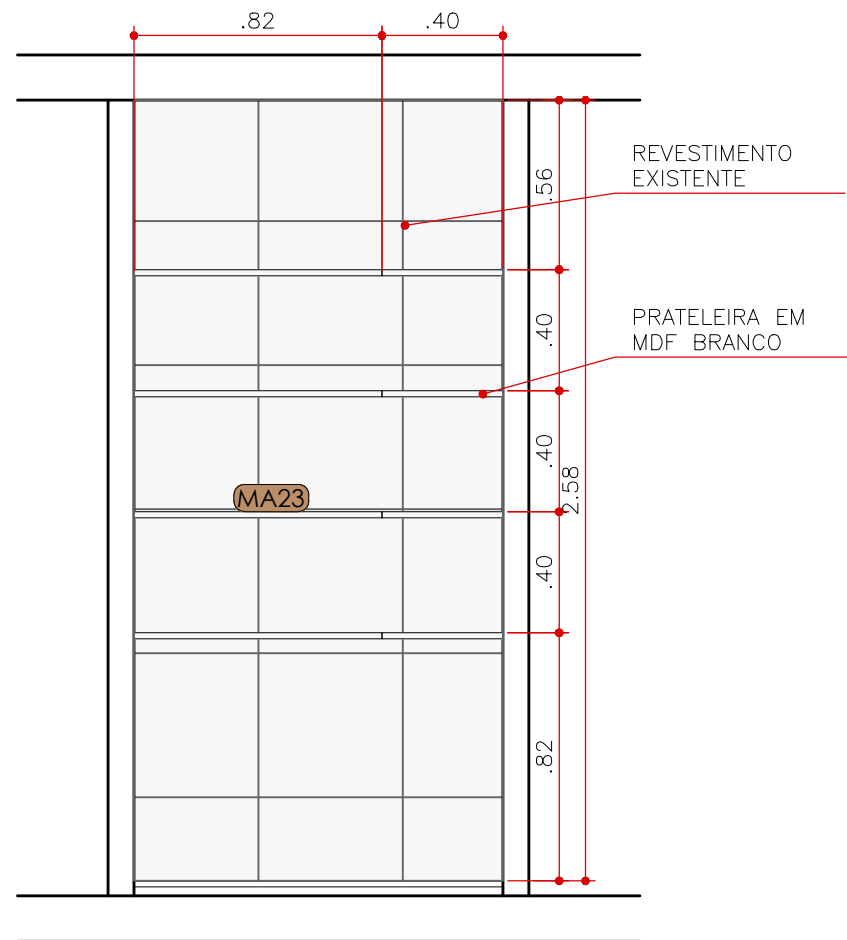
ELEVAÇÃO 14 DESPENSA ESCALA 1:25
