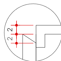
DETALHE PUXADOR CAVA ESCALA 1:5 (MEDIDAS EM CM)
