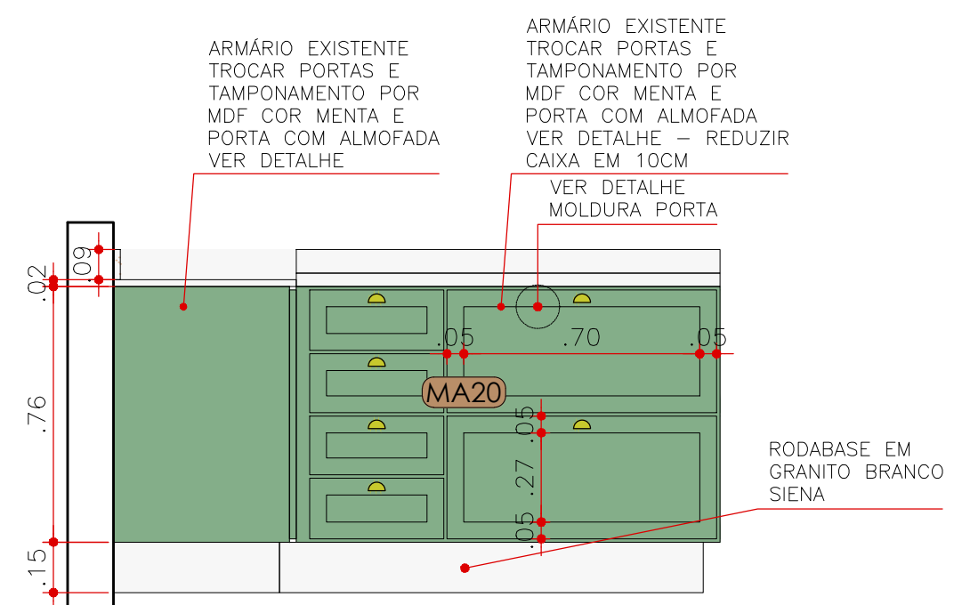
ELEVAÇÃO 2 MA 19 ESCALA 1:20
