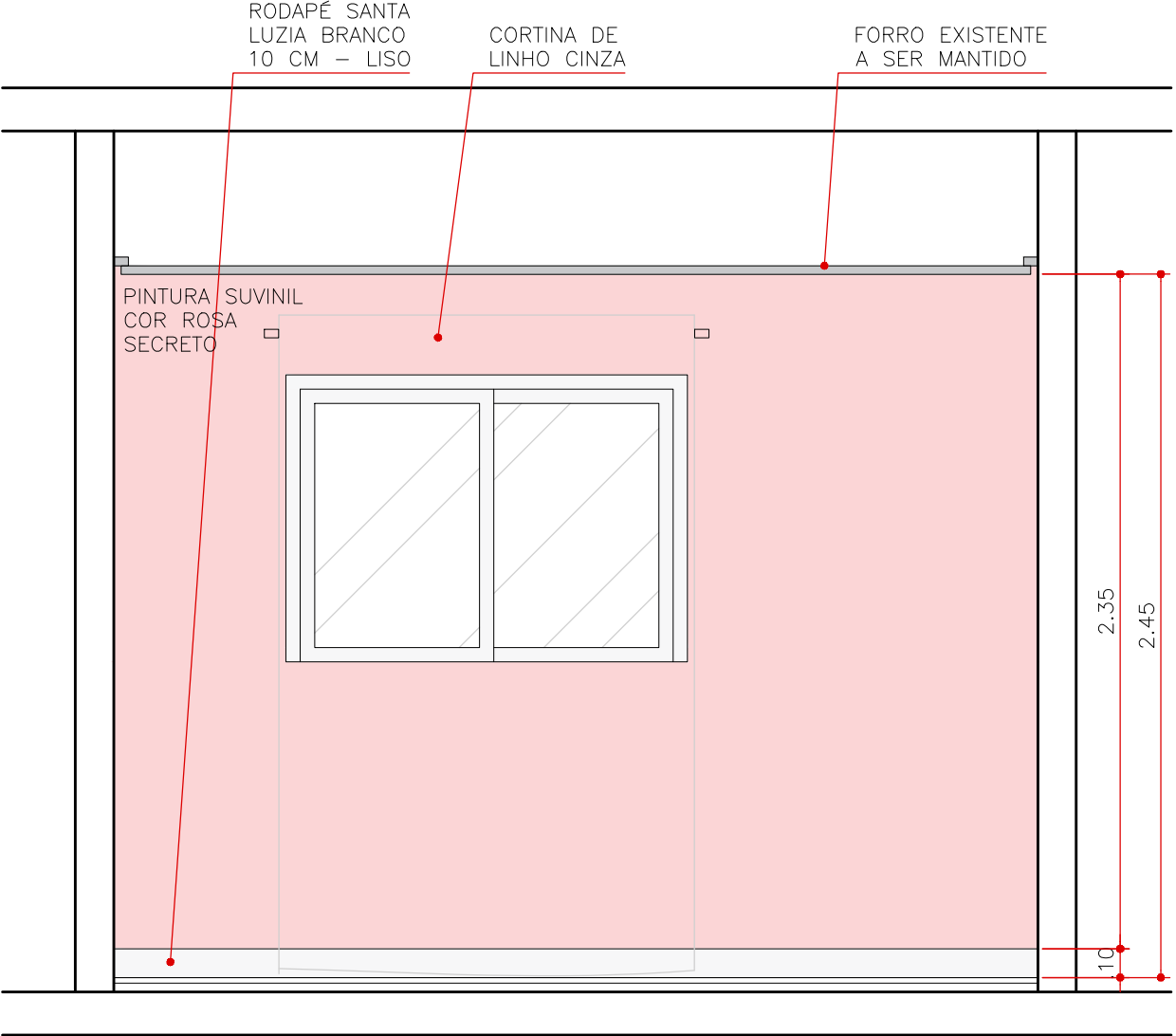
ELEVAÇÃO 20 QUARTO CASAL ESCALA 1:25
