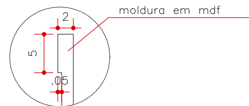
DETALHE MOLDURA PORTA ESCALA 1:5 (MEDIDAS EM CM)
