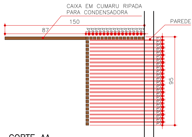
CORTE AA MA 09 ESCALA 1:20
