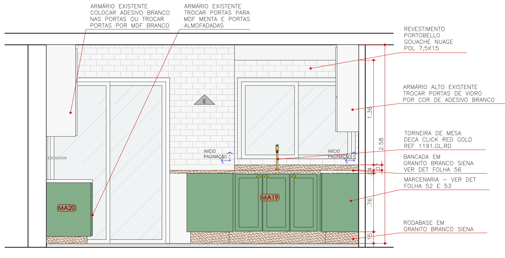
ELEVAÇÃO 9 COZINHA ESCALA 1:25
