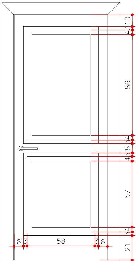
PORTA SALA ESCALA 1:20 (MEDIDAS EM CM)
