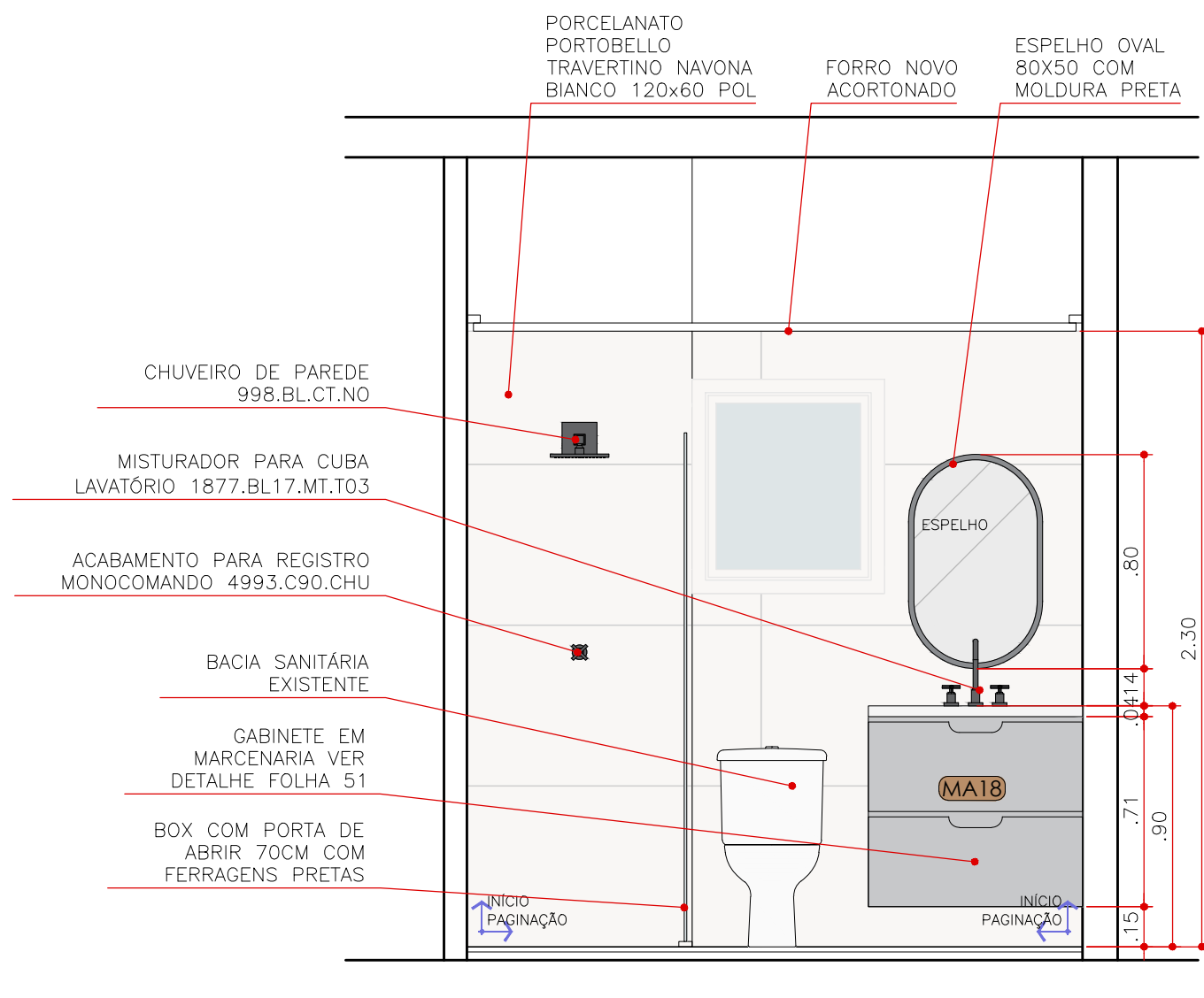
ELEVAÇÃO 36 BANHO MENINOS ESCALA 1:25
