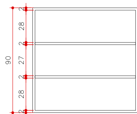
VISTA 1 SEM PORTA MA 10 ESCALA 1:20 (MEDIDAS EM CM)
