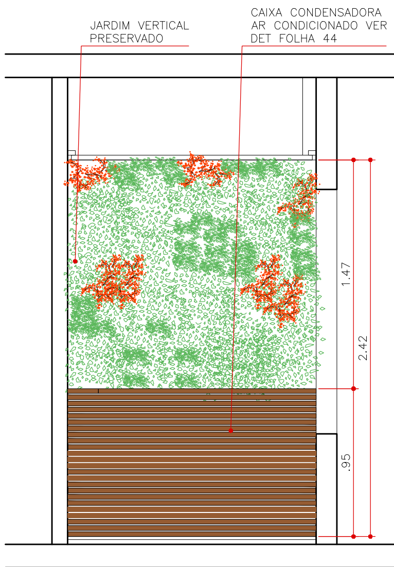
ELEVAÇÃO 17 VARANDA ESCALA 1:25
