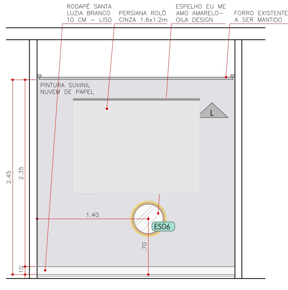
ELEVAÇÃO 29 QUARTO MIGUEL ESCALA 1:25
