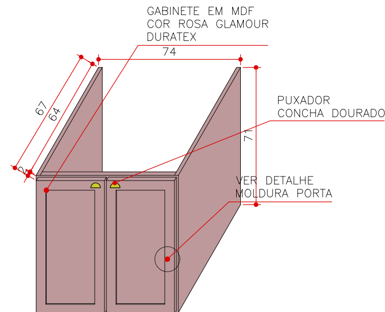
PERSPECTIVA MA 08 ESCALA 1:20
