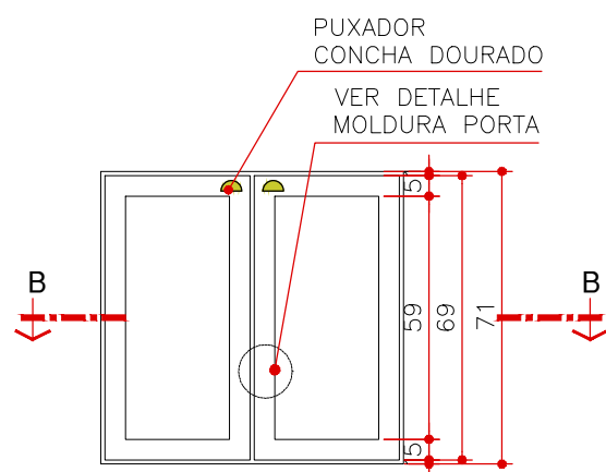
ELEVAÇÃO 1 MA 08 ESCALA 1:20
