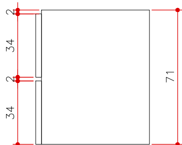
VISTA 2 MA 18 ESCALA 1:20 (MEDIDAS EM CM)
