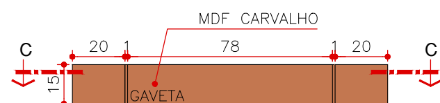
ELEVAÇÃO 1 MA 04 ESCALA 1:20
