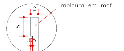
DETALHE MOLDURA PORTA ESCALA 1:5 (MEDIDAS EM CM)
