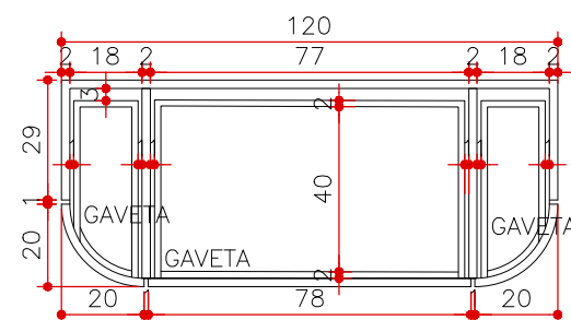
CORTE CC MA 04 ESCALA 1:20
