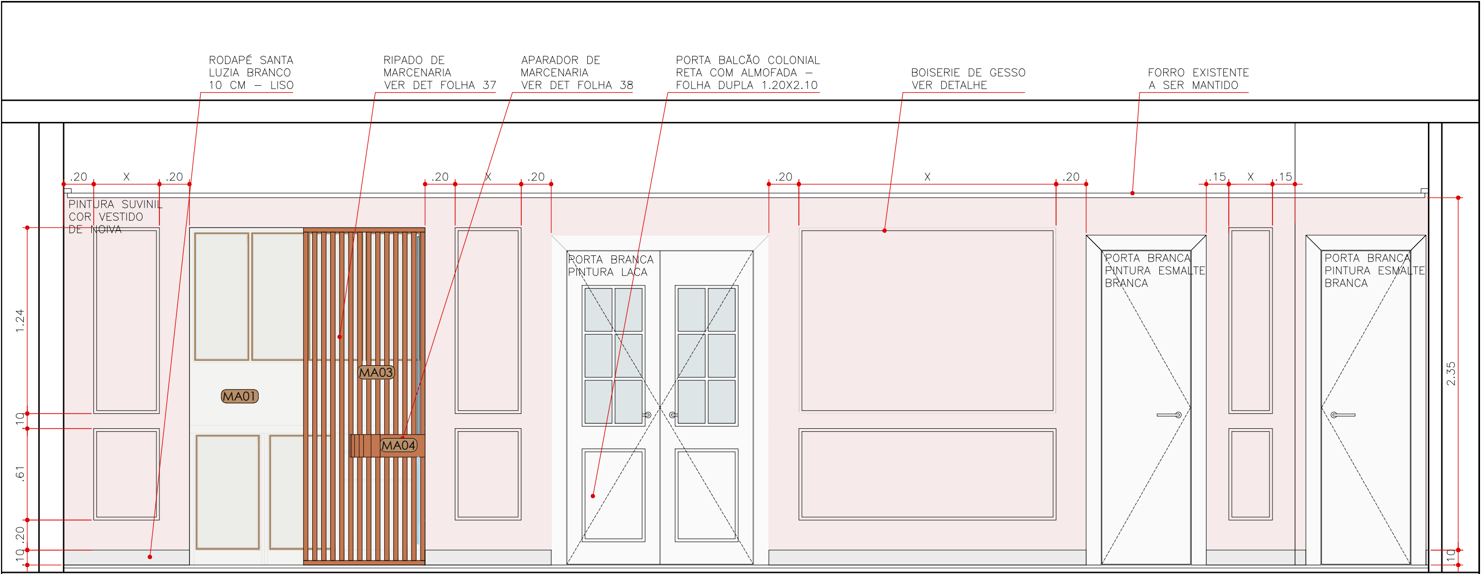
ELEVÇÃO 4 SALA ÉSTAR E JANTAR ESCALA 1:25
