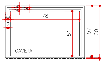
CORTE B MA 10 ESCALA 1:20 (MEDIDAS EM CM)
