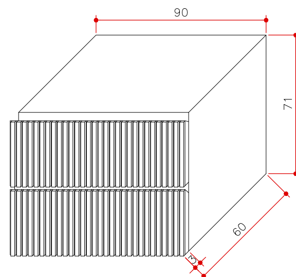
PERSPECTIVA MO 10 ESCALA 1:20 (MEDIDAS EM CM)
