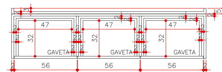
CORTE B MA 11 ESCALA 1:20 (MEDIDAS EM CM)
