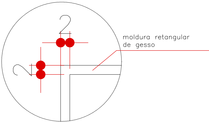
DETALHE BOISERIE ESCALA 1:5 (MEDIDAS EM CM)
