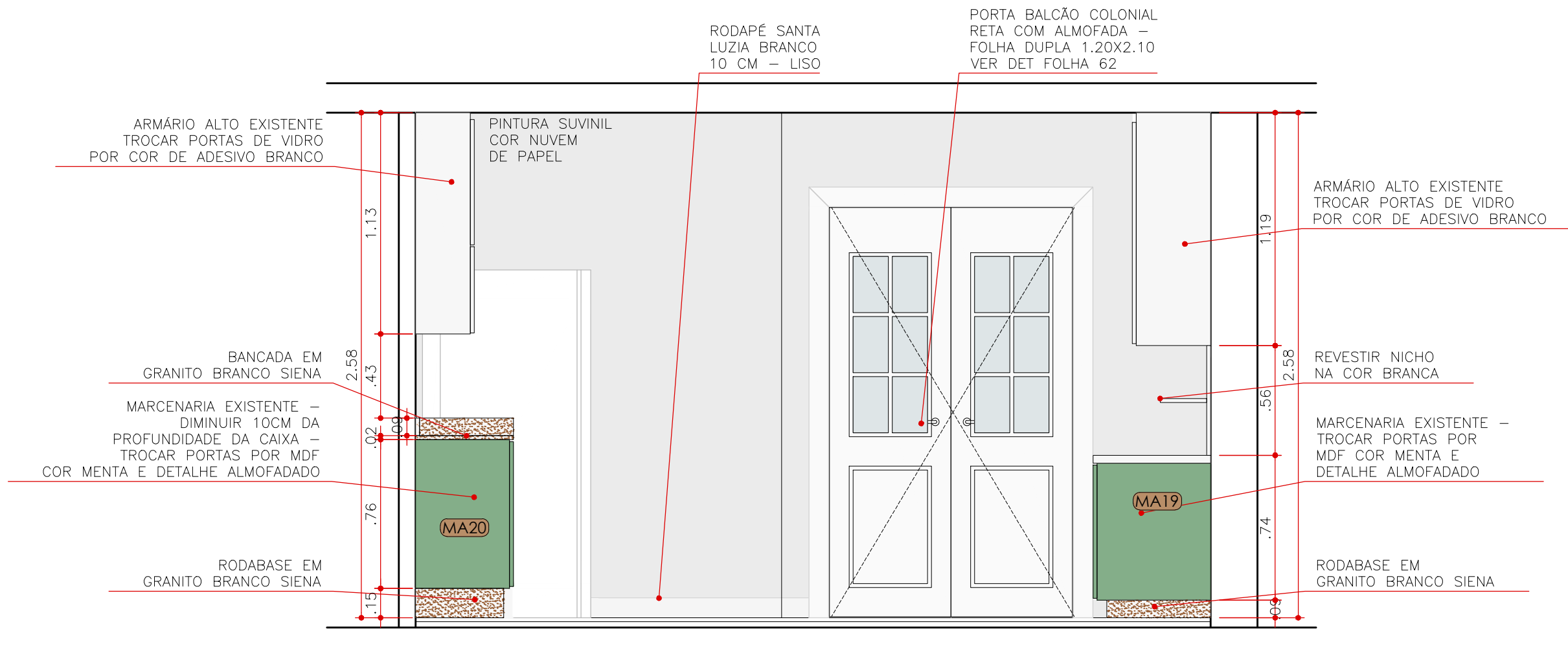
ELEVAÇÃO 11 COZINHA ESCALA 1:25
