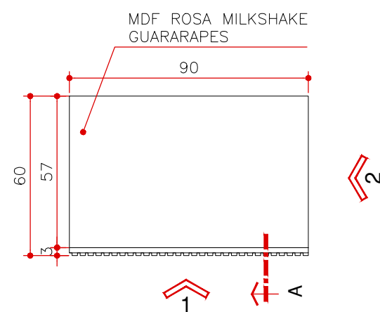
PLANTA MA 10 ESCALA 1:20 (MEDIDAS EM CM)
