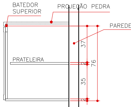
CORTE AA MA 21 ESCALA 1:20
