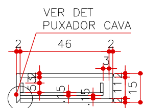
CORTE AA MA 04 ESCALA 1:20
