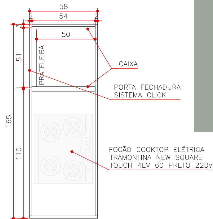
PLANTA MA 19 ESCALA 1:20
