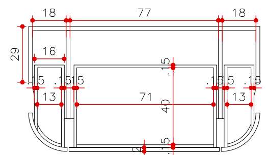
CORTE CC MA 04 ESCALA 1:20
