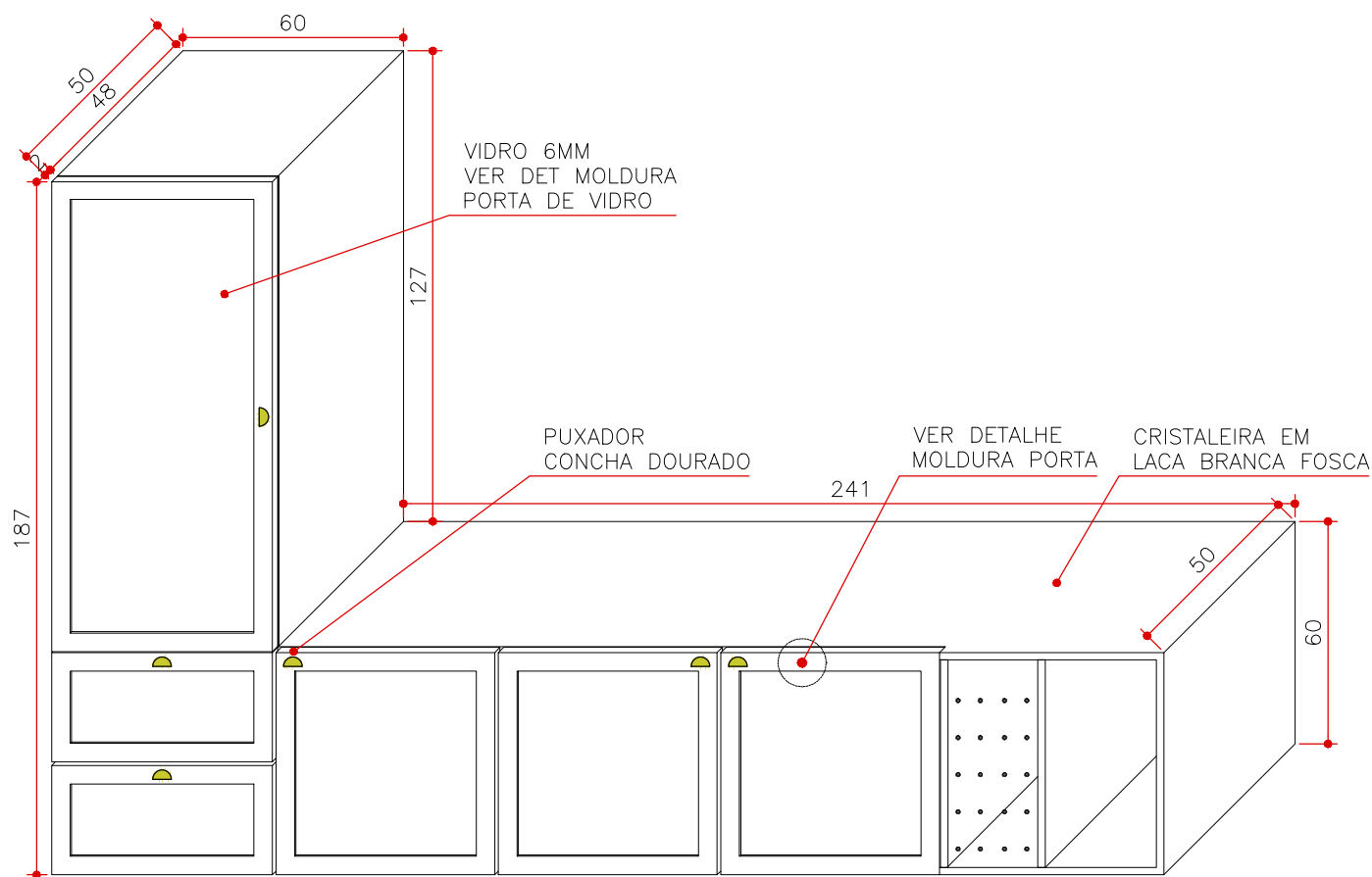
PERSPECTIVA MA 05 ESCALA 1:20 (MEDIDAS EM CM)
