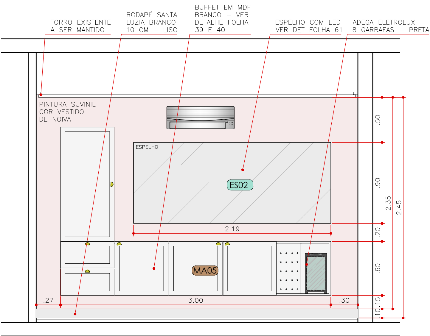
ELEVAÇÃO 3 SALA ESTAR E JANTAR ESCALA 1:25
