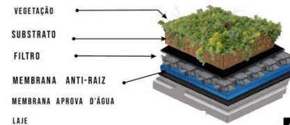
COBERTURA TELHADO VERDE
