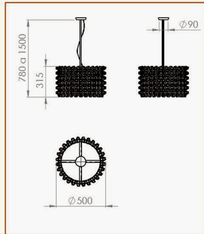
Luminária pendente
