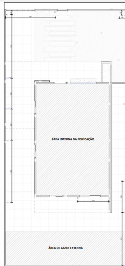
PLANTA DE PONTOS ELÉTRICOS - PRIMEIRO PAVIMENTO ESCALA 1:30
