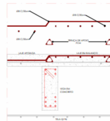
DET. DA ARMADURA EM BALANÇOS DE LAJE ESCALA 1:10
