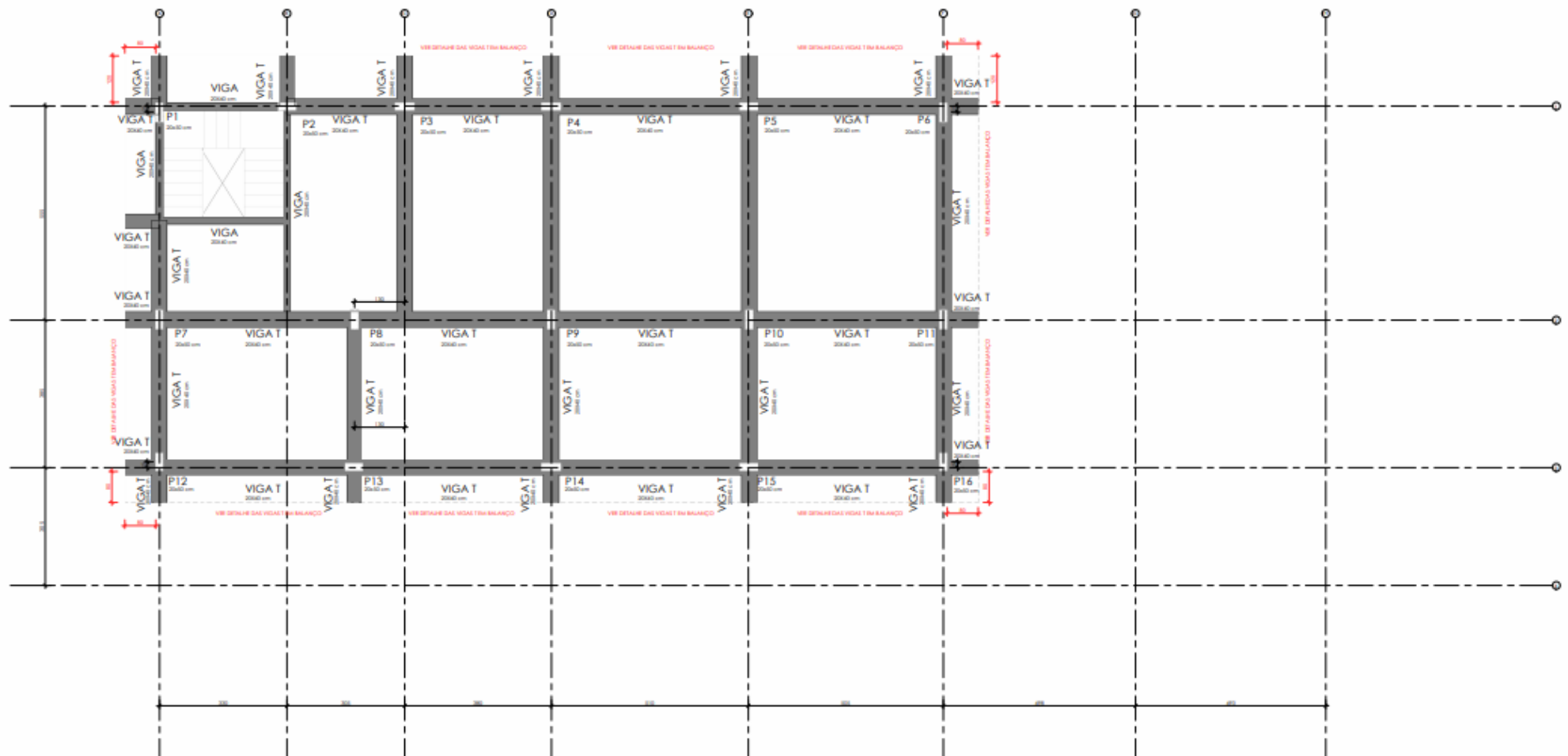
VIGAS - COBERTURA ESCALA 1:50
