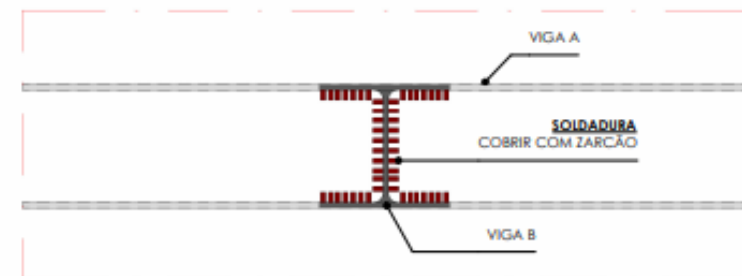
DET.04 ESCALA 1 : 10
