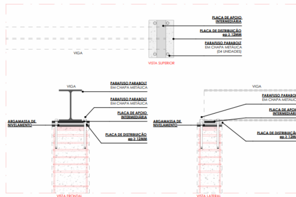
DET.06 ESCALA 1:10
