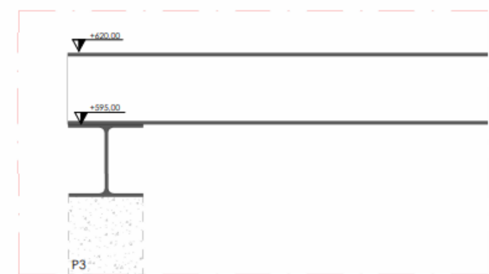
DET.03 ESCALA 1 : 10
