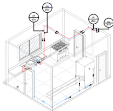
ISOMETRIA 2 ESCALA
