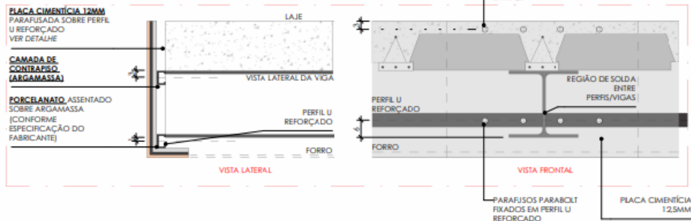
DET.01 ESCALA 1 : 10
