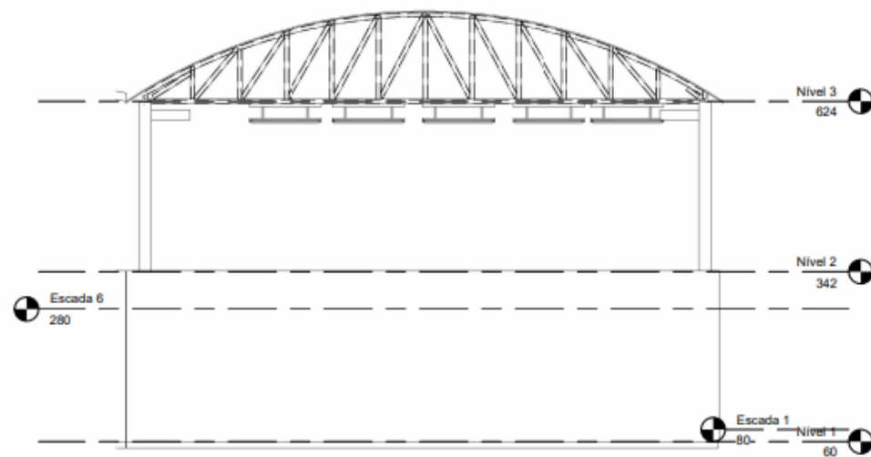
④ Frente Trelça 1 : 50
