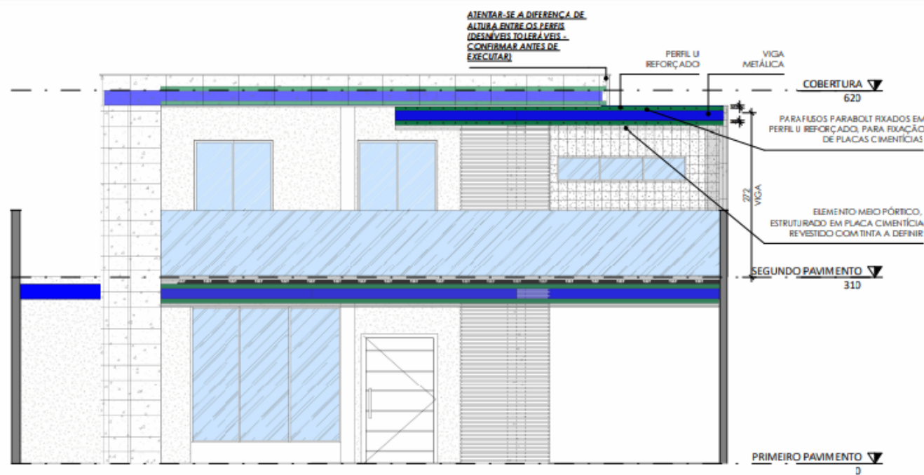
DET FACHADA - VISTA FRONTAL DOS PERFIS U ESCALA 1 : 50
