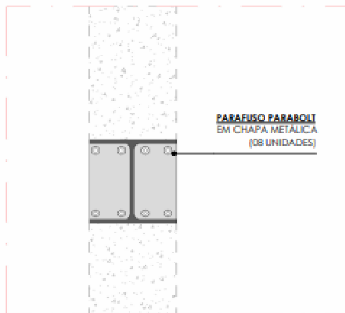
DET.05 ESCALA 1:10
