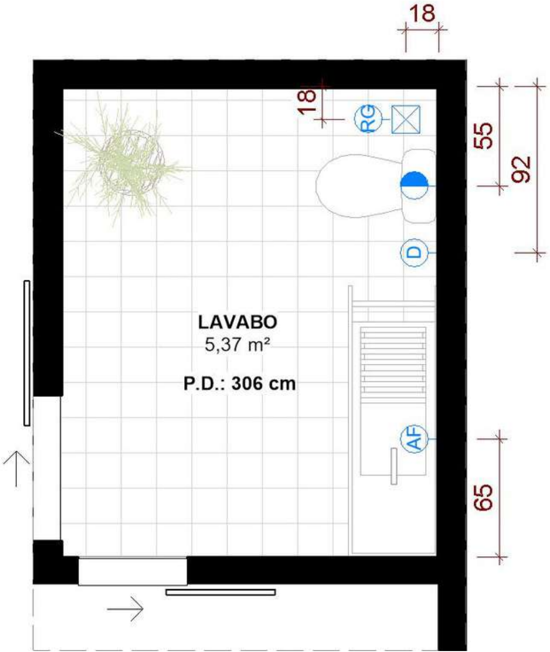
Planta de Hidráulica Lavabo (Executivo)
