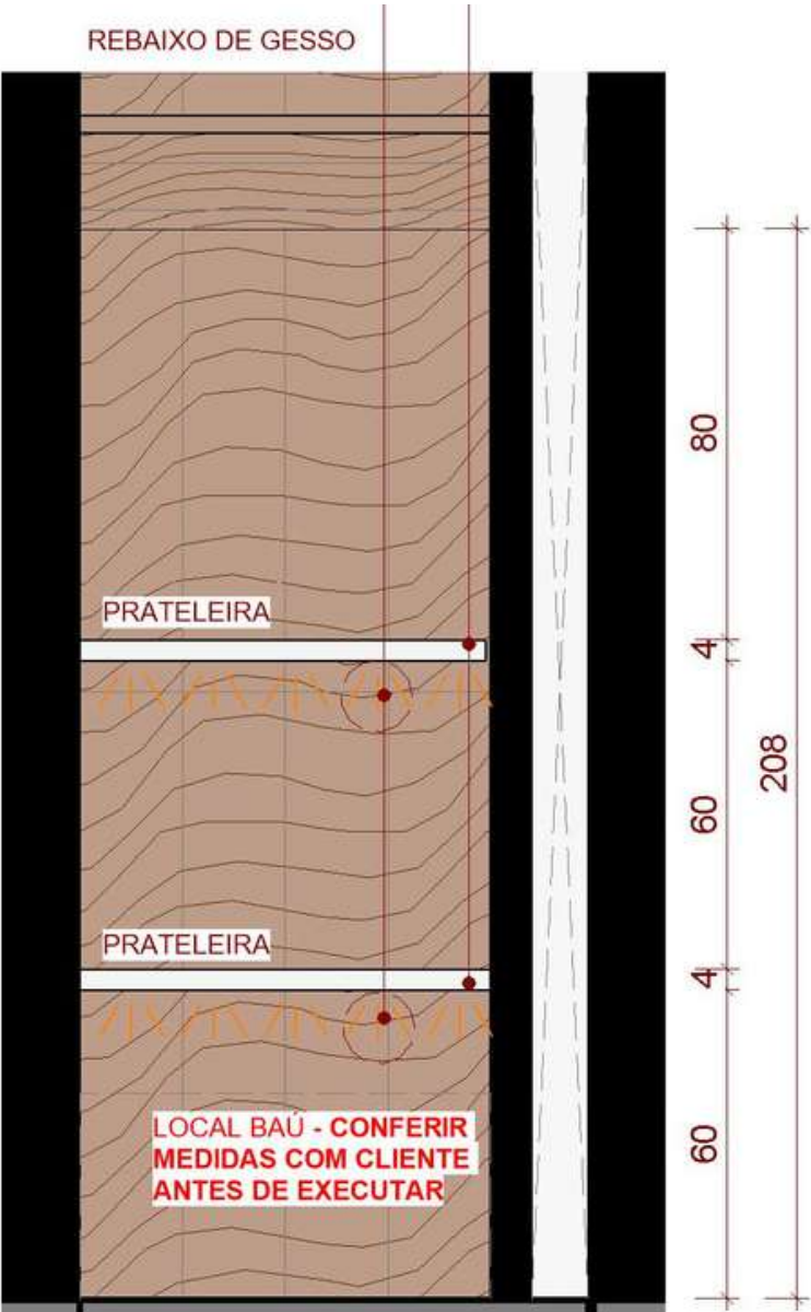
Vista Hall (det. de marcenaria)
