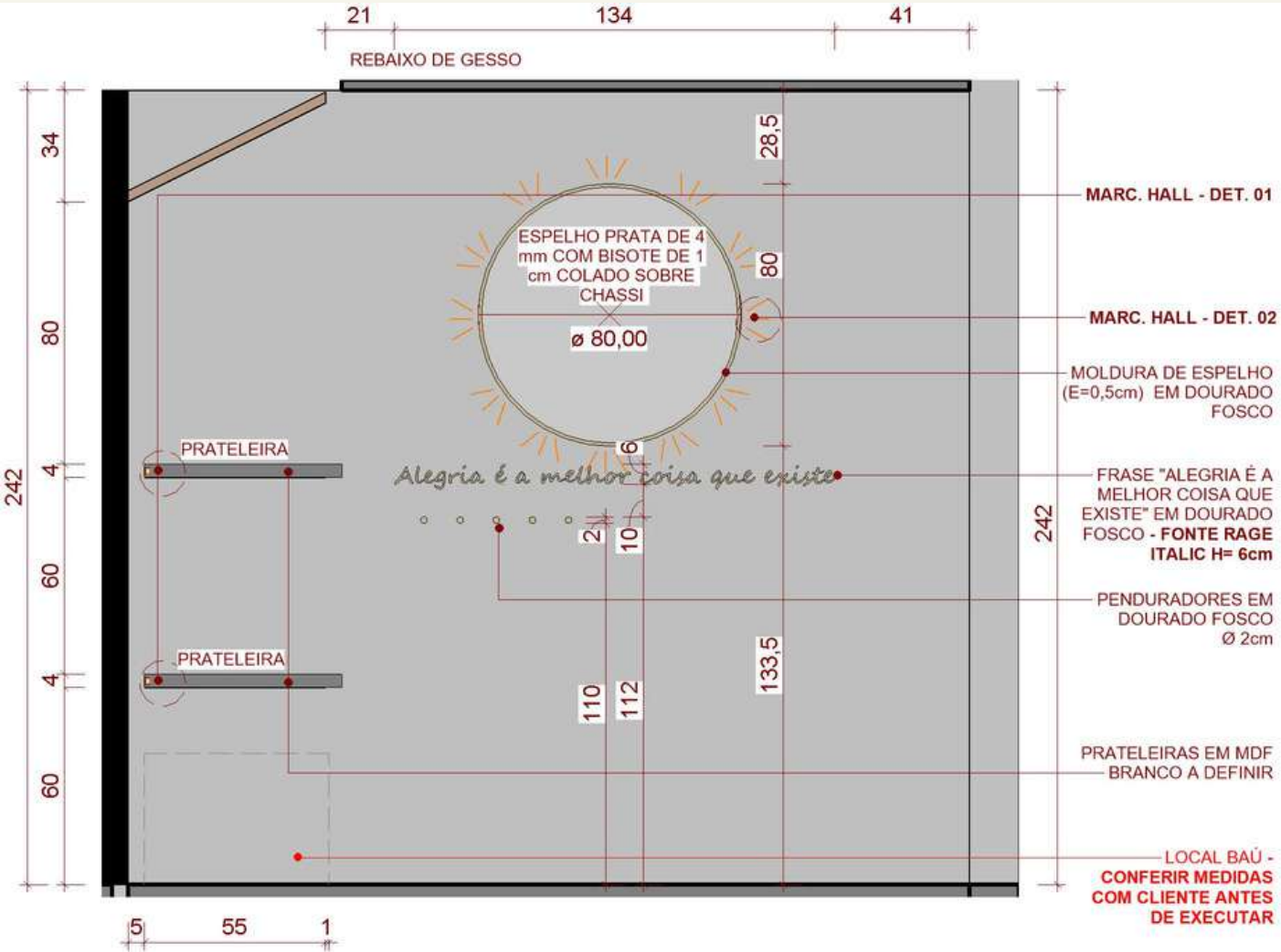
Vista Hall (det. de marcenaria)
