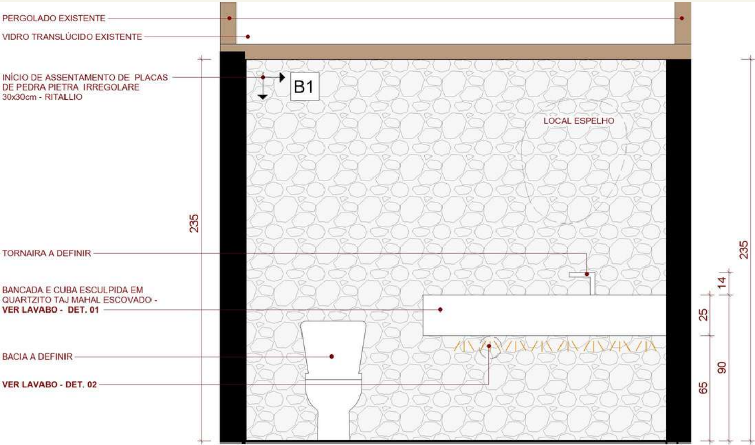
Vista Lavabo (Detalhamento)
