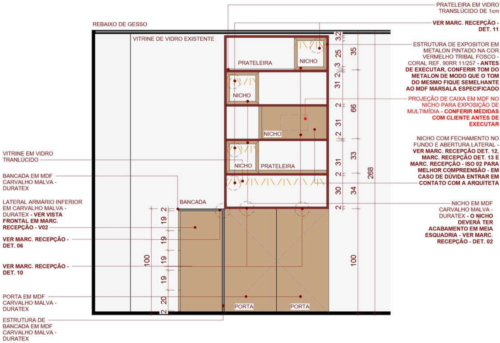
Vista (det. de marcenaria)
