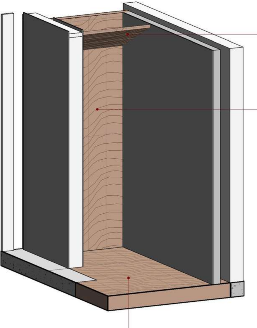
Isométrica Hall (Detalhamento) - Modelagem no Revit
