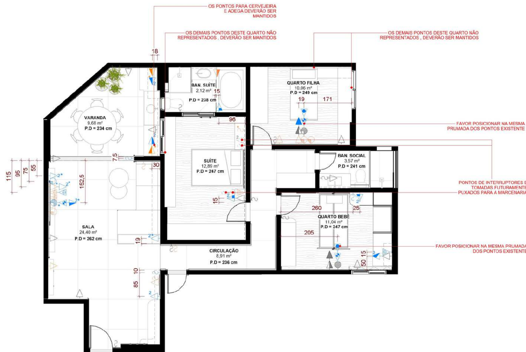
Planta de Forro e Iluminação (Executivo)
