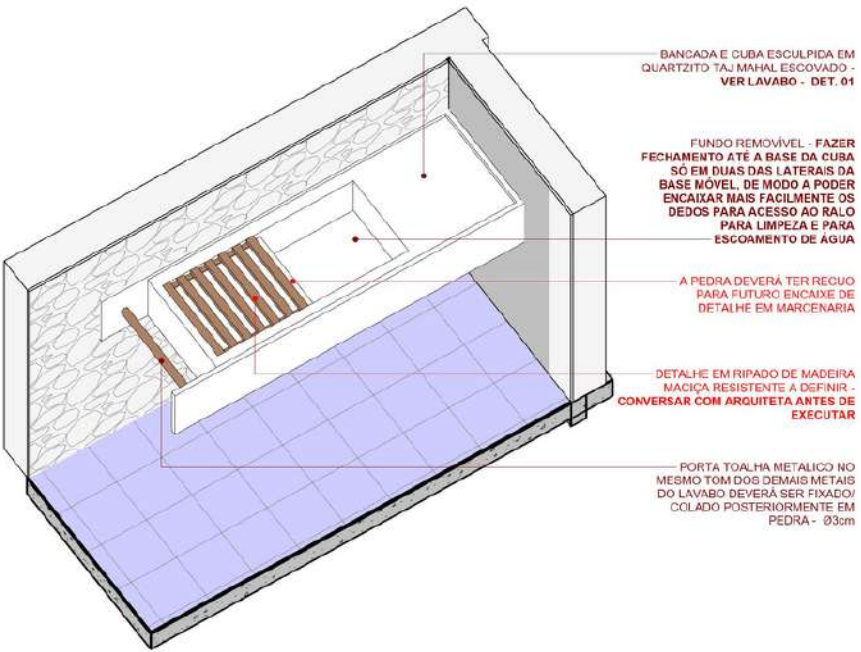
Isométrica Lavabo (Detalhamento) - Modelagem no Revit
