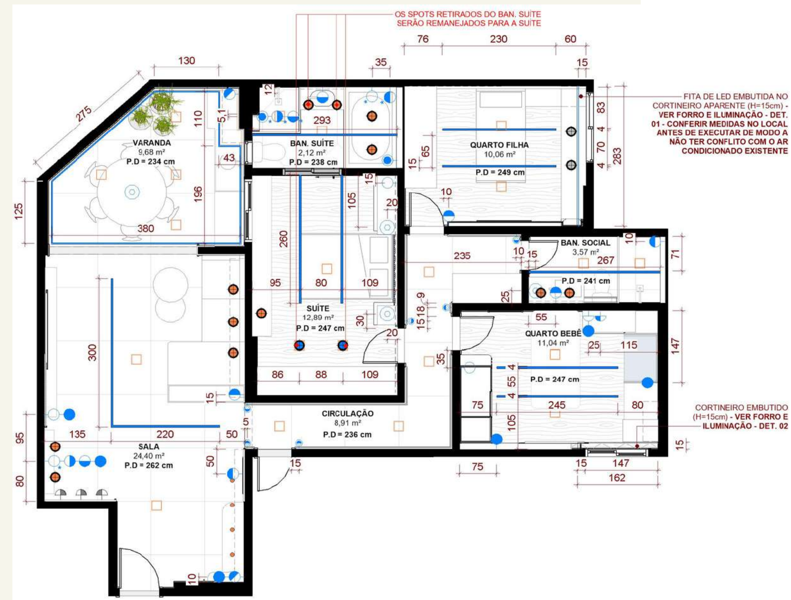
Planta de Elétrica (Executivo)
