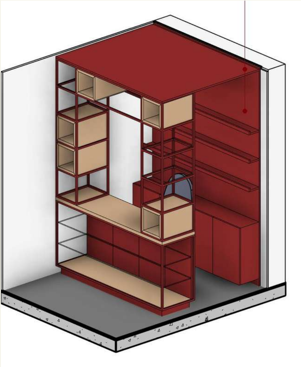
Isométrica (det. de marcenaria) - Modelagem no Revit
