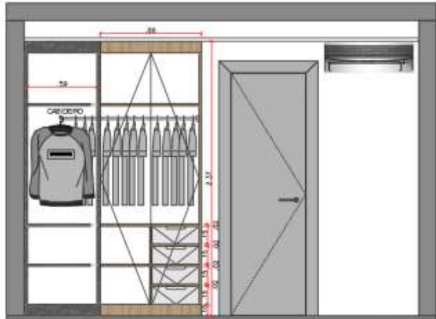
ELEVAÇÃO 01 esc 1:25
