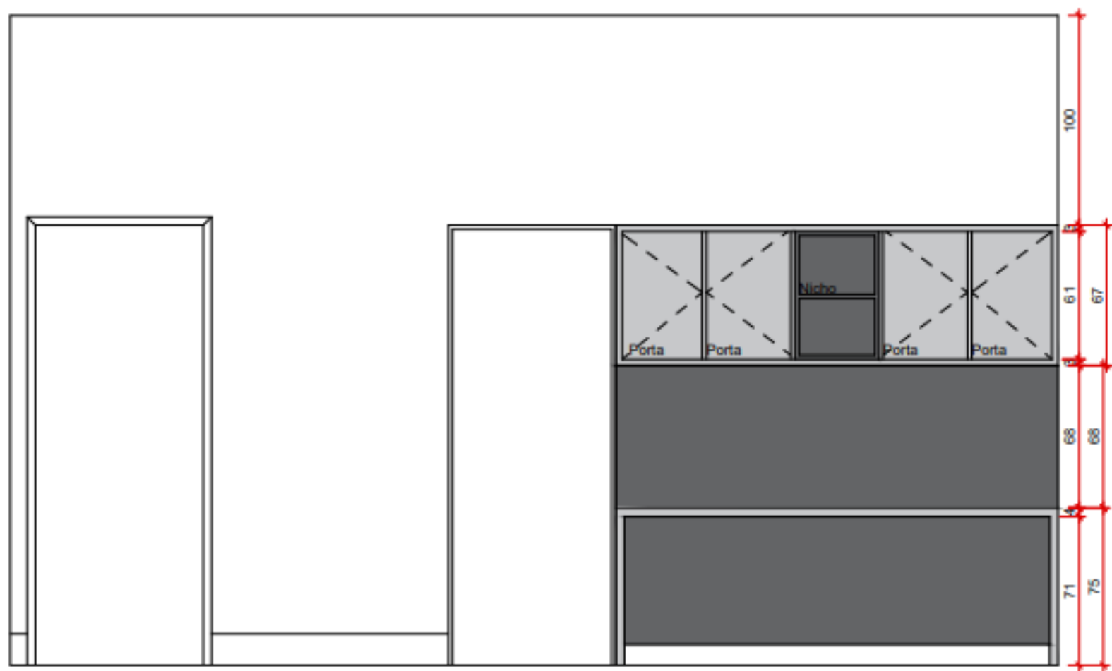
Suite Gustavo -Vista C (Aberto) Escala.: 1/25
