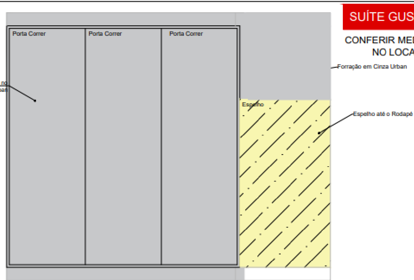
Suite Gustavo -Vista A (Aberto) Escala.: 1/25
