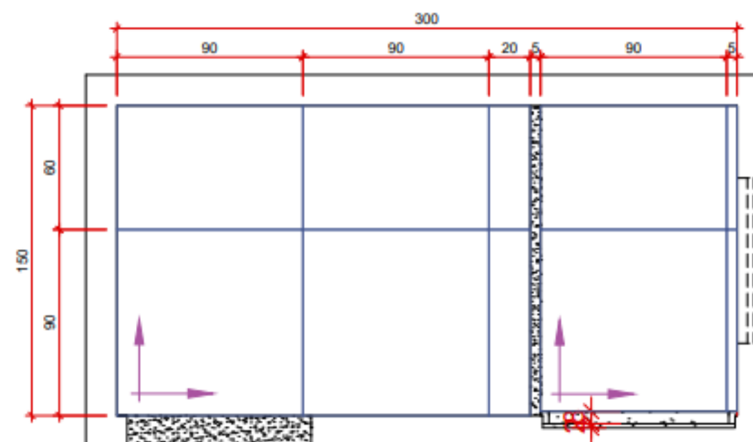
Paginação de Banho Gustavo Escala.: 1/25
