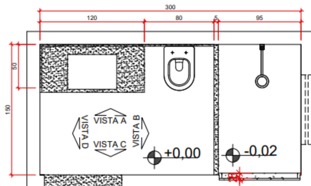
Planta Baixa Banho Gustavo Escala.: 1/25
