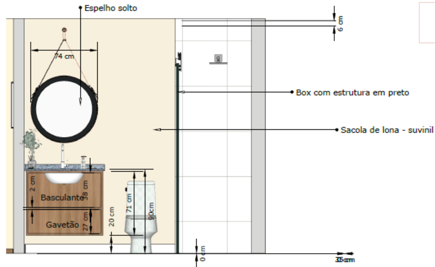
17 Vista E (Aberto) Esc: 1/25
