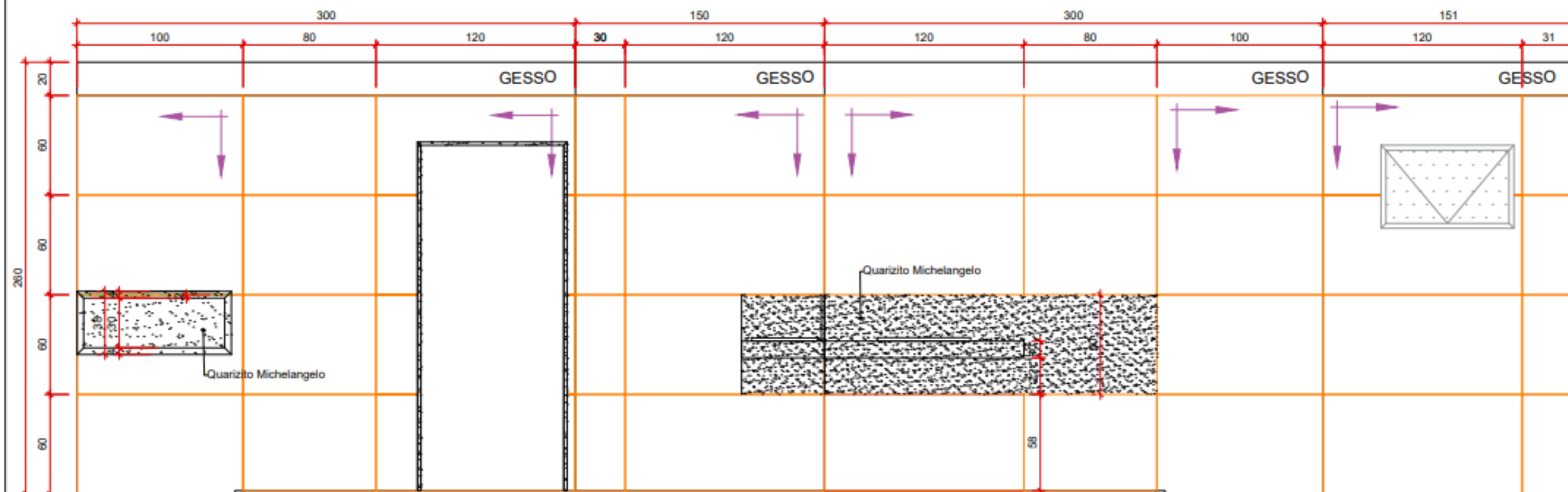
Vista D Escala.: 1/25
