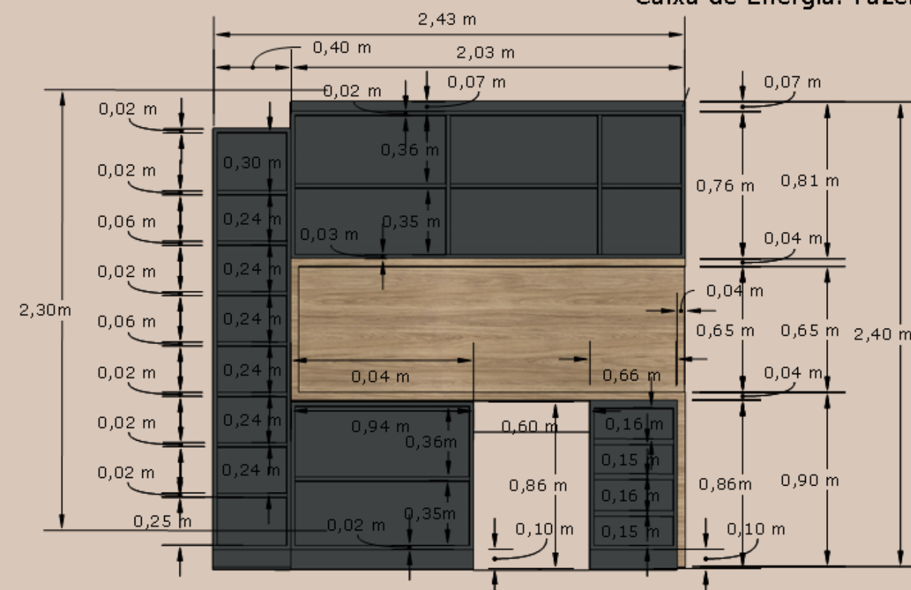
Vista B - Armário em Marcenaria (Aberto) Escala 1:25
