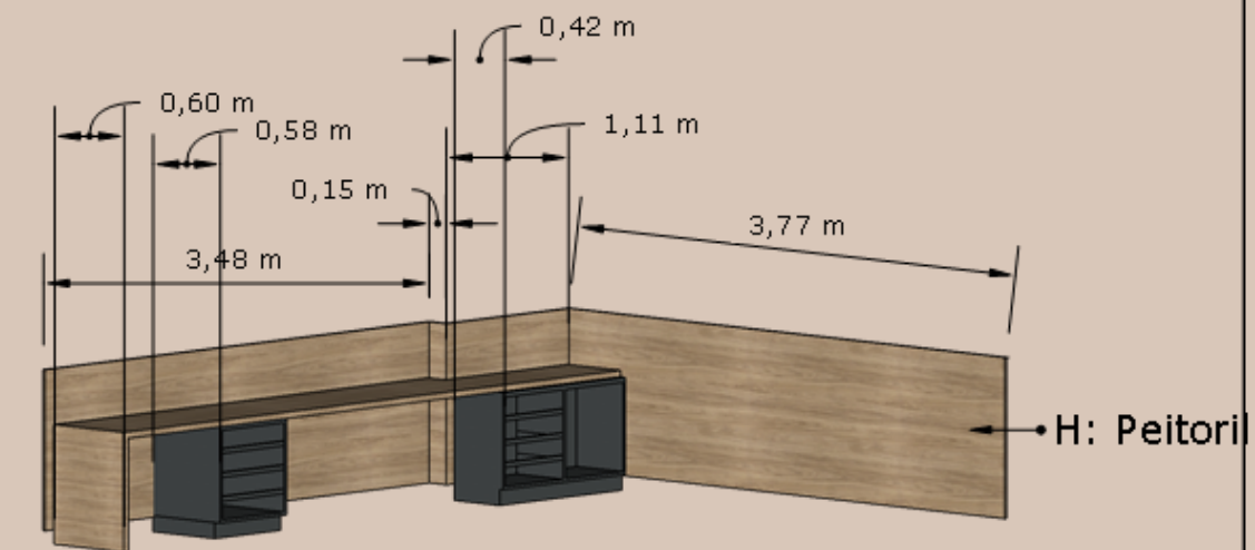
Perspectiva Vista B - Mesa de Trabalho Escala 1:50
