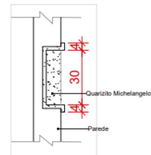
Det. Corte Nicho
