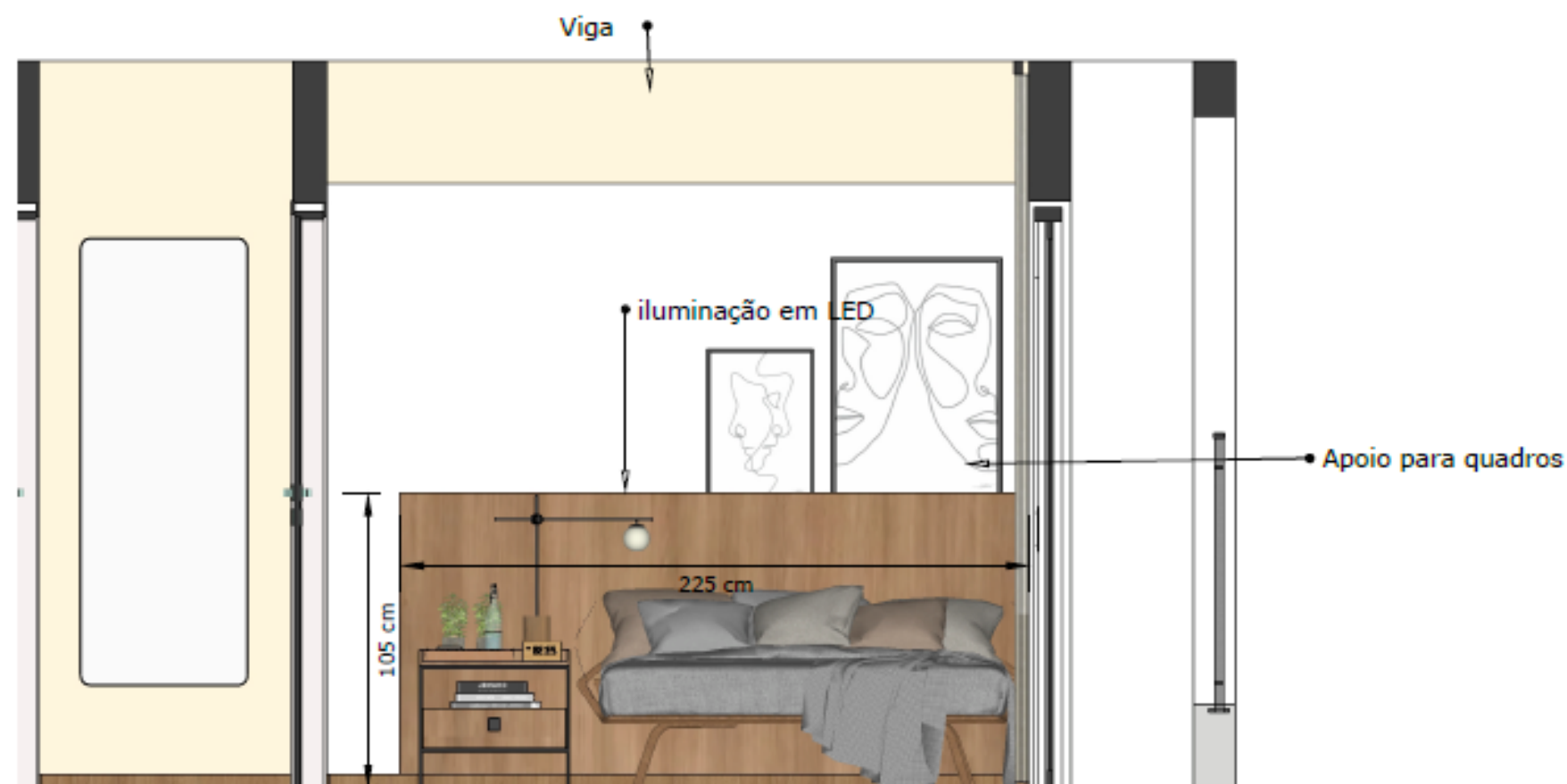
15 Vista G Esc: 1/25
