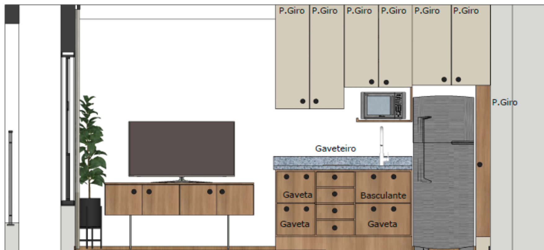
06 Vista A Esc: 1/25
