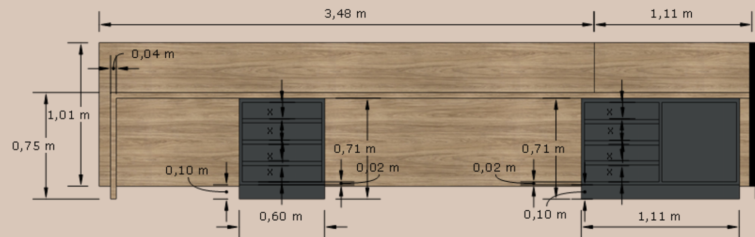
Perspectiva Vista B - Mesa de Trabalho Escala 1:25
