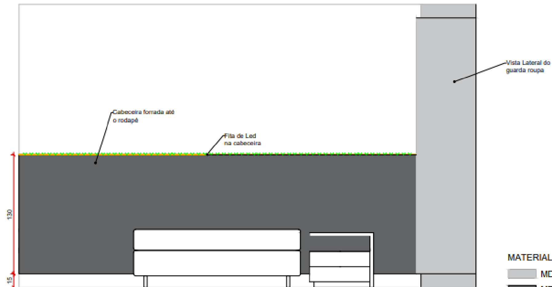
Suite Gustavo -Vista B Escala.: 1/25
