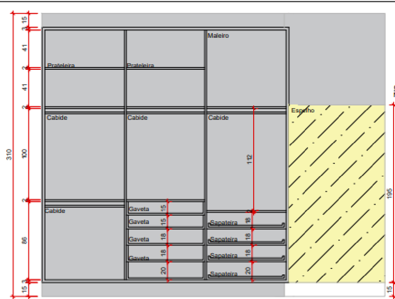
Suite Gustavo -Vista A (Aberto) Escala.: 1/25
