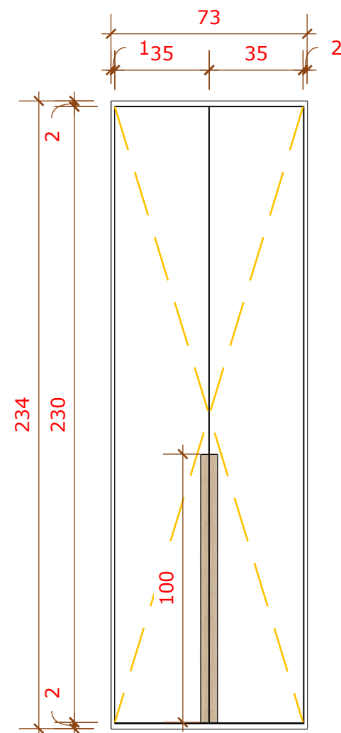
05 VISTA FRONTAL ARM. MULTIUSO 1/20
