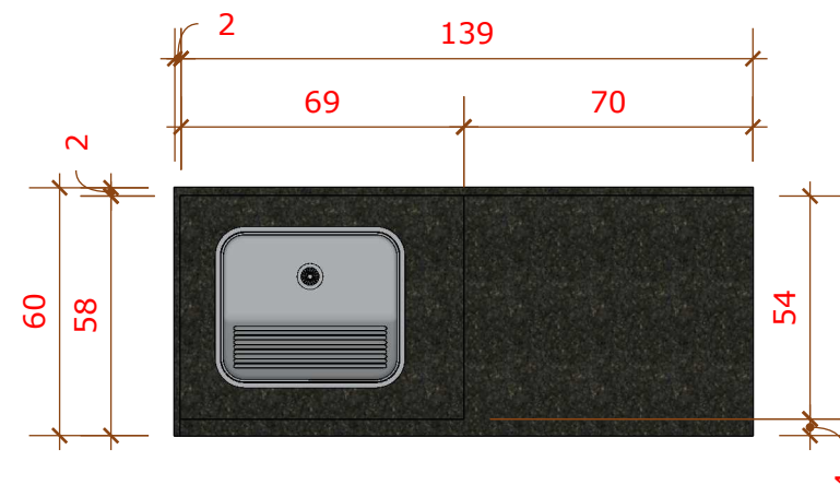
03 VISTA SUPERIOR BANCADA 1/20
