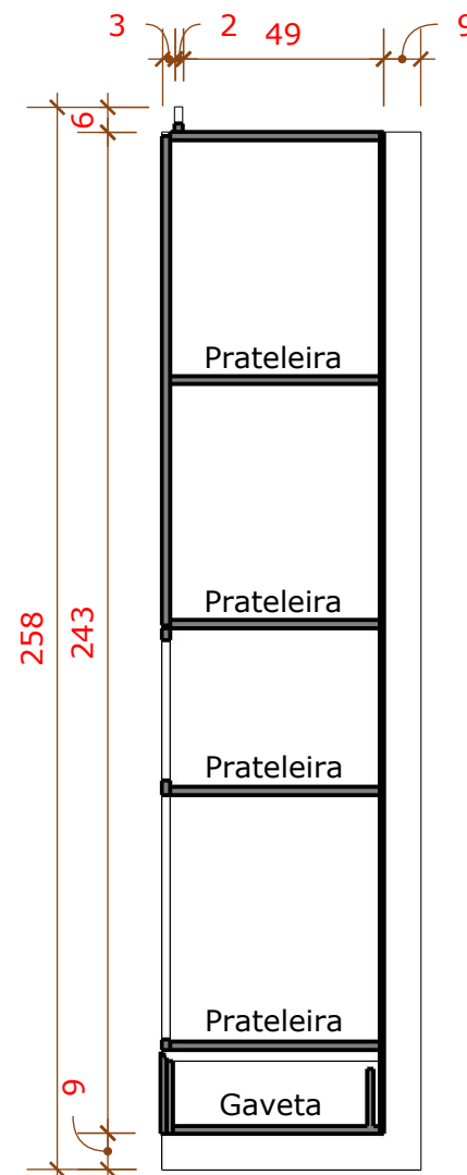
03 CORTE LATERAL TORRE 1/20
