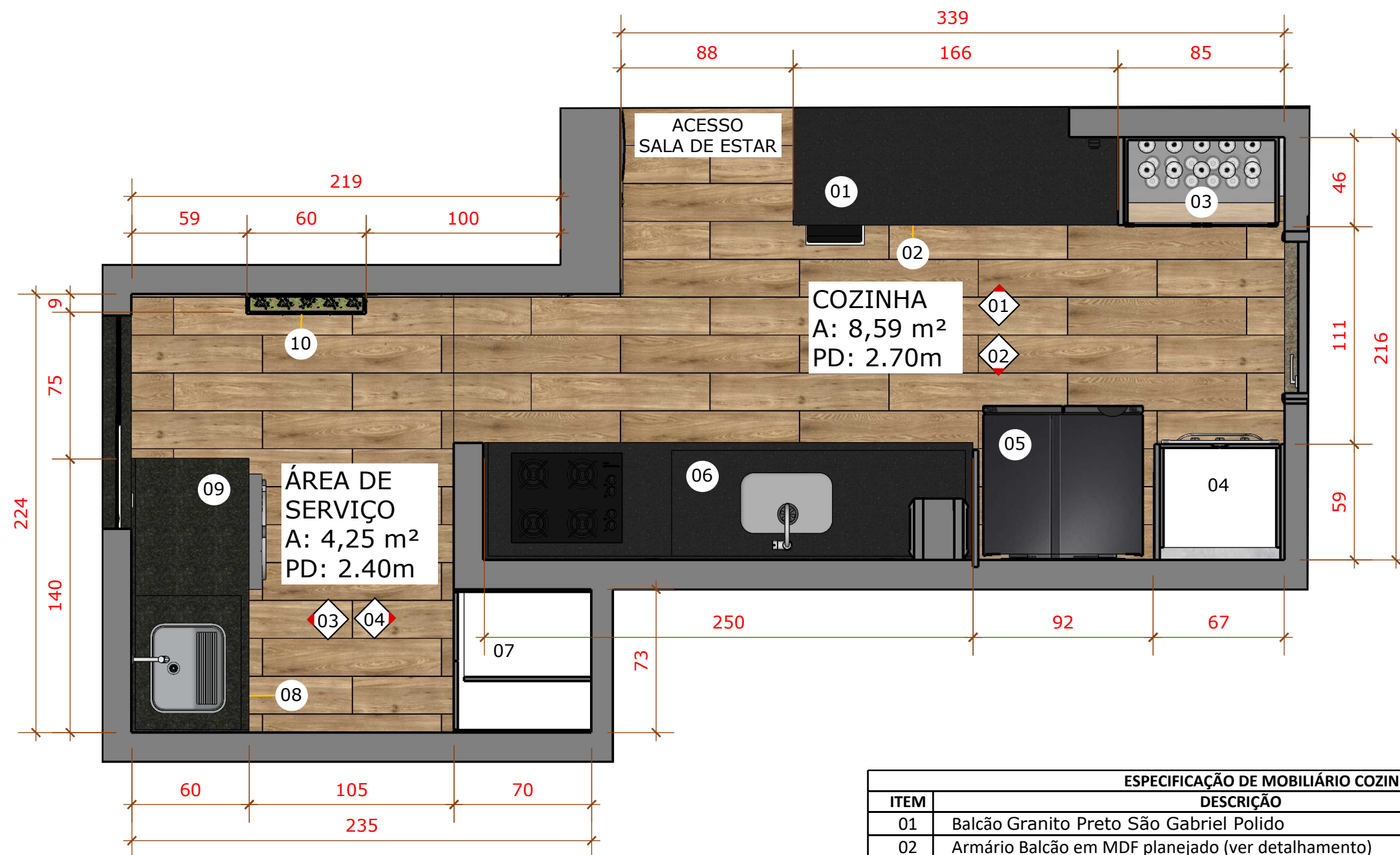
01 LAYOUT COZINHA E ÁREA DE SERVIÇO 1/25
