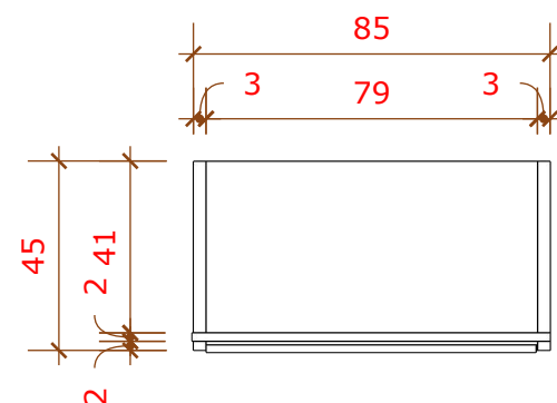
04 VISTA SUPERIOR CRISTALEIRA 1/20
