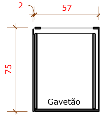
02 CORTE LATERAL GAVETÃO 1/20
