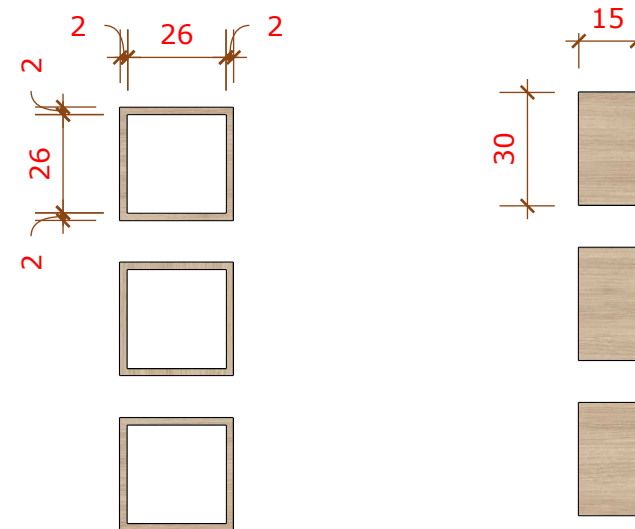
05 VISTA FRONTAL NICH 1/20
