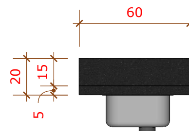
07 VISTA LATERAL BANCADA 1/20
