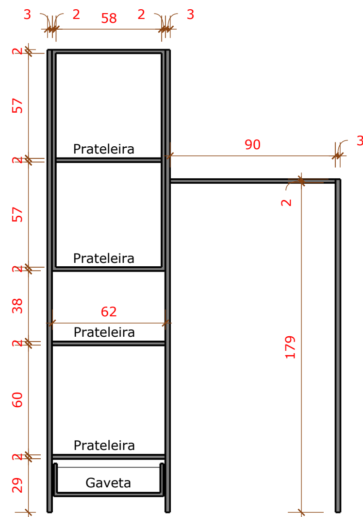
02 VISTA INTERNA TORRE 1/20
