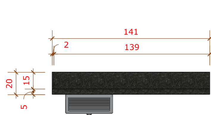
01 VISTA FRONTAL BANCADA 1/20
