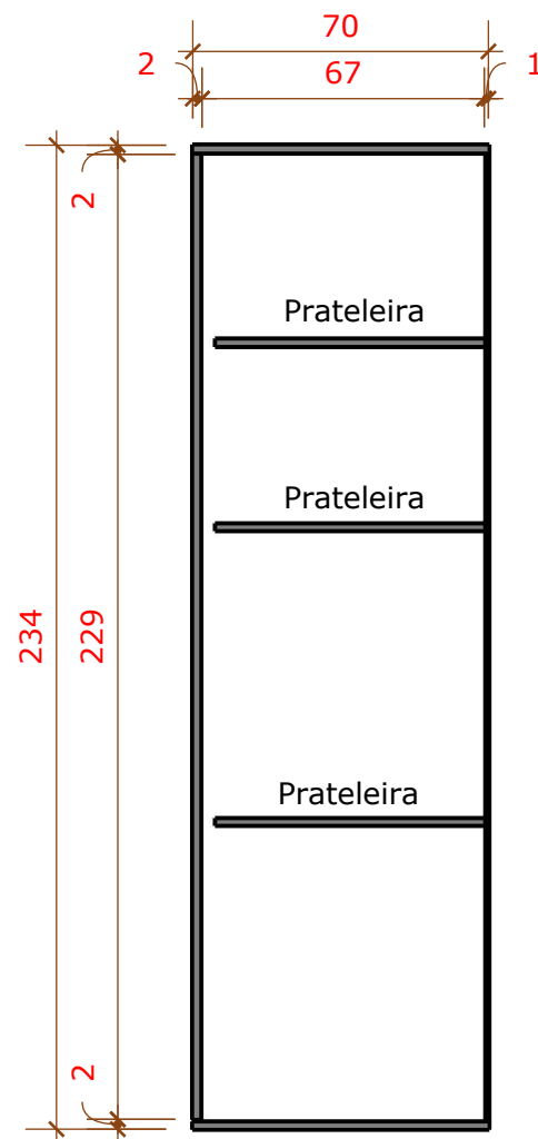
06 CORTE LATERAL ARM. MULTIUSO 1/20
