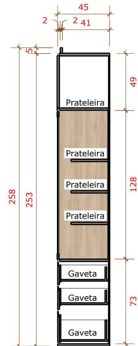
03 CORTE LATERAL CRISTALEIRA 1/20
