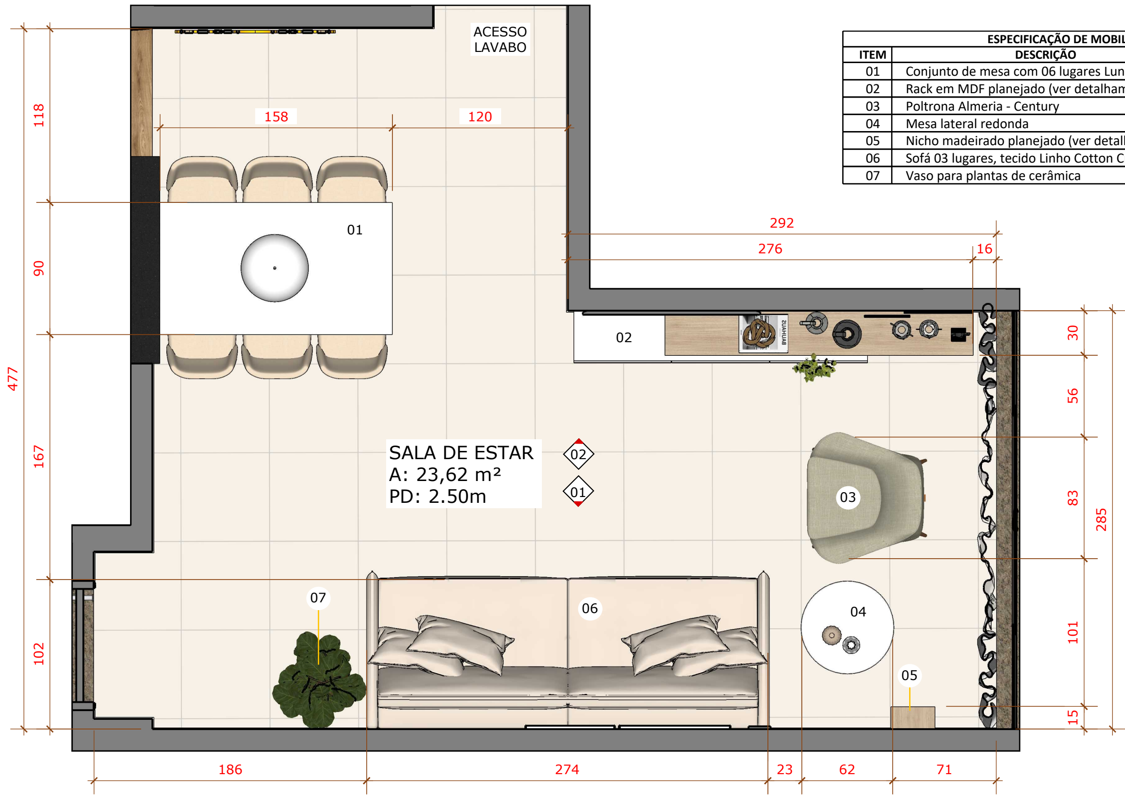
01 LAYOUT SALA DE ESTAR 1/25
