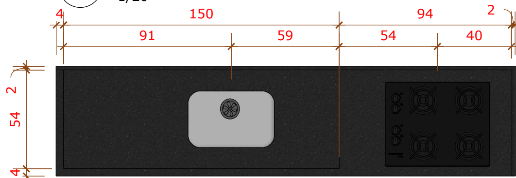
06 VISTA SUPERIOR BANCADA 1/20
