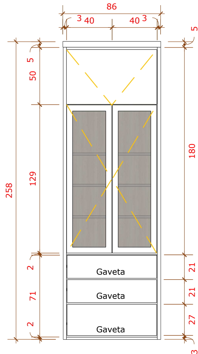
01 VISTA FRONTAL CRISTALEIRA 1/20
