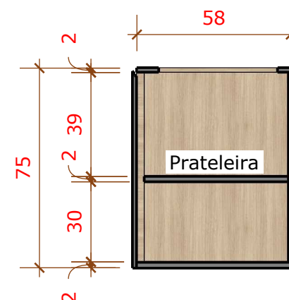
06 CORTE LATERAL ARM. BANCADA 1/20
