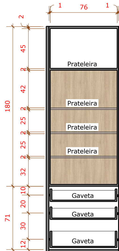
02 VISTA INTERNA CRISTALEIRA 1/20
