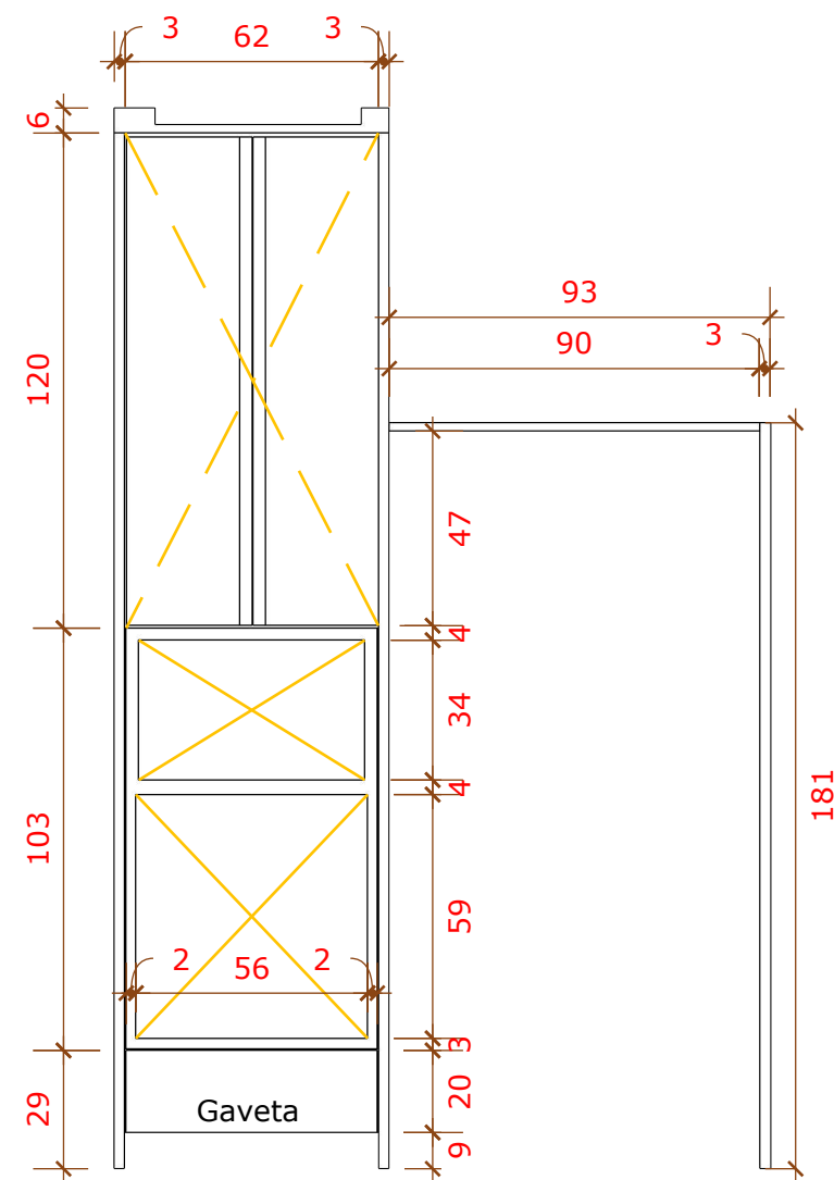
01 VISTA FRONTAL TORRE 1/20
