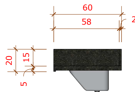
02 VISTA LATERAL BANCADA 1/20
