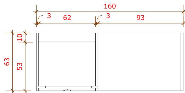
04 VISTA SUPERIOR TORRE 1/20
