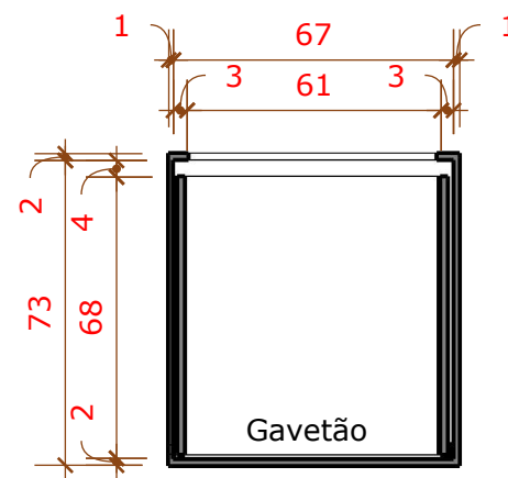
03 VISTA INTERNA GAVETÃO 1/20
