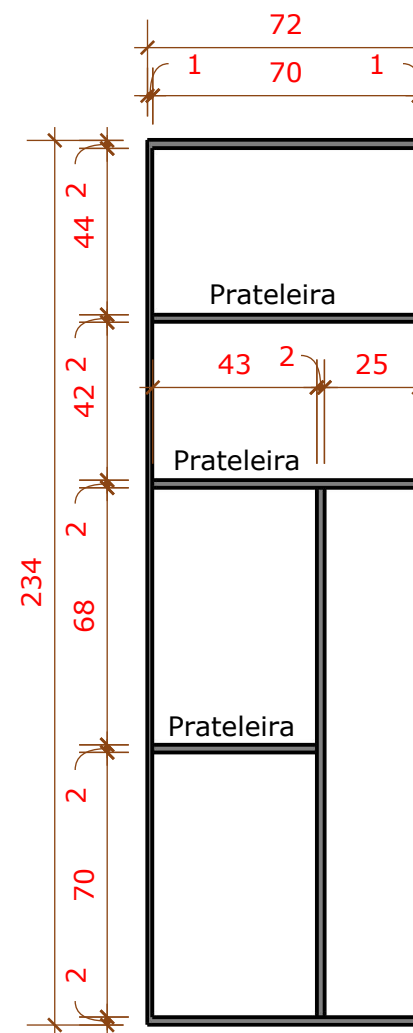
07 VISTA INTERNA ARM. MULTIUSO 1/20
