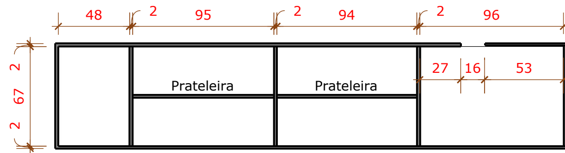
04 VISTA INTERNA ARM. SUP. 01 1/25
