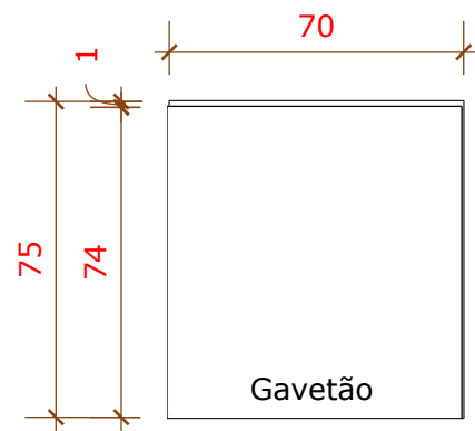
01 VISTA FRONTAL GAVETÃO 1/20
