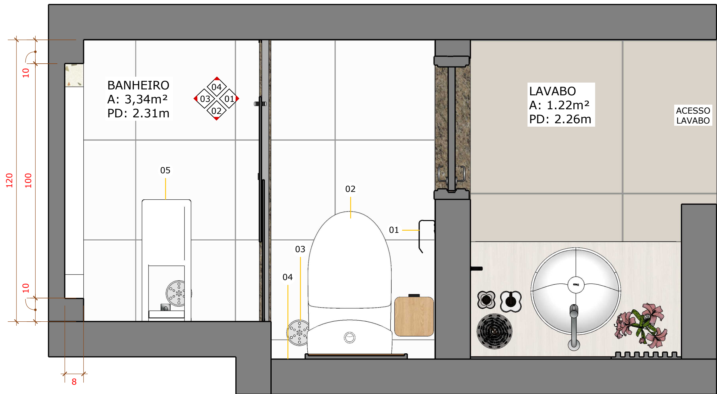
01 LAYOUT BANHEIRO 1/10
