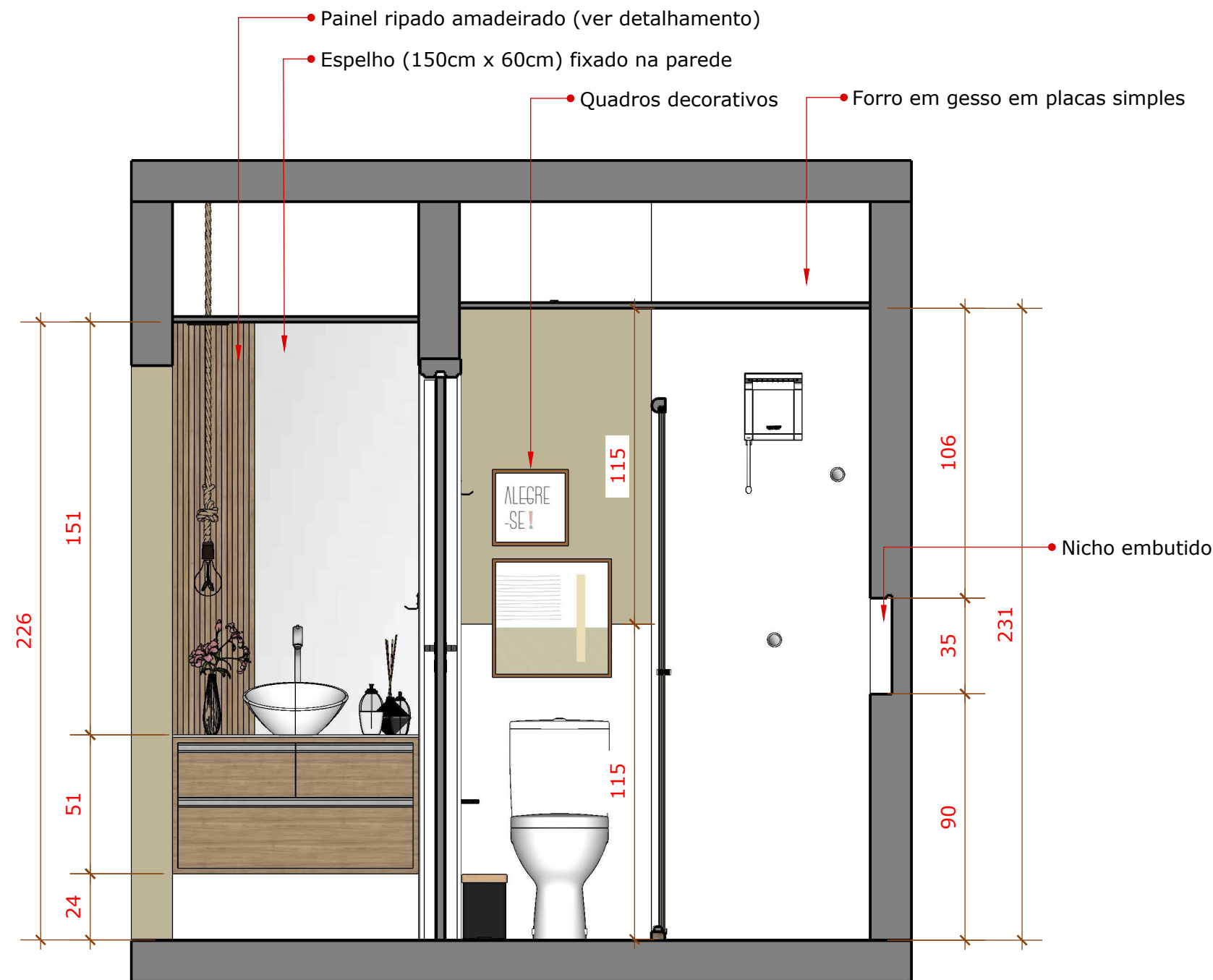
01 VISTA 01 1/20
