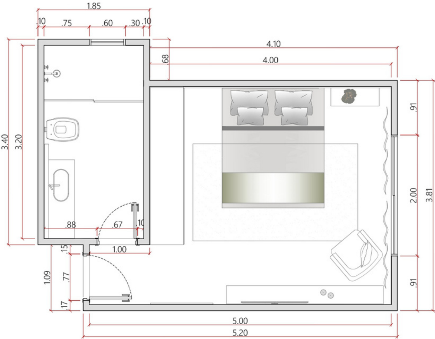
PLANTA LAYOUT SEM ESCALA
