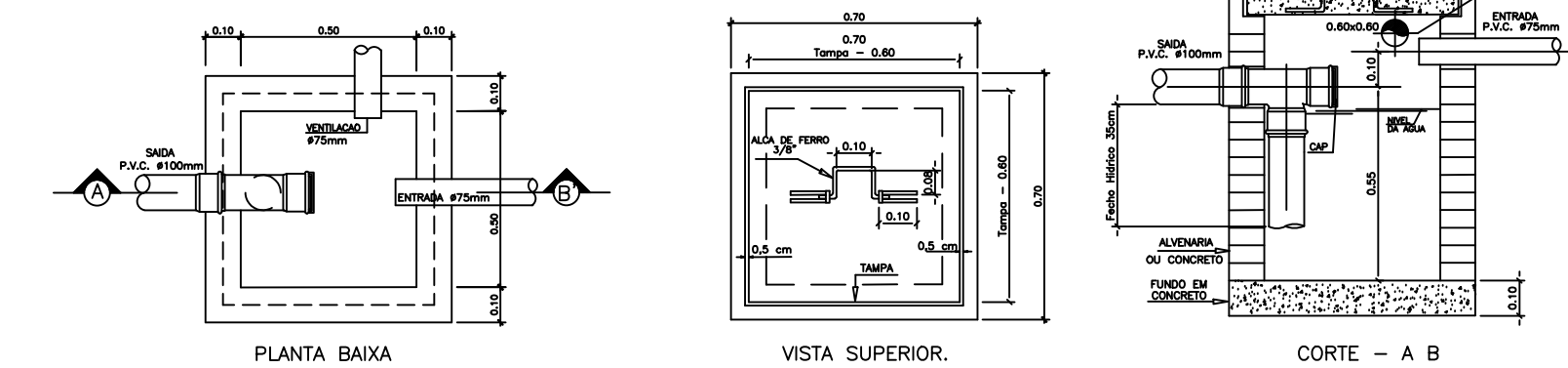
DETALHE EXECUTIVO DE ESGOTO CAIXA DE GORDURA (Capacidade 120 litros)
