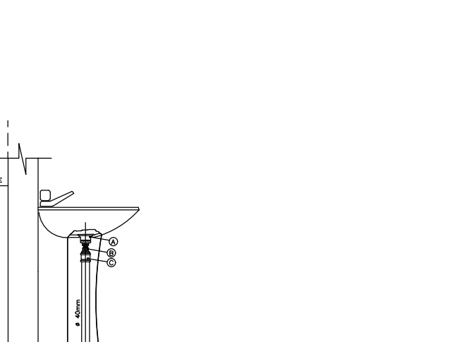
DETALHE EXECUTIVO HIDROSSANITÁRIO RAMAL DO LAVATÓRIO
