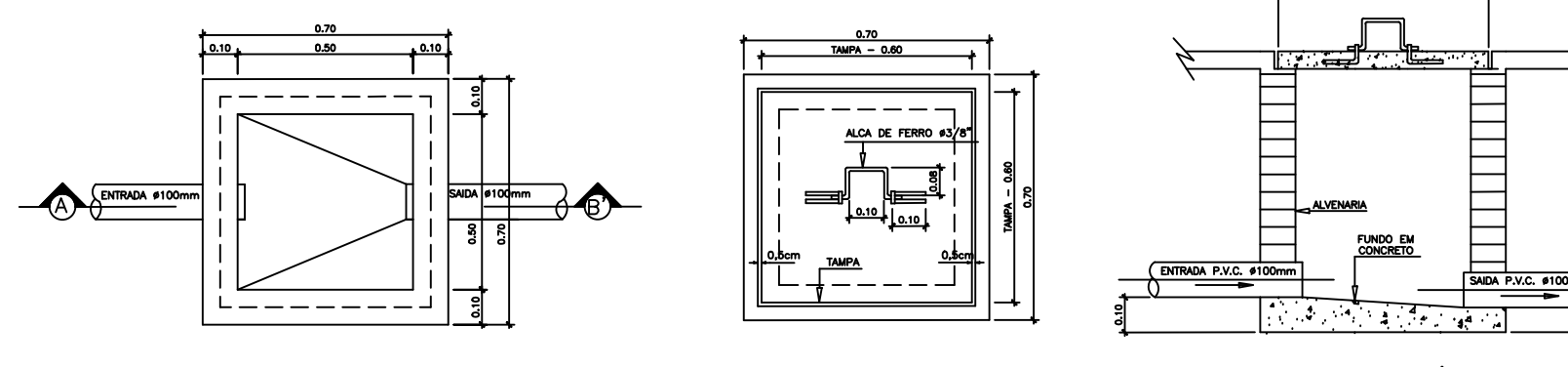
DETALHE EXECUTIVO DE ESGOTO CAIXA DE PASSAGEM 50x50 — TAMPA DE CONCRETO
