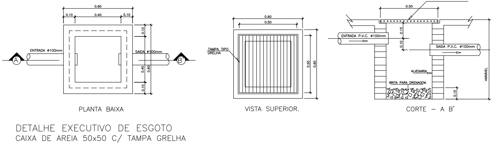
DETALHE EXECUTIVO DE ESGOTO CAIXA DE AREIA 50x50 C/ TAMPA GRELHA
