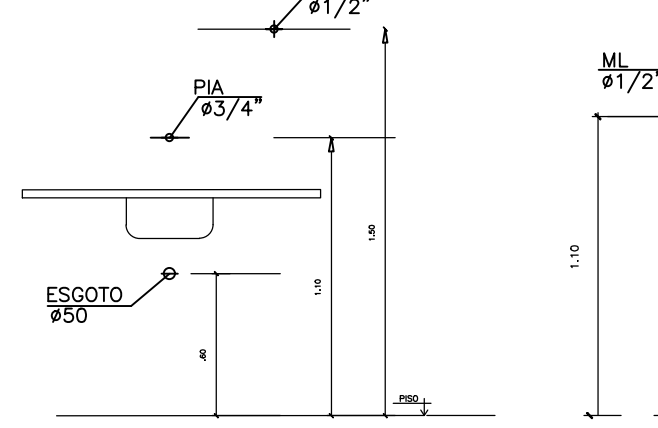
DETALHE EXECUTIVO SANITÁRIO RAMAL DA PIA/COZINHA COM SIFÃO
