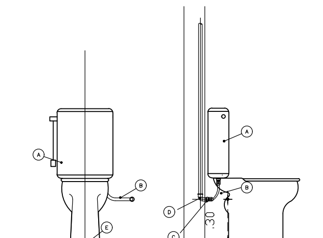
DETALHE EXECUTIVO HIDROSSANITÁRIO VASO SANITÁRIO C/ CAIXA DE ACOPLADA
