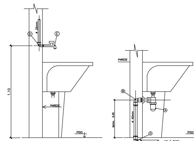
DETALHE EXECUTIVO HIDROSSANITÁRIO RAMAL DA PIA/COZINHA (c/ misturador)
