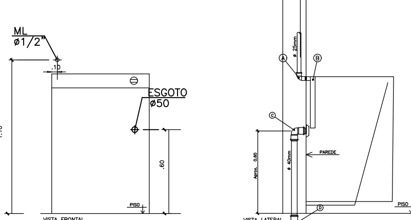
DETALHE EXECUTIVO HIDROSSANITÁRIO RAMAL DA MÁQUINA DE LAVAR
