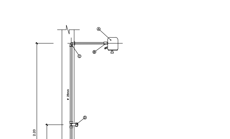
DETALHE EXECUTIVO HIDROSSANITÁRIO RAMAL DO CHUVEIRO
