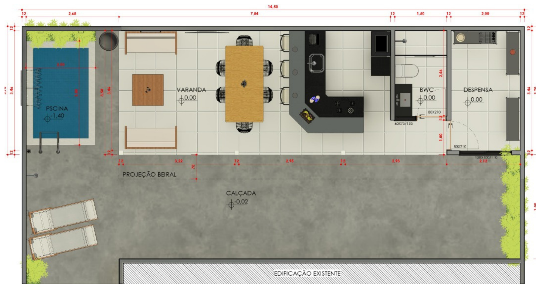
Planta Baixa
