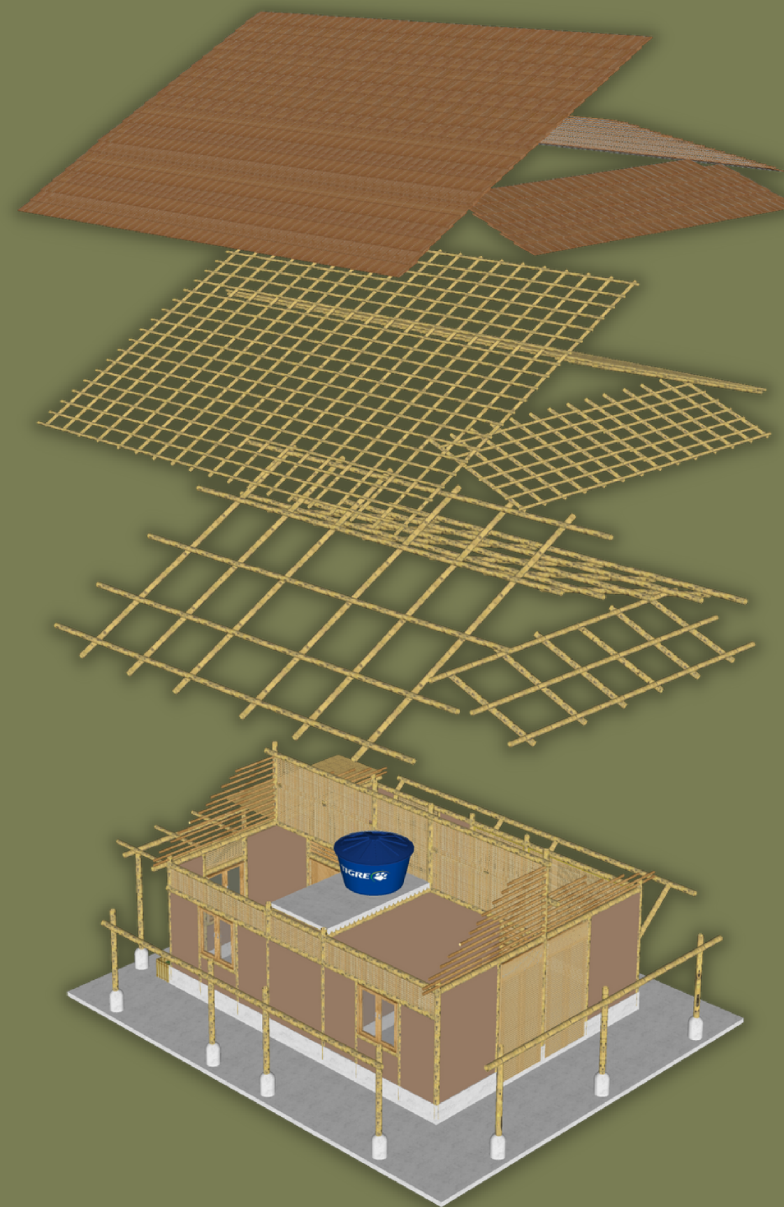
MODELAGEM EXPLODIDA
