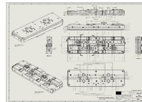
Proj. Micrométrico Matriz P1 – Desenho Técnico
