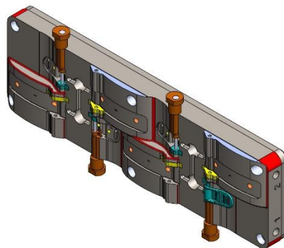
Proj. Micrométrico Matriz P2
