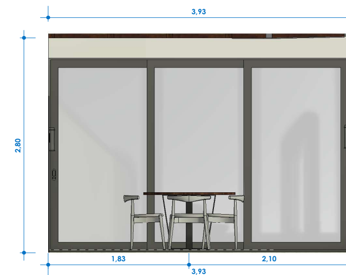
VISTA C ESCALA 1:75
