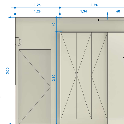
VISTA B ESCALA 1:50
