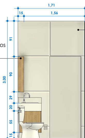
VISTA C ESCALA 1:50
