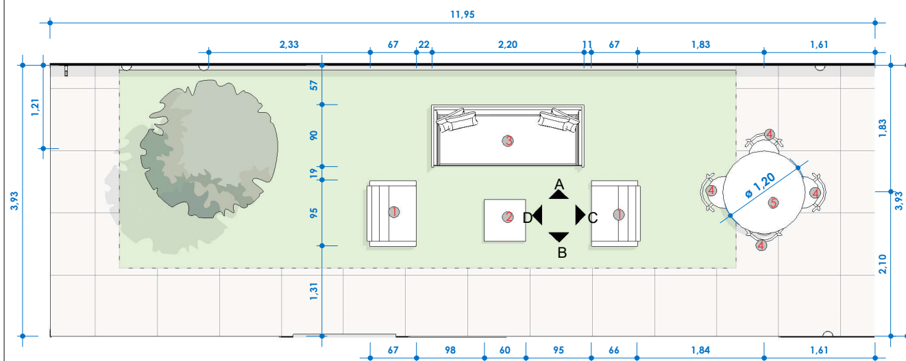
LAYOUT ESCALA 1:50
