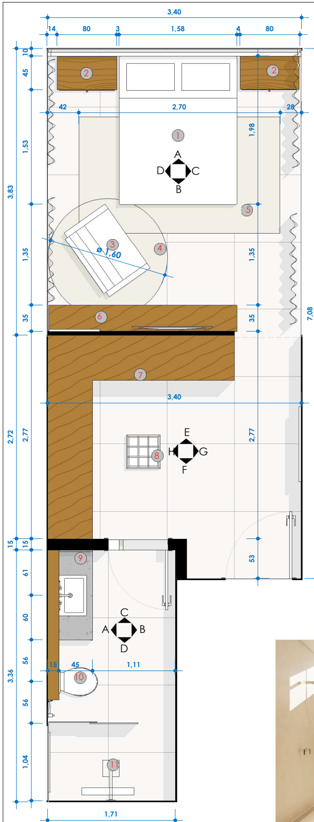
LAYOUT ESCALA 1:50
