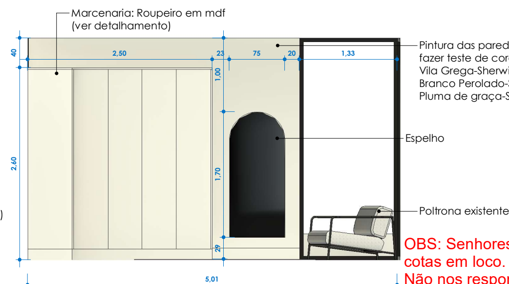
VISTA B ESCALA 1:50
