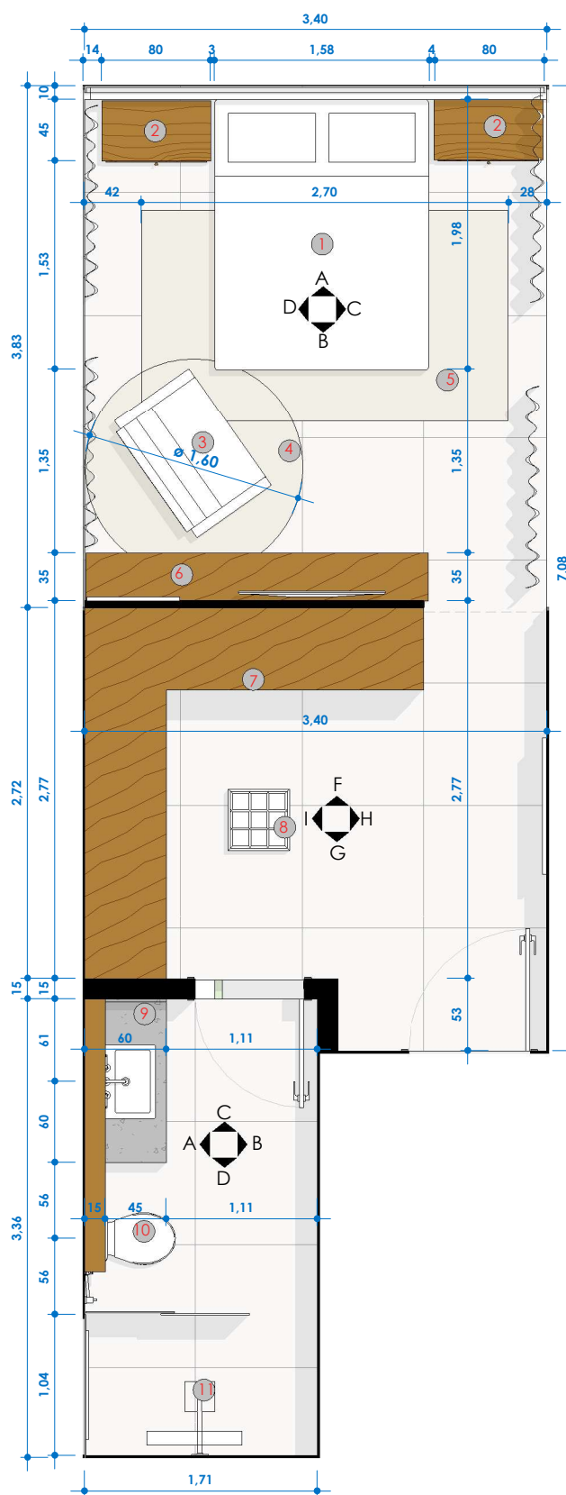
LAYOUT ESCALA 1:50
