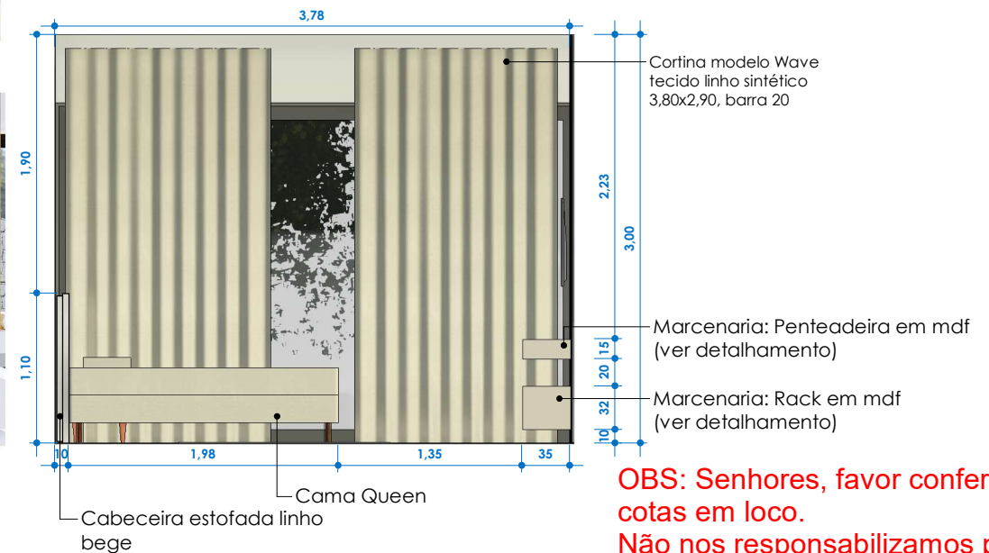
VISTA C ESCALA 1:50
