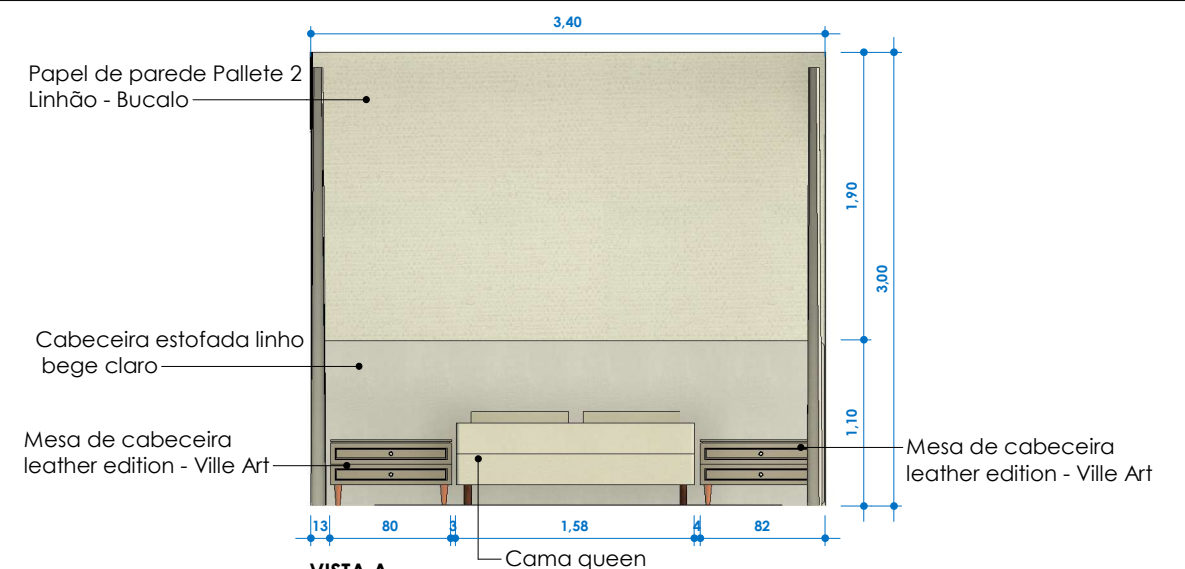
VISTA A ESCALA 1:50
