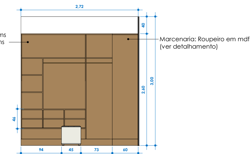
VISTA H ESCALA 1:50
