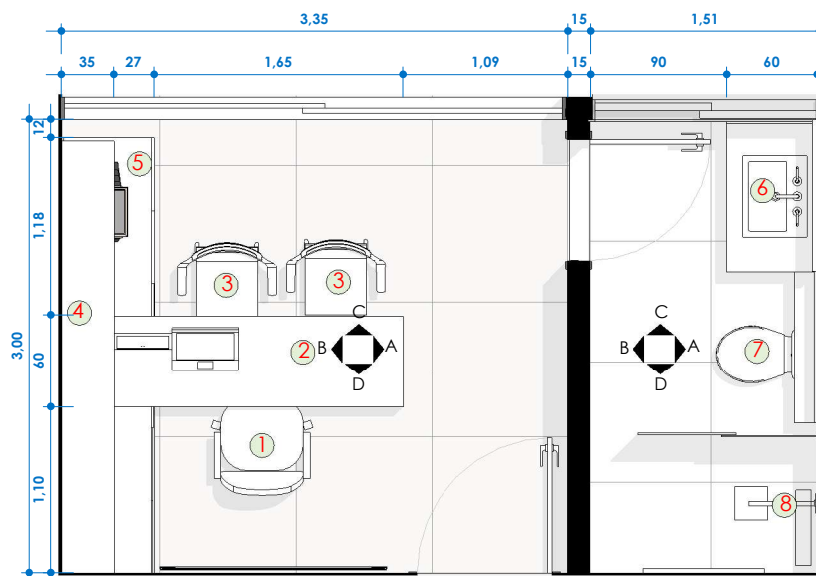
LAYOUT ESCALA 1:50
