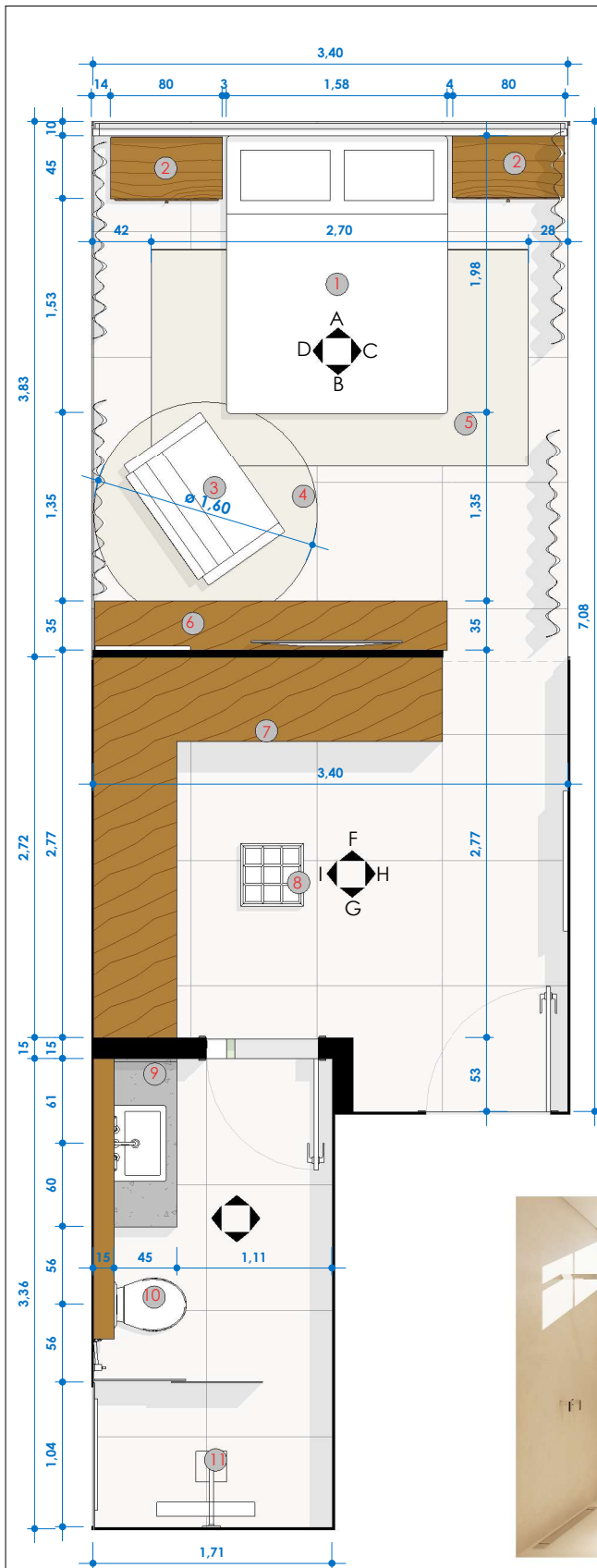
LAYOUT ESCALA 1:50
