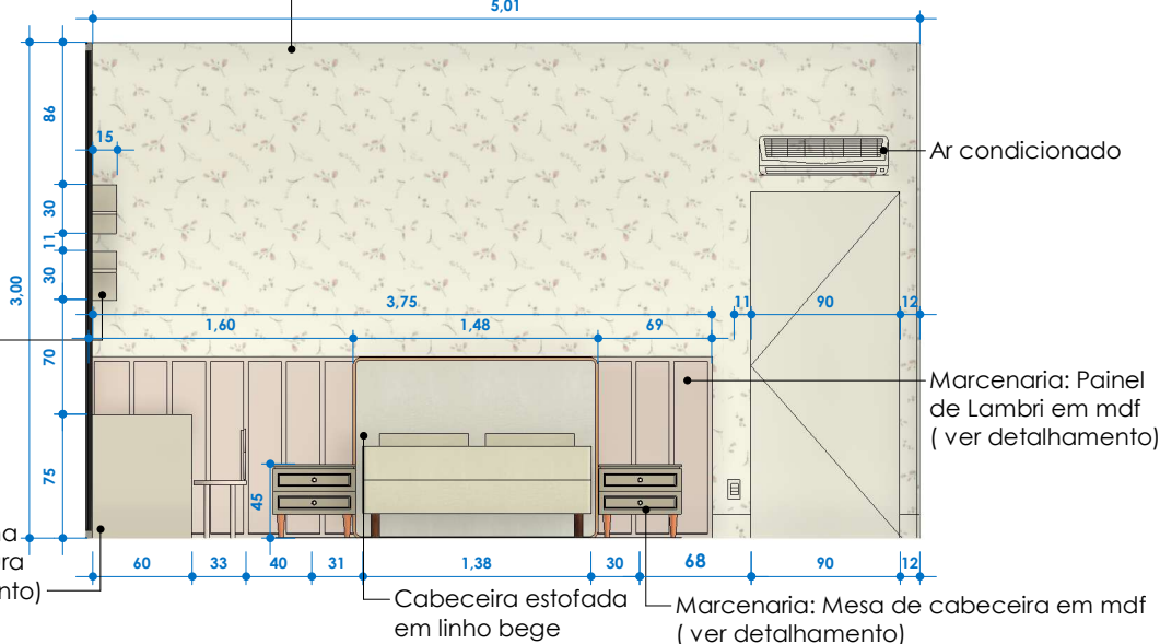
VISTA A ESCALA 1:50
