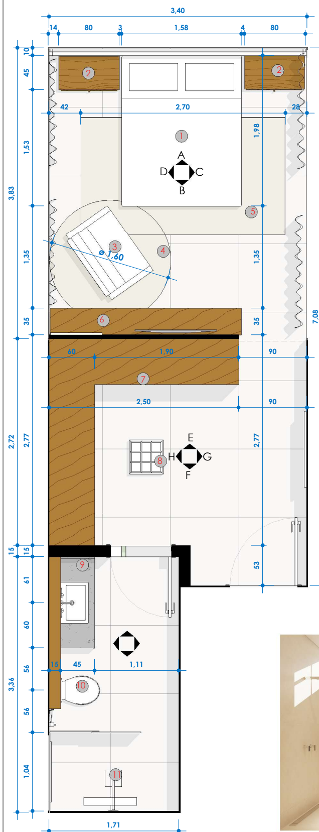
LAYOUT ESCALA 1:50
