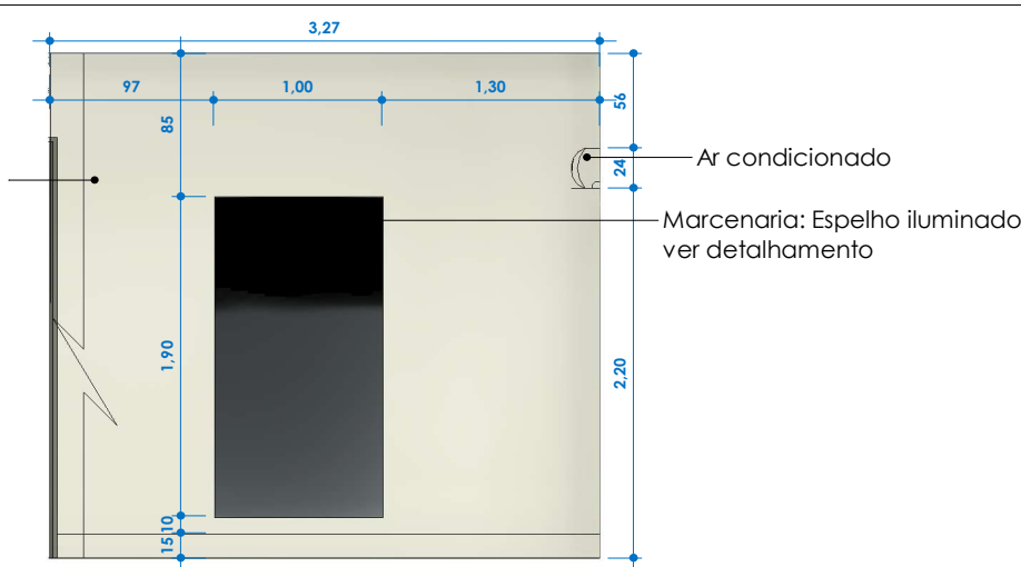
VISTA G ESCALA 1:50
