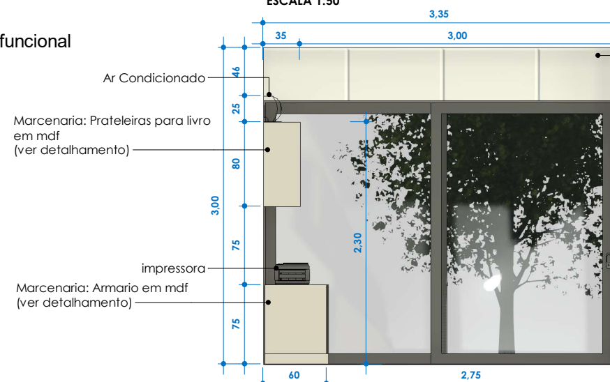
VISTA C ESCALA 1:50
