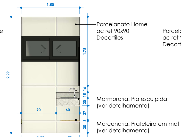
VISTA C ESCALA 1:50
