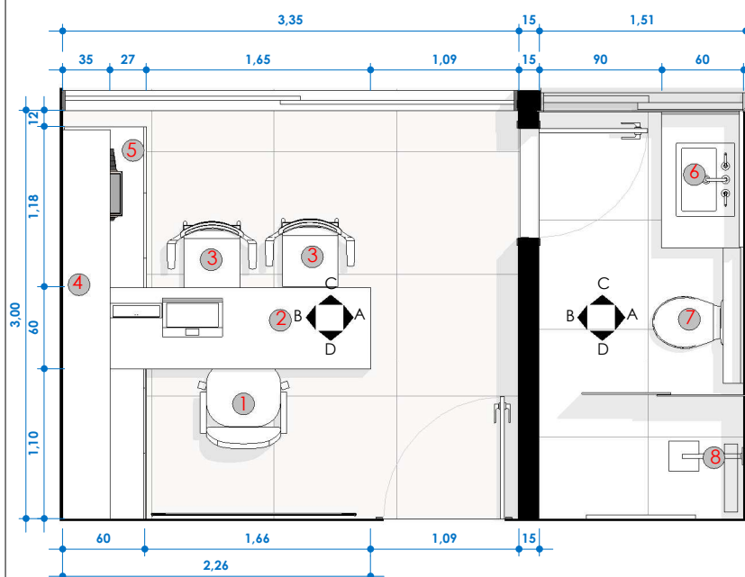
LAYOUT ESCALA 1:50
