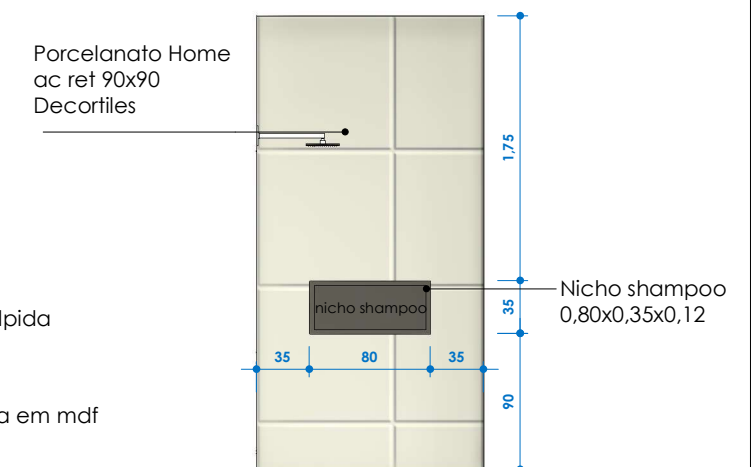
VISTA D ESCALA 1:50
