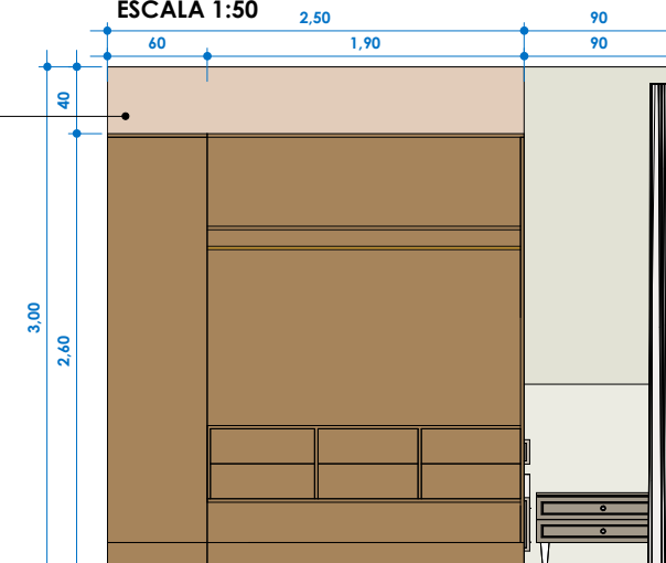
VISTA E ESCALA 1:50
