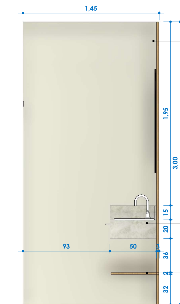
VISTA C ESCALA 1:25
