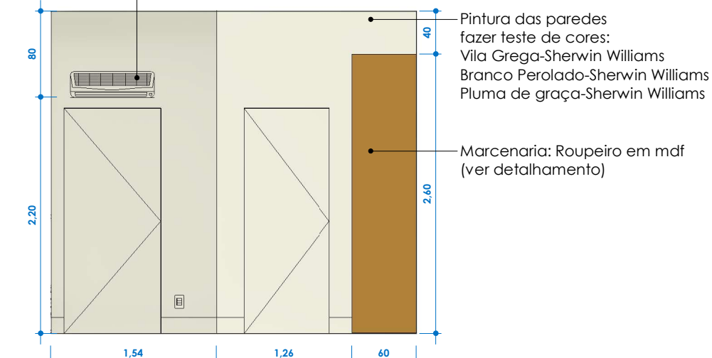
VISTA F ESCALA 1:50
