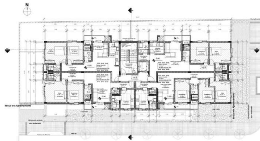
Planta baixa por Lucas Salin
