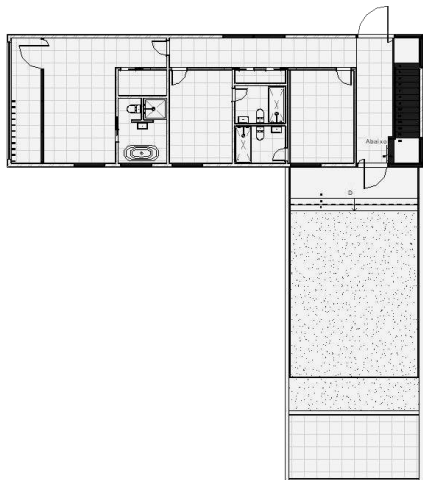
Planta baixa por Lucas Salin
