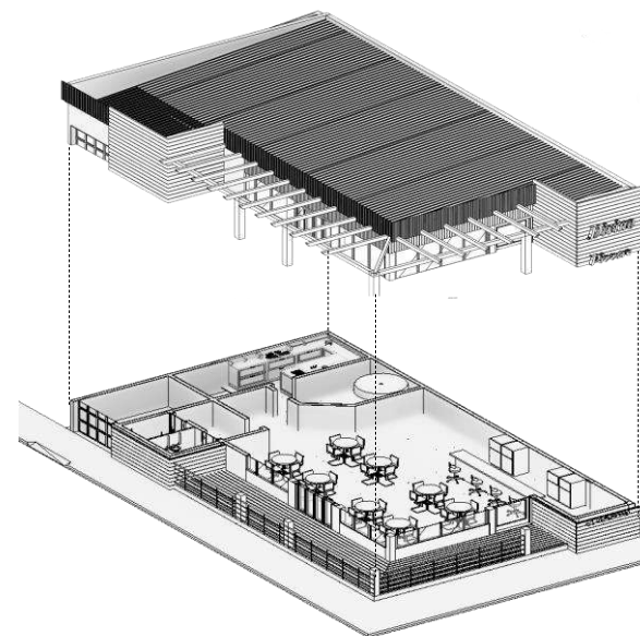
Perspectiva explodida por Lucas Salin
