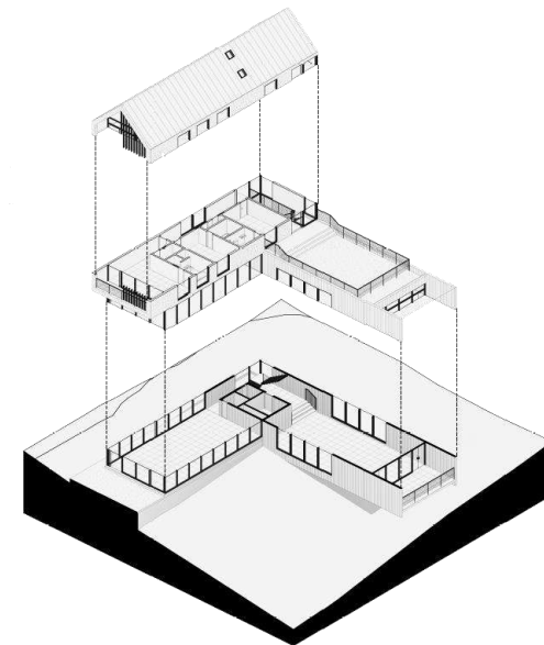
Perspectiva explodida por Lucas Salin
