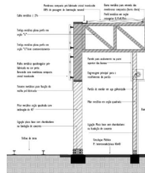
Corte/detalhamento por Lucas Salin
