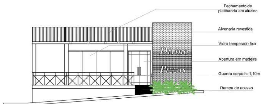
Fachada Norte por Lucas Salin
