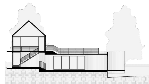
Corte por Lucas Salin
