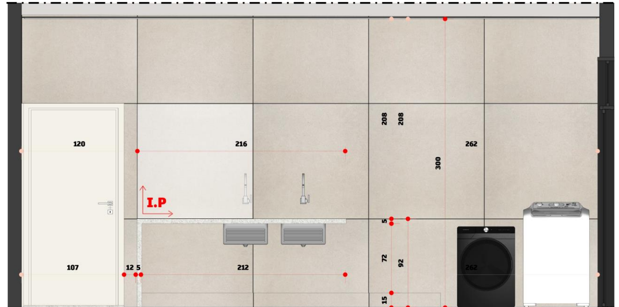
VISTA 04 | LAVANDERIA Esc 1/25
