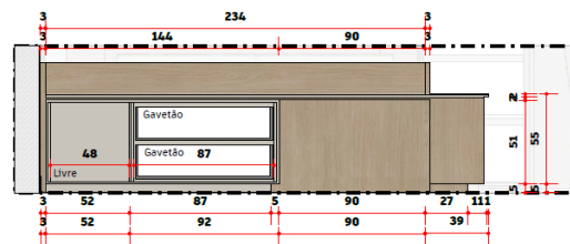
Vista 02 | Aparador/Bufet (interno) Esc 1/20
