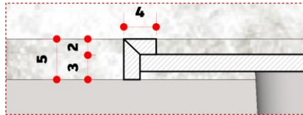
Det. 02 | área molhada Esc 1/5
