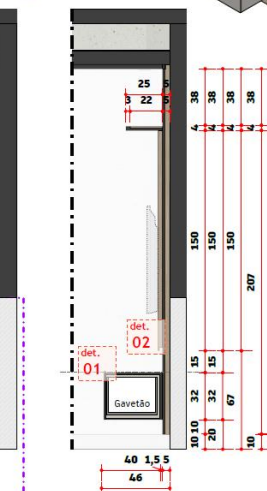
Corte 01 Esc 1/20
