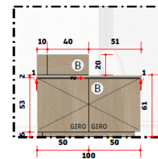
Vista 03 (externo) Esc 1/20
