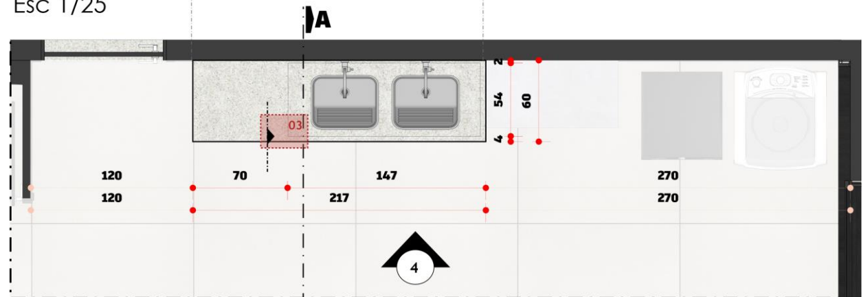
PLANTA | LAVANDERIA Esc 1/25
