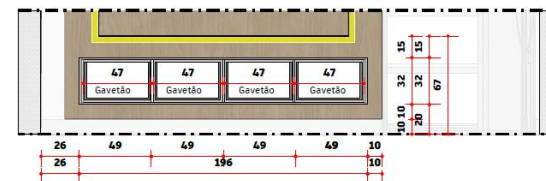
Vista 01 | rack + painel TV (interno) Esc 1/20
