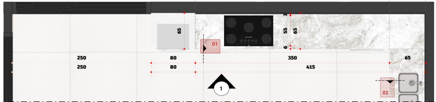
PLANTA | BANCADA COZINHA Esc 1/25
