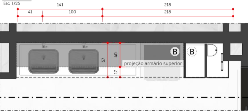
PLANTA COZINHA
