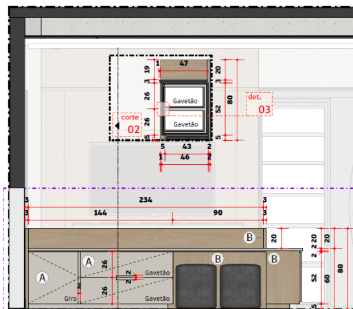
Vista 02 | Aparador/Bufet (externo) Esc 1/20
