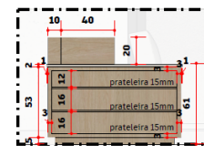
Vista 03 (interno) Esc 1/20
