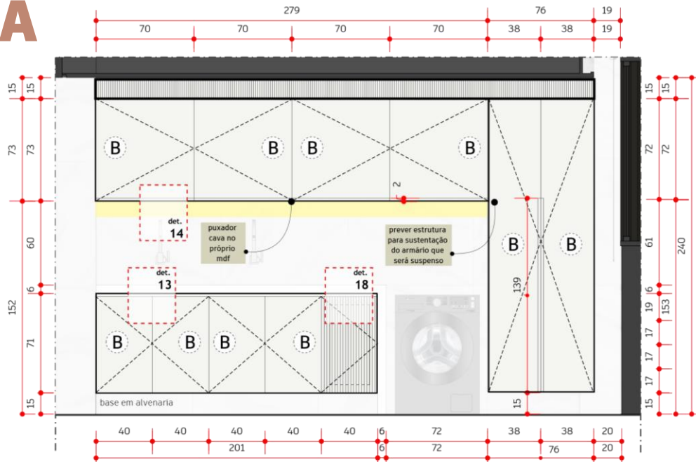
CORTE KK
