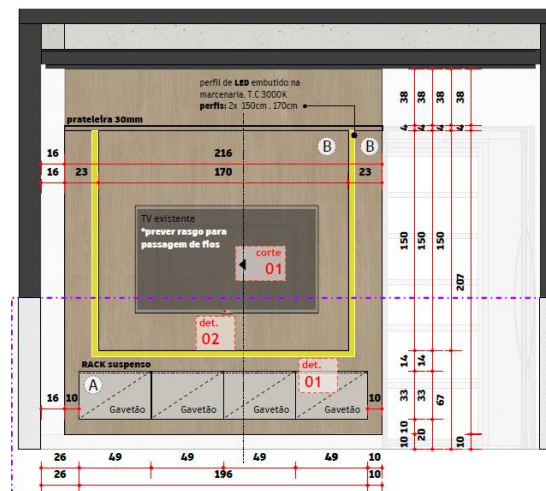
Vista 01 | rack + painel TV (externo) Esc 1/20
