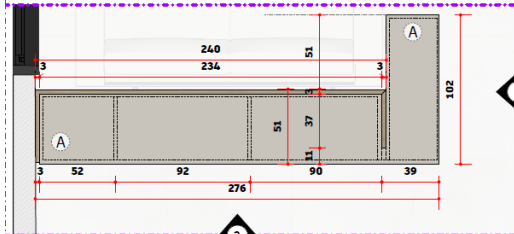
PLANTA | Aparador/Bufet Esc 1/20
