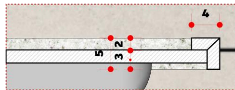
Det. 03 | área molhada Esc 1/5
