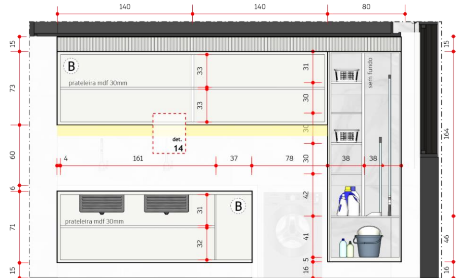
CORTE KK | SEM PORTAS
