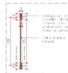
PORTA DO GAVETEIRO DE ROUPA SUJA DET 1
