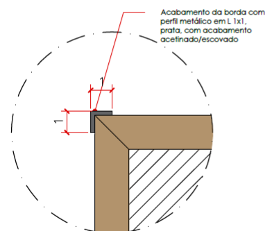
DET003 Acabamento borda degrau
