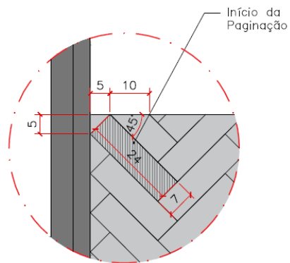
DET001 Início da paginação
