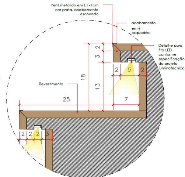
DET002 Degraus
