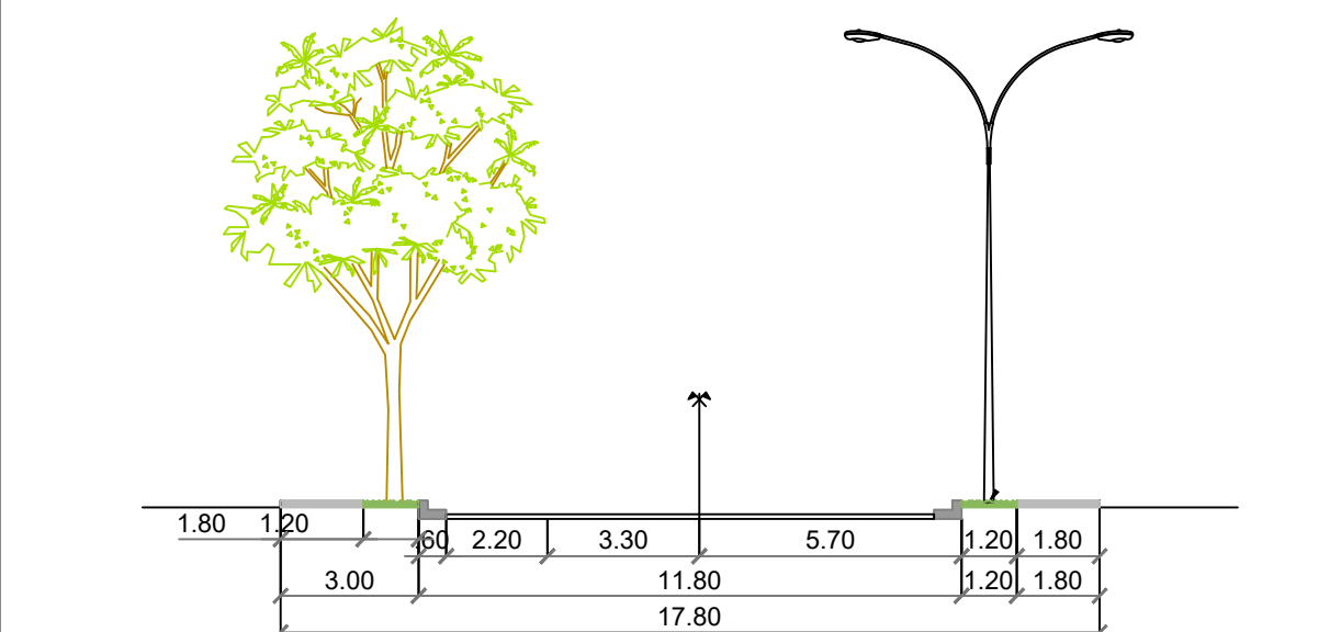
3 PERFIL DA VIA DE PASSAGEM SEM ESCALA
