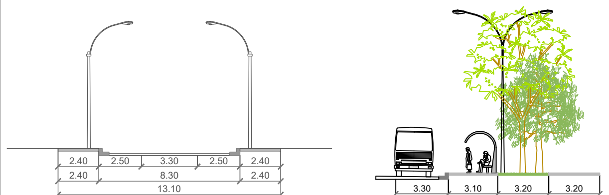
1 PERFIL DA VIA LOCAL SEM ESCALA
