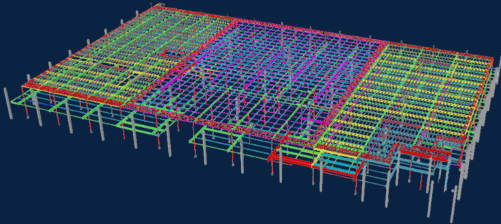
Mezanino Brainfarma (800 toneladas) Etapa - Modelagem e Detalhamento Cliente - EMTEC
