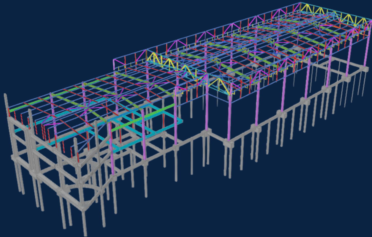
Galpão Industrial - Metalcoat Etapa - Modelagem e Detalhamento Cliente - Staux
