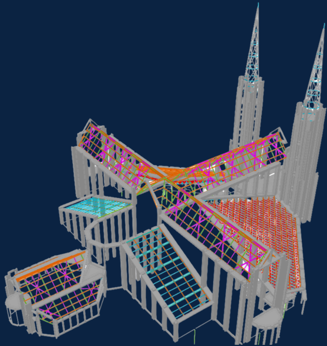
Igreja Católica - Estrutura Espacial Etapa - Cálculo / Modelagem / Detalhamento Cliente - DFS Engenharia
