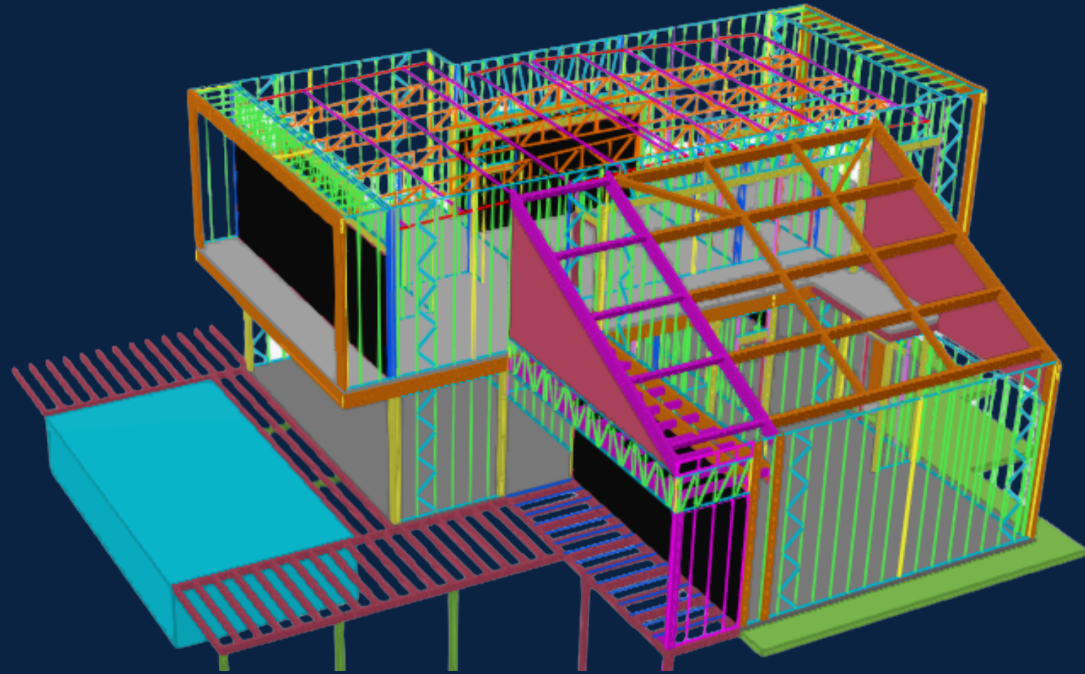
Residência - Steel Frame Etapa - Modelagem e Detalhamento Cliente - Alfred Dutzmann
