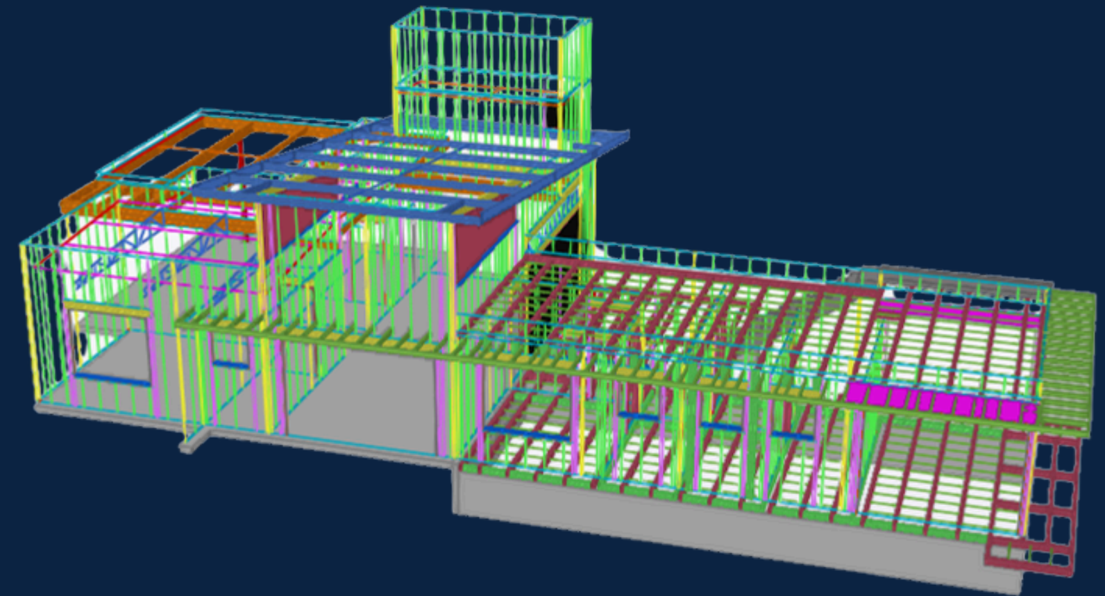
Residência - Steel Frame Etapa - Modelagem e Detalhamento Cliente - Alfred Dutzmann
