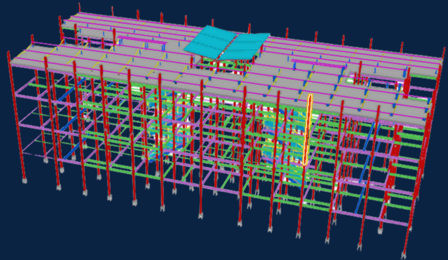
Prédio CDHU (90 Toneladas) Etapa - Cálculo / Modelagem / Detalhamento Cliente - SteelCORP.
