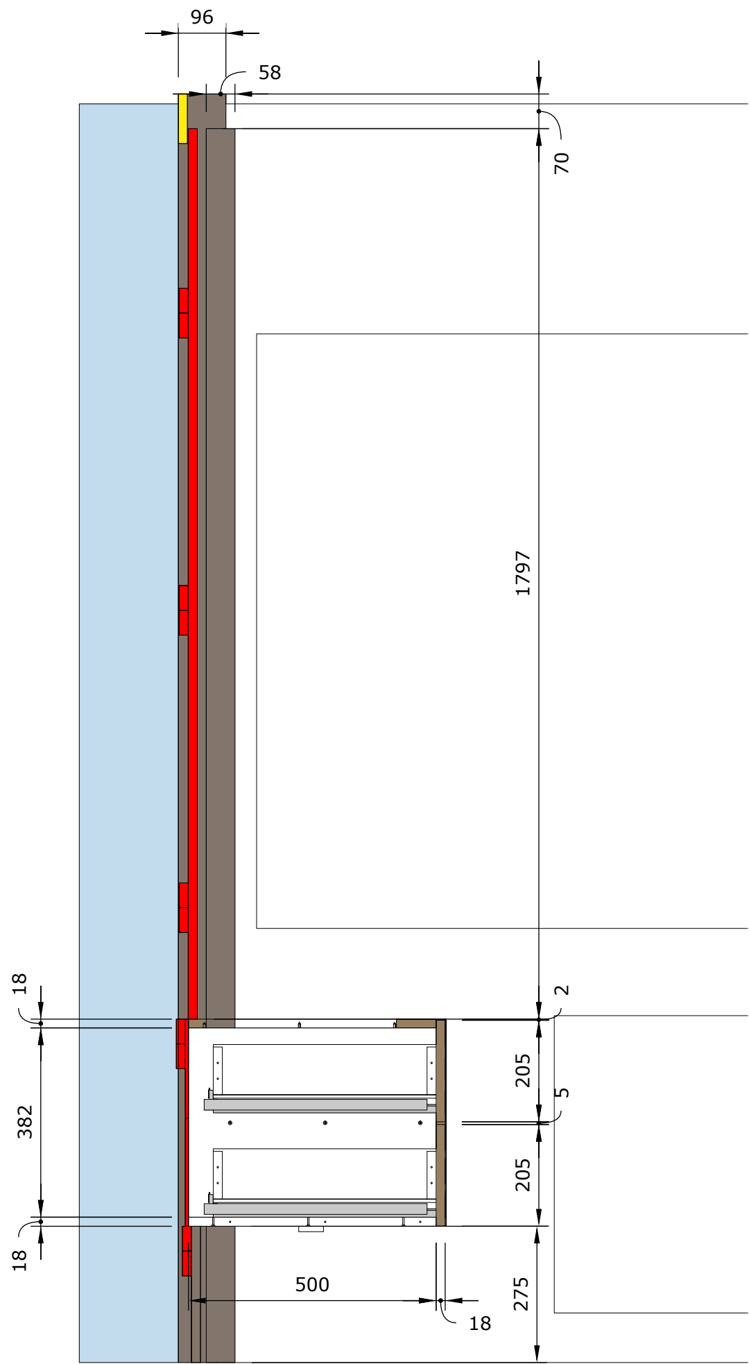
Corte Lateral 2
