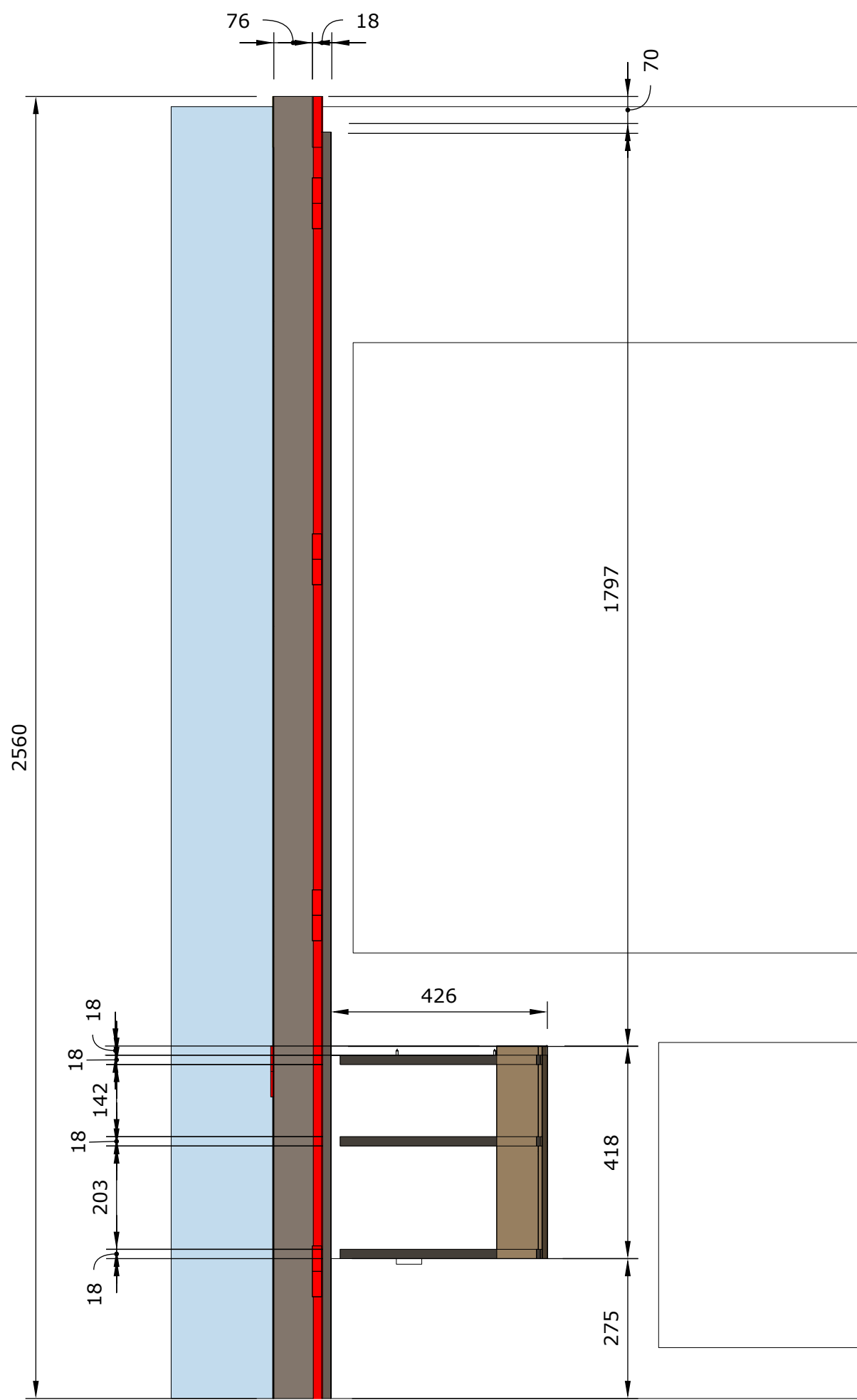
Corte Lateral 1
