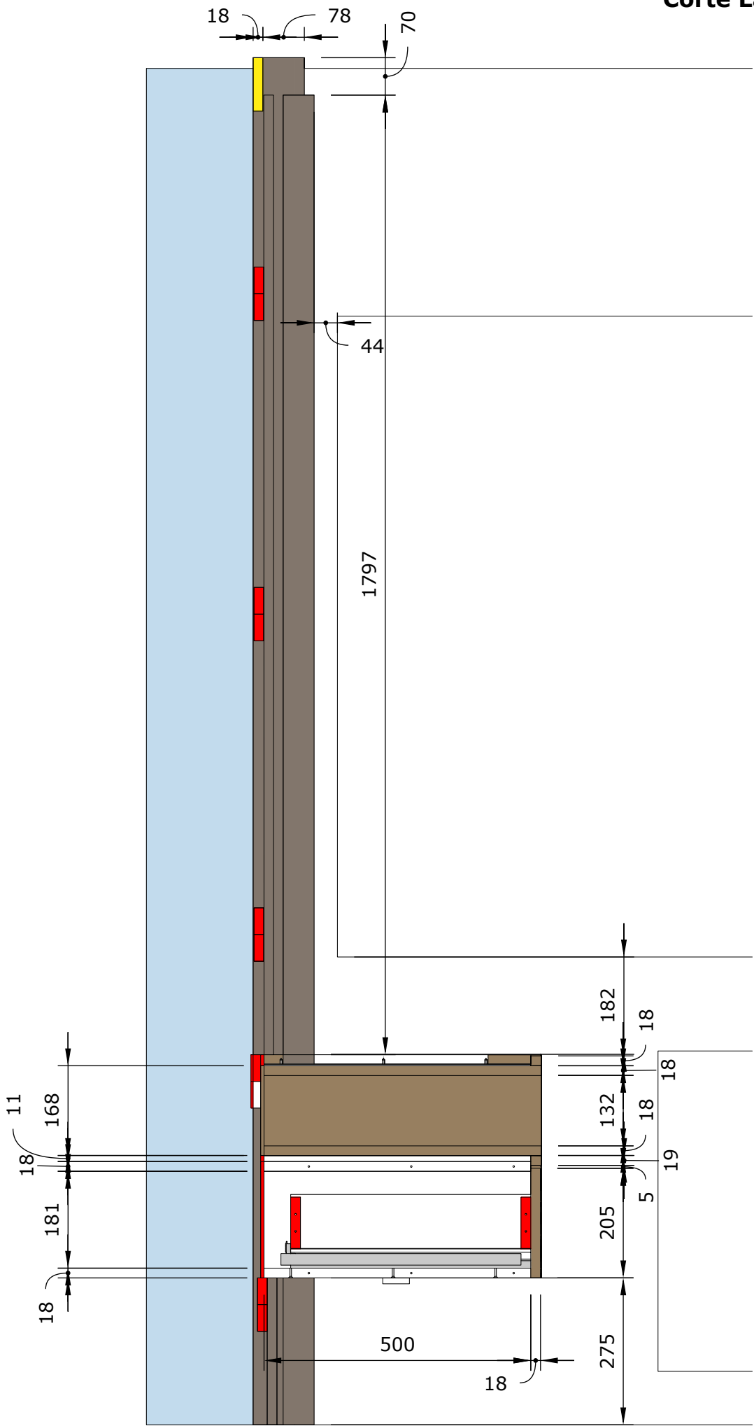
Corte Lateral 3
