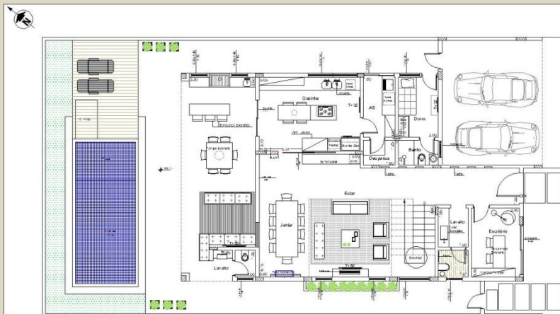
PLANTA PAV. TÉRREO
