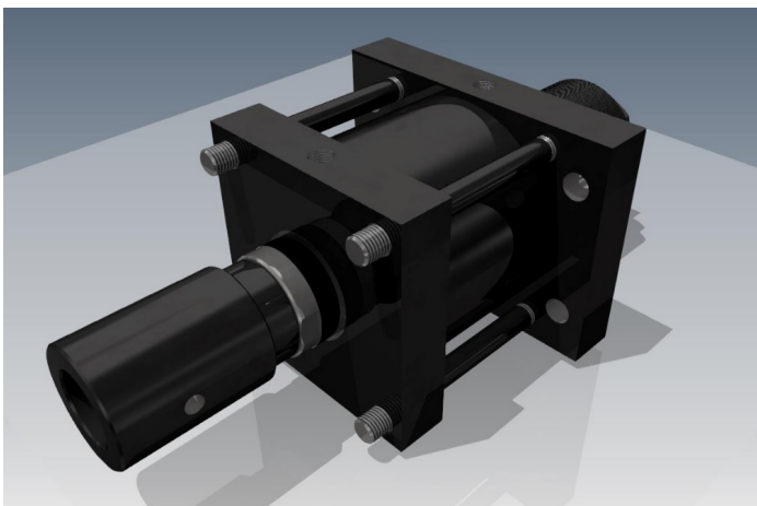
CILINDRO HIDRÁULICO ESTICADOR DE ESTEIRA
