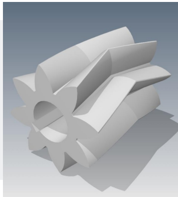
ENGRENAGEM BI-HELICOIDAL
