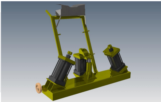
DISPOSITIVO DE FECHAMENTO DE VAGÕES
