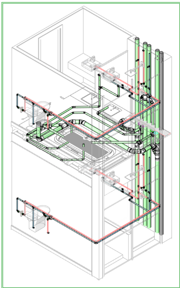
Perspectiva da instalação - Banheiro
