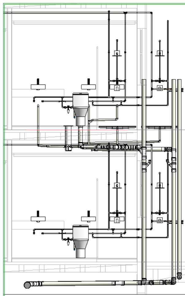
Corte Banheiro
