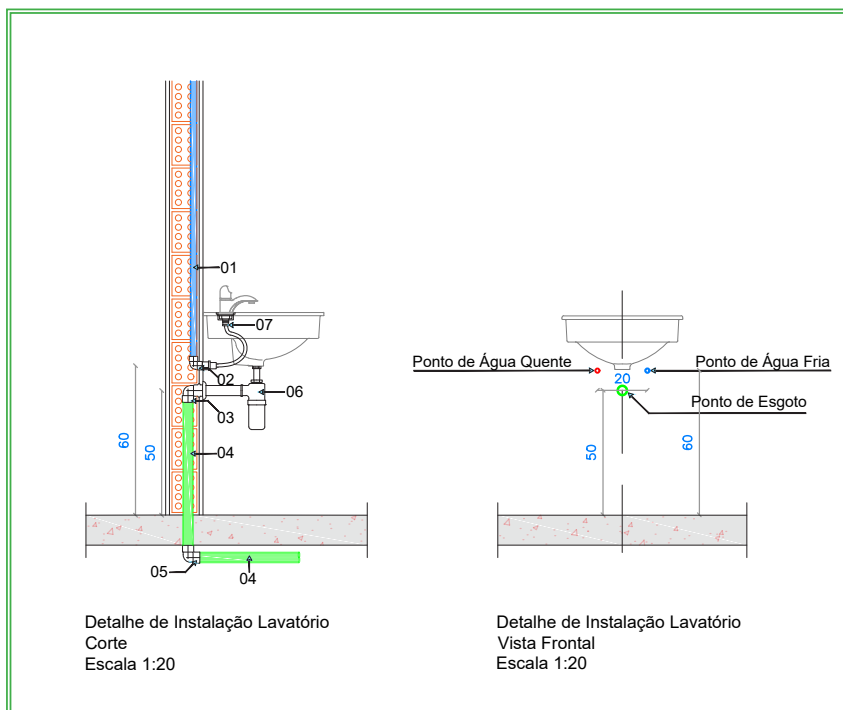
Detalhe Instalação Lavatório
