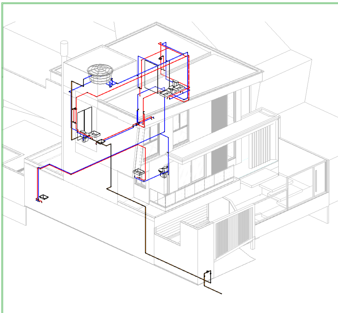
Perspectiva Hidráulica
