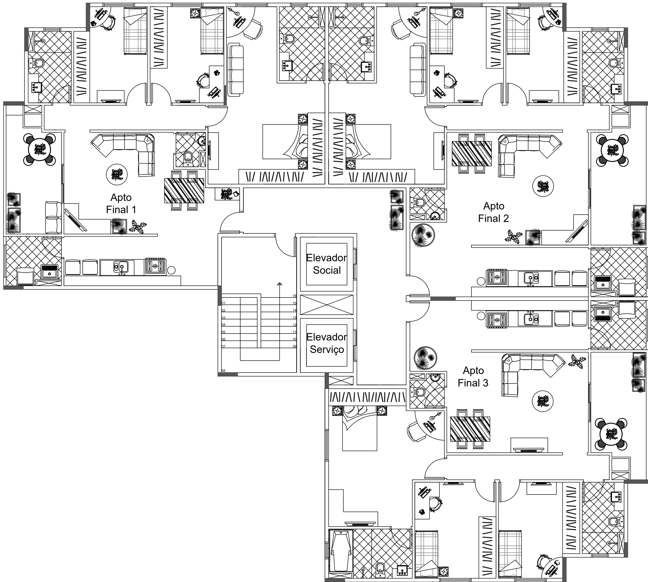
Escala 1:75 1º AO 5º ANDAR
